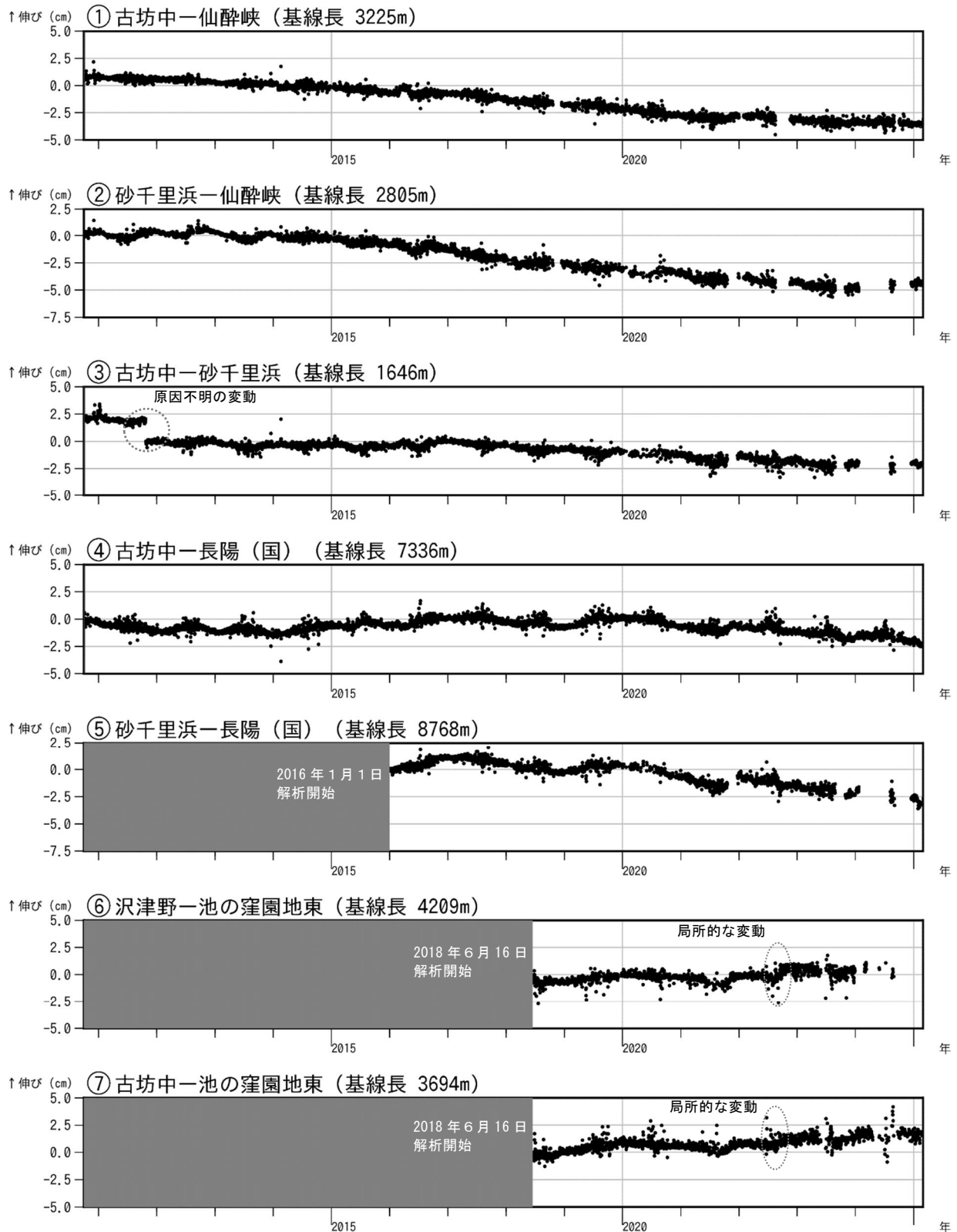
図 5 阿蘇山 GNSS 連続観測による基線長変化（2010 年 10 月～2025 年 2 月）
