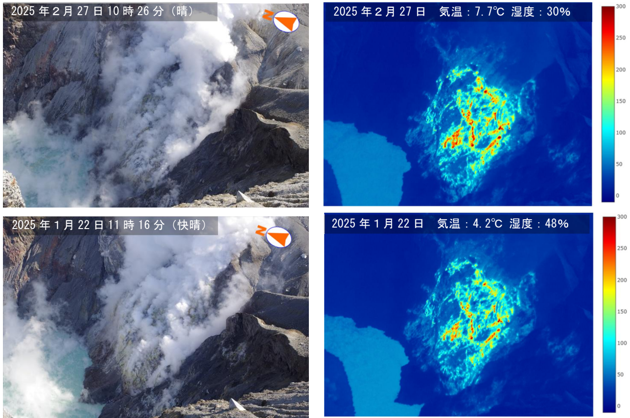
図 2-2 阿蘇山 中岳第一火口 南側火口壁の状況 (火口南西側観測定点から撮影 上図：2月27日、下図：1月22日)
