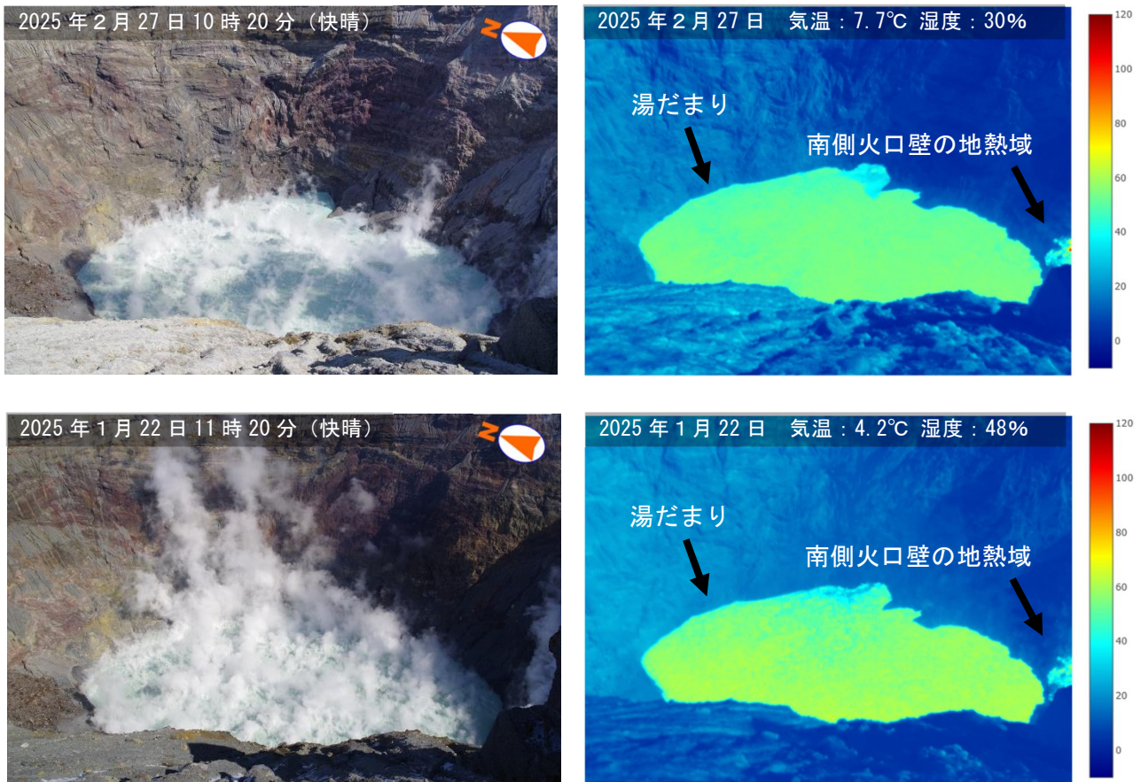
図 2-1 阿蘇山 中岳第一火口底の状況
