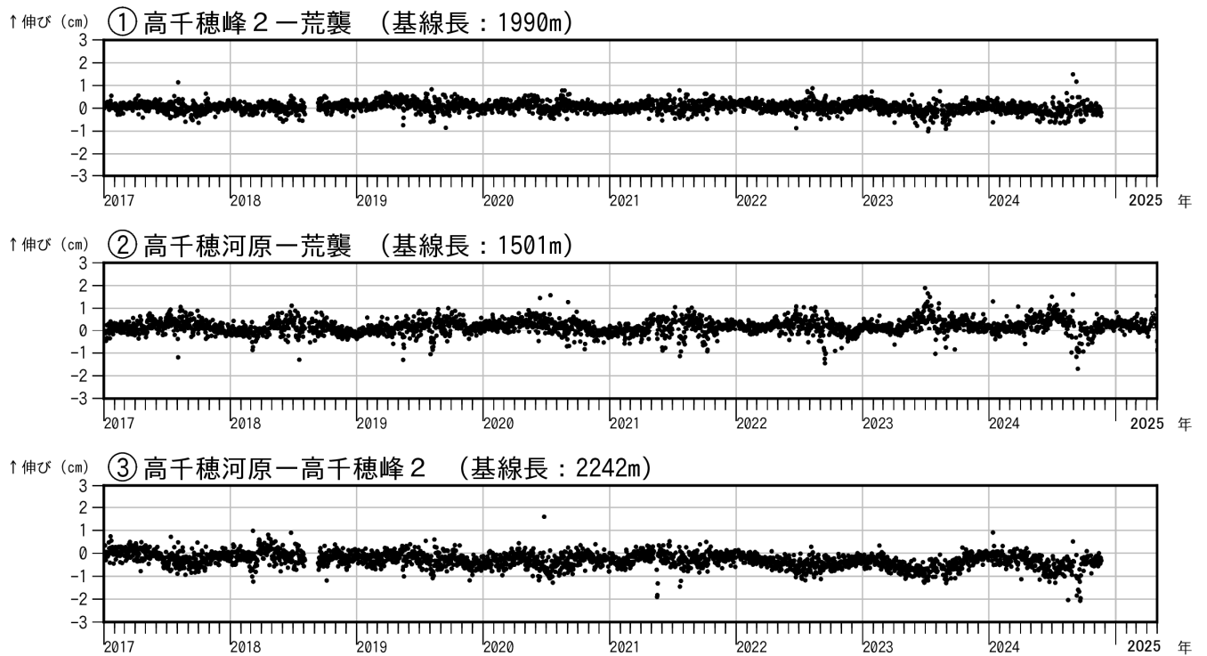
図4 霧島山（御鉢） GNSS 連続観測による基線長変化（2017年1月～2025年4月）
