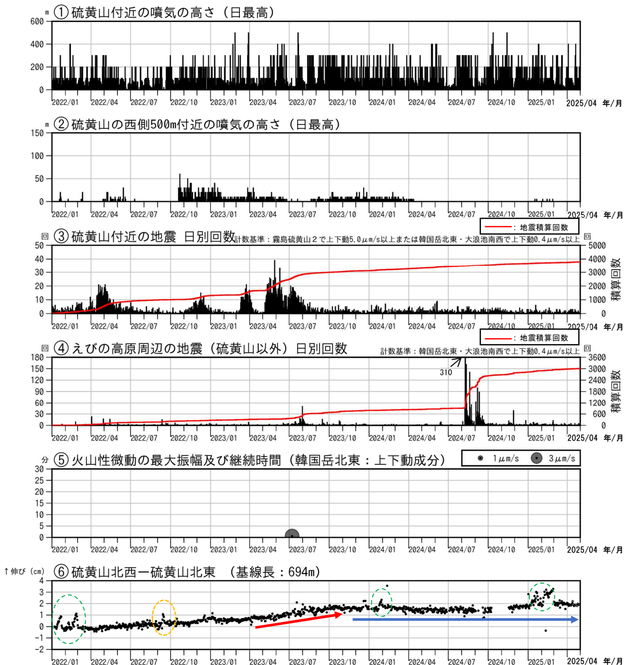
図2 霧島山（えびの高原（硫黄山）周辺） 火山活動経過図（2022年1月～2025年4月）
