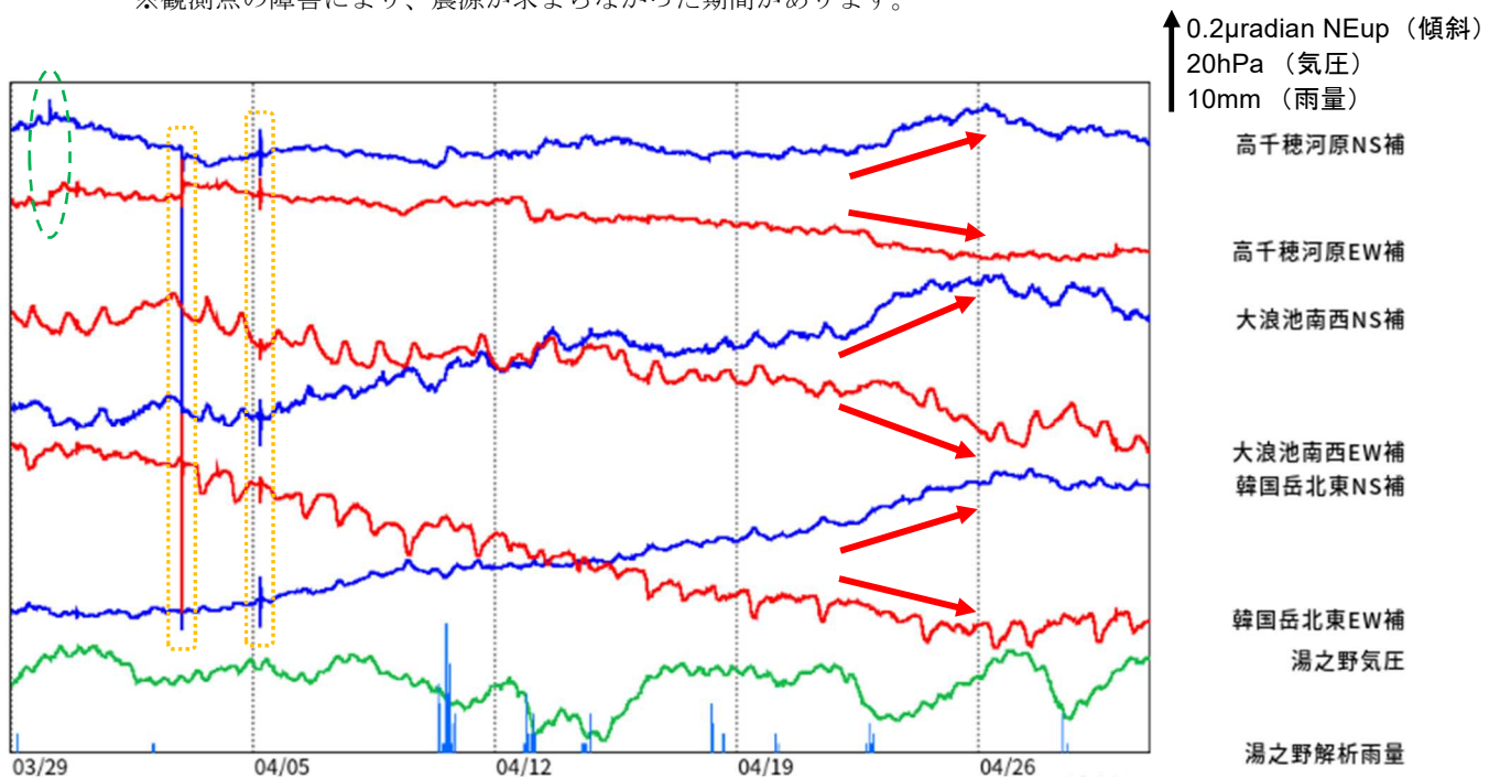
図 9 霧島山（新燃岳） 傾斜計による地殻変動の状況（分値）
