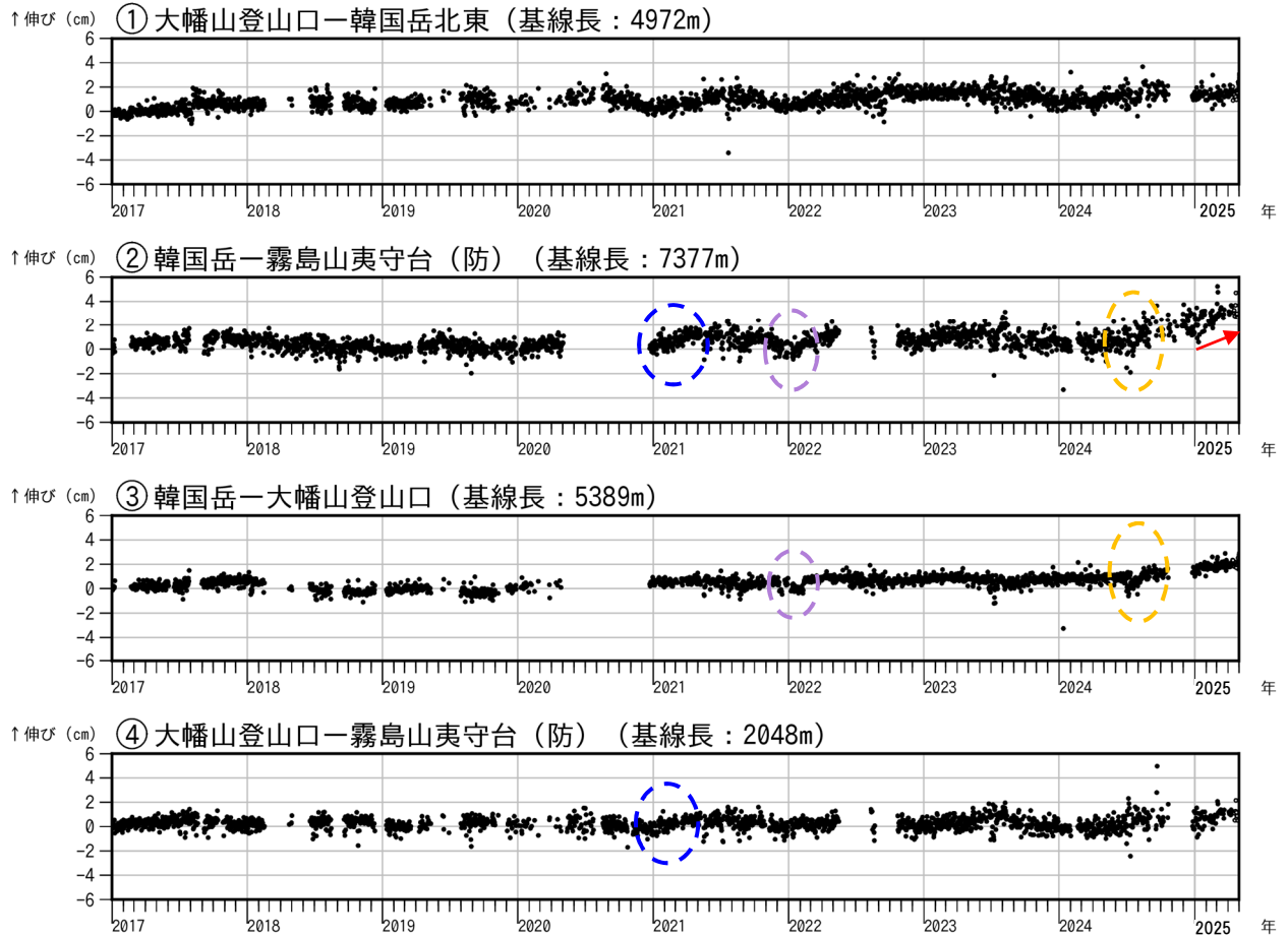
図4 霧島山（大幡池） GNSS 連続観測による基線長変化（2017年1月～2025年4月）
