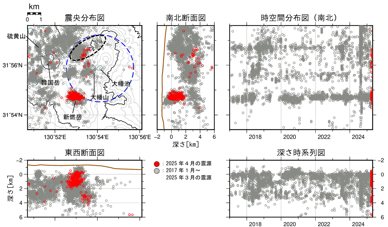
図3 霧島山（大幡池） 震源分布図（2017年1月～2025年4月）
