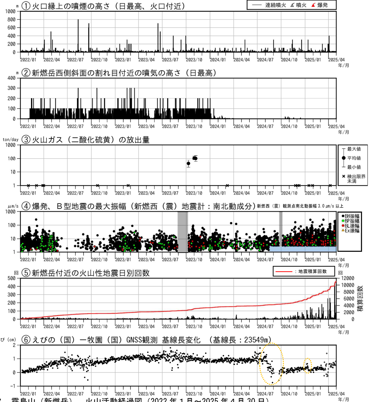
図7 霧島山（新燃岳） 火山活動経過図（2022年1月～2025年4月30日）
