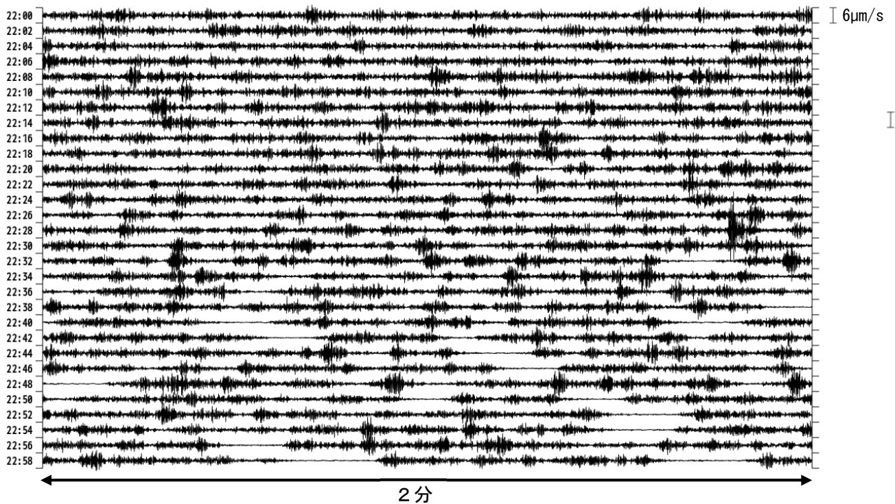
図5 霧島山（新燃岳） 27日に発生した火山性微動の状況（27日22時00分から1時間表示） （新燃西（震）地震計：速度波形上下動成分）
