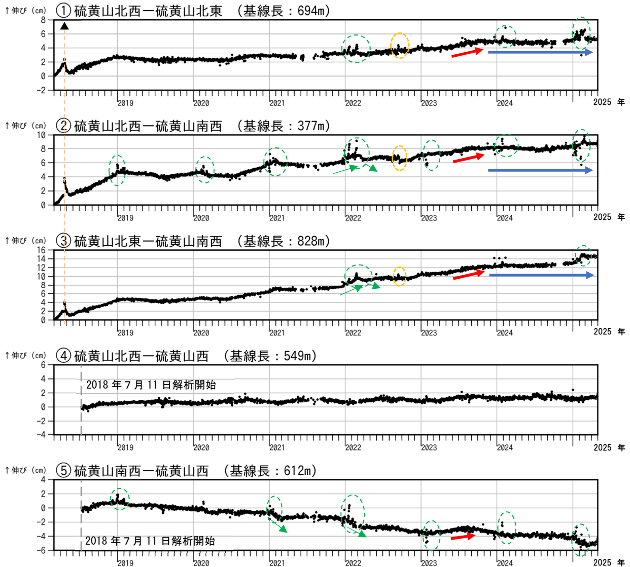
図4 霧島山（えびの高原（硫黄山）周辺） GNSS 連続観測による基線長変化（2018年3月～2025年4月）
