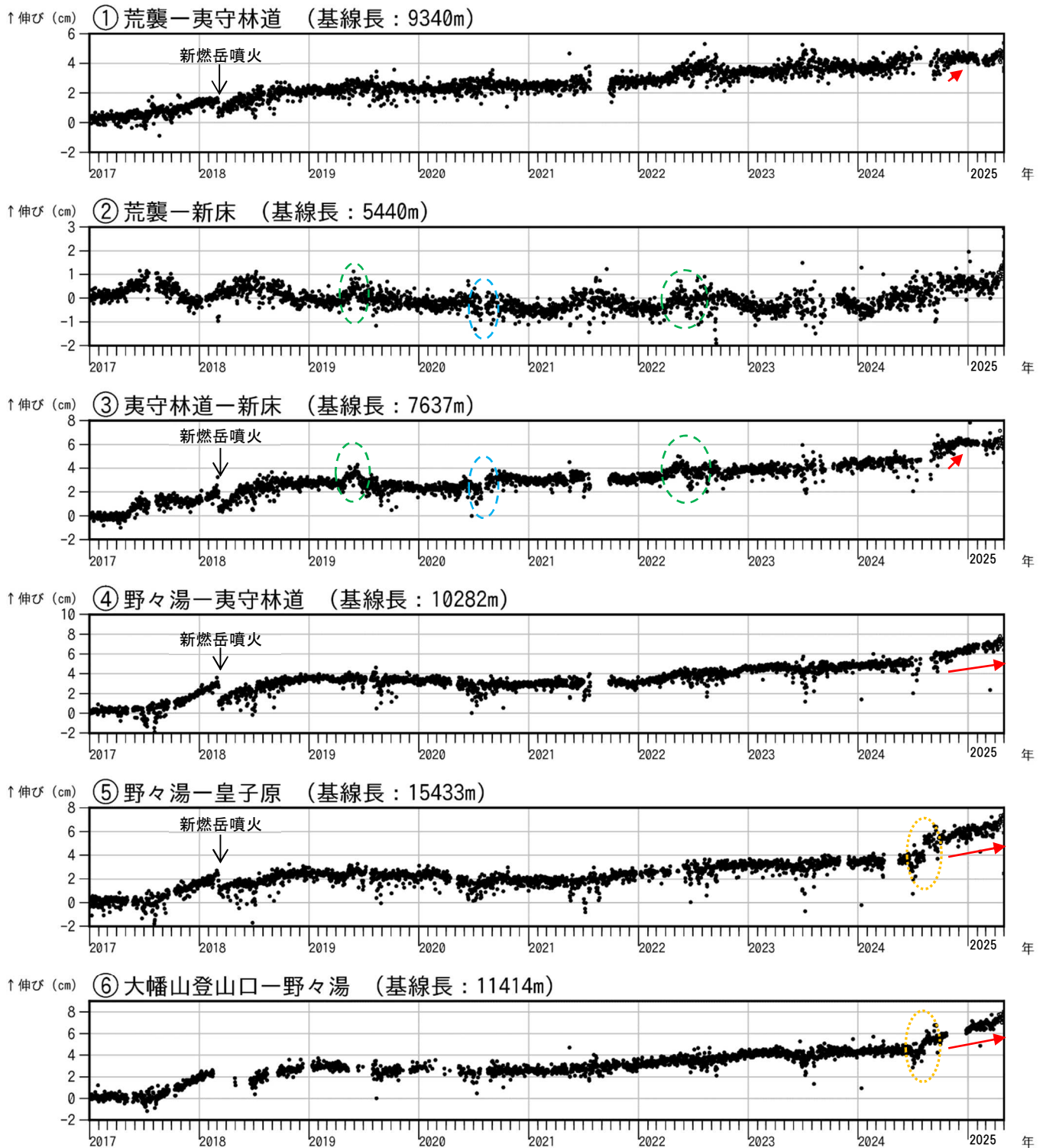
図10 霧島山（新燃岳） GNSS 連続観測による基線長変化（2017年1月～2025年4月）
