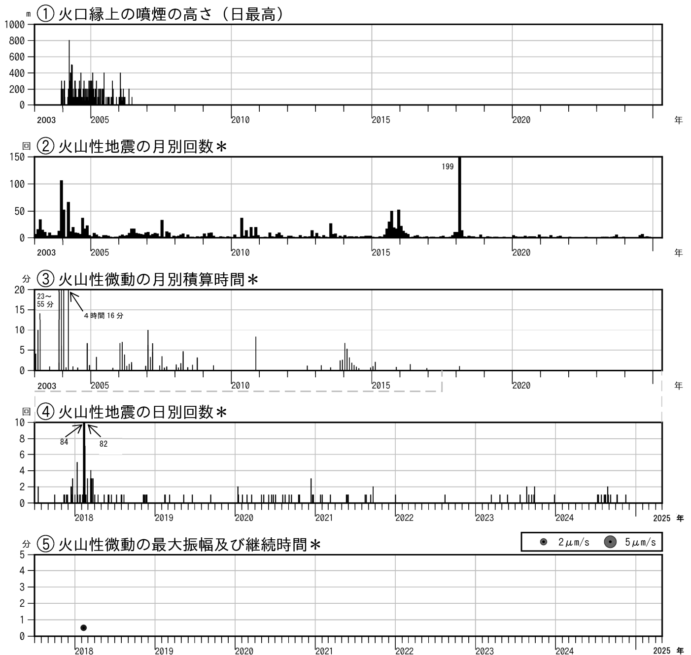
図3 霧島山（御鉢） 火山活動経過図（2003年1月～2025年4月）
