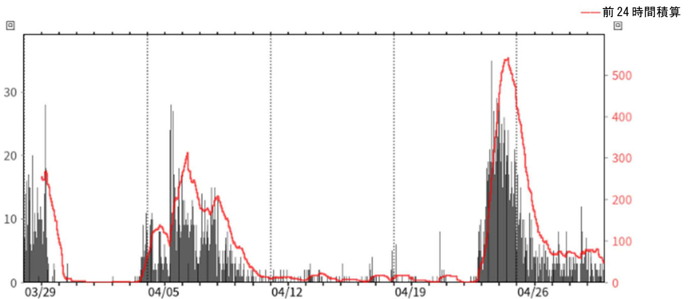
図 4 霧島山（新燃岳） 火山性地震の時間別回数及び前 24 時間積算回数（赤線） （2025 年 3 月 29 日（期間外）～ 4 月 30 日）
