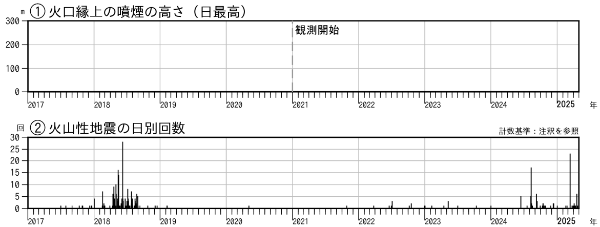
図2 霧島山（大幡池） 火山活動経過図（2017年1月～2025年4月）
