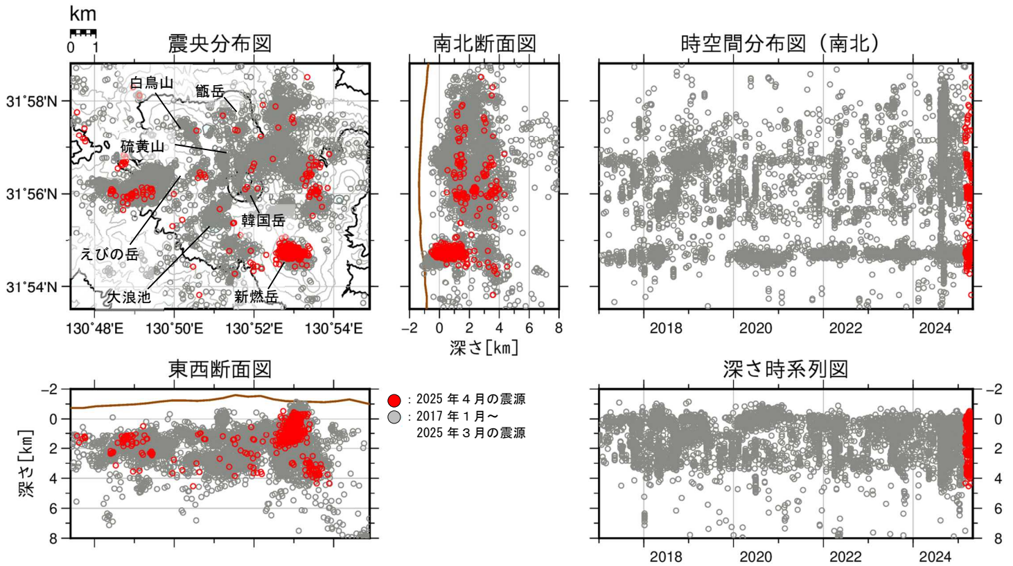
図 3 霧島山（えびの高原（硫黄山）周辺） 震源分布図（2017 年 1 月～2025 年 4 月）
