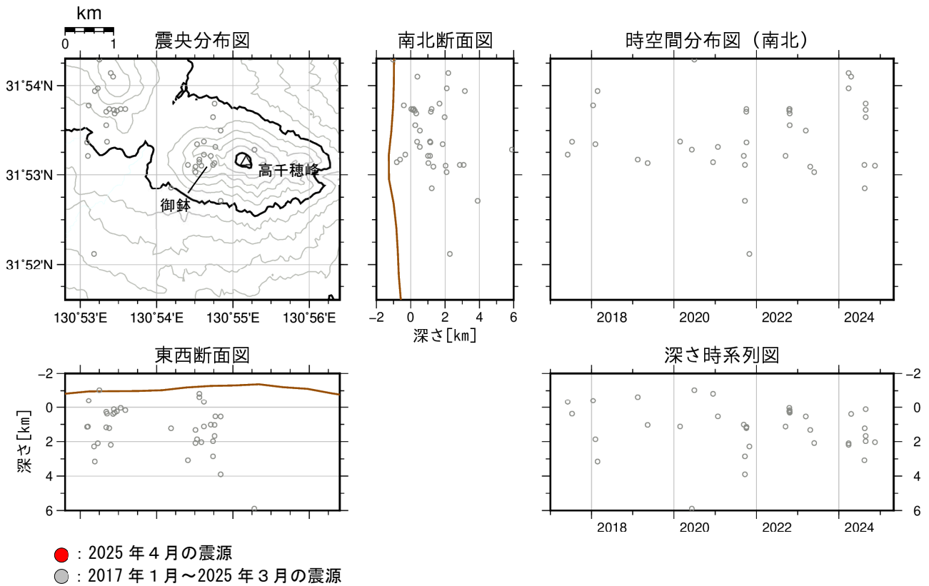
図2 霧島山（御鉢） 震源分布図（2017 年 1 月～2025 年 4 月）
