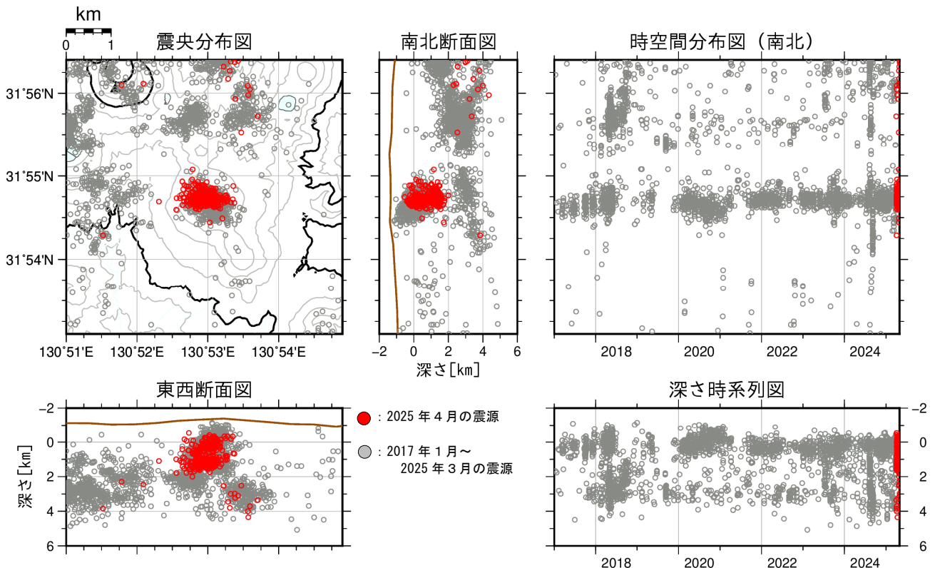
図 8 霧島山（新燃岳） 震源分布図（2017 年 1 月～2025 年 4 月）
