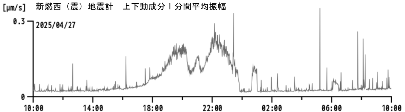
図6 霧島山（新燃岳） 27日の火山性微動発生前後の新燃西（震）地震計の振幅の状況 （2025年4月27日10時00分～4月28日10時00分）
