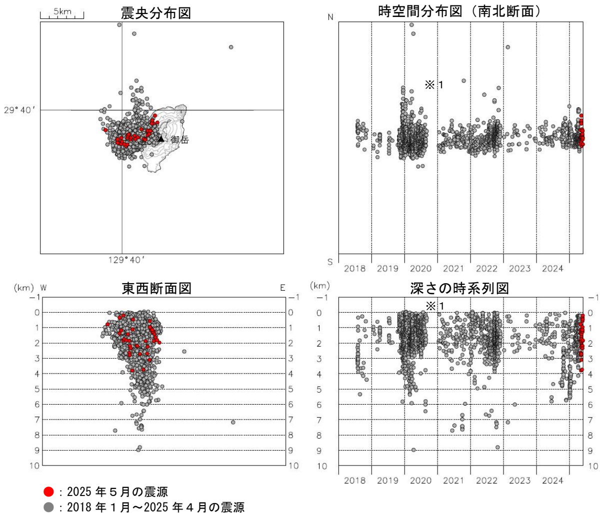
図 4 諏訪之瀬島 震源分布図（2018 年 1 月～2025 年 5 月）
