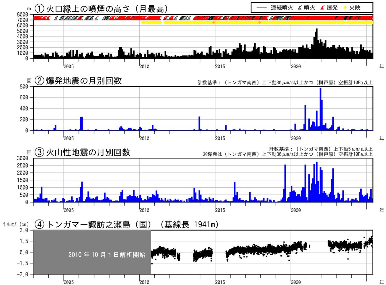
図2 諏訪之瀬島 長期の火山活動経過図（2003年1月～2025年5月）
