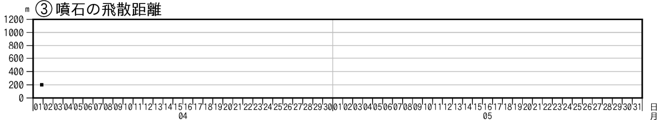
図5 諏訪之瀬島 ナベタオ観測点の傾斜変動と噴火活動（2025年4月～5月）
