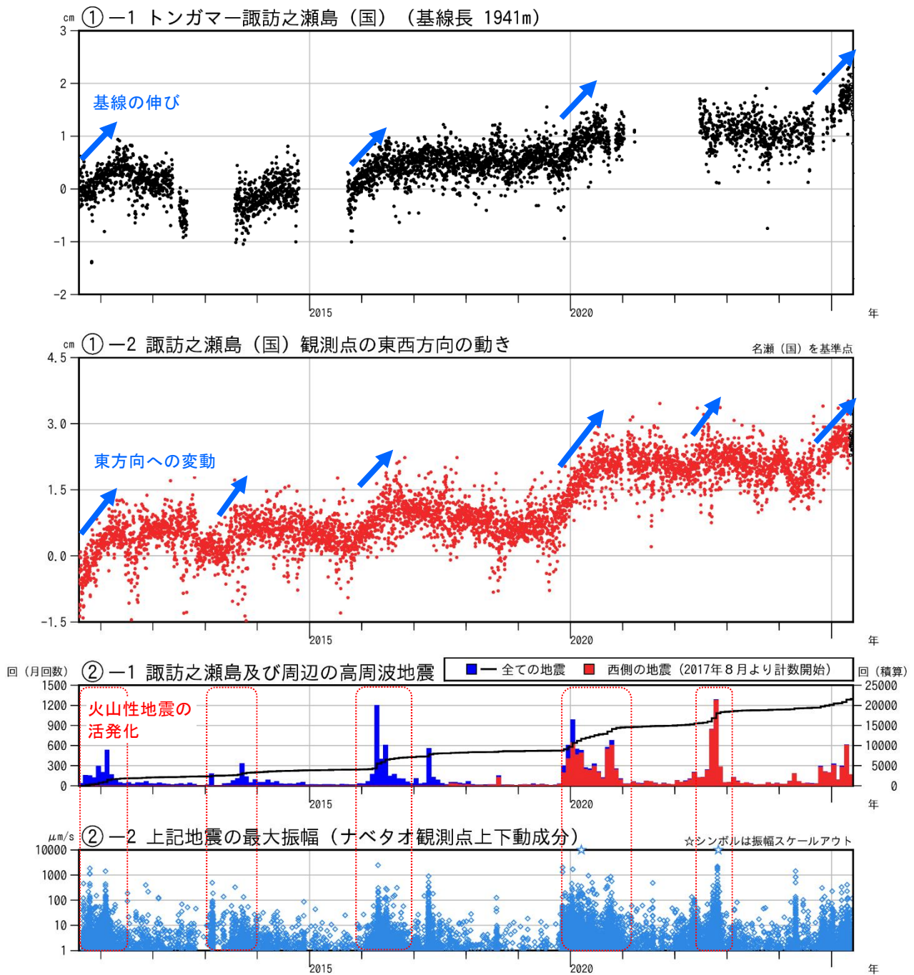
図6 諏訪之瀬島 GNSS連続観測と周辺の火山性地震（2010年8月～2025年5月）
