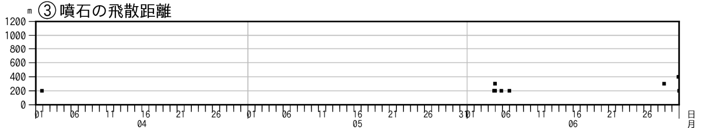
図5 諏訪之瀬島 ナベタオ観測点の傾斜変動と噴火活動（2025年4月～6月）
