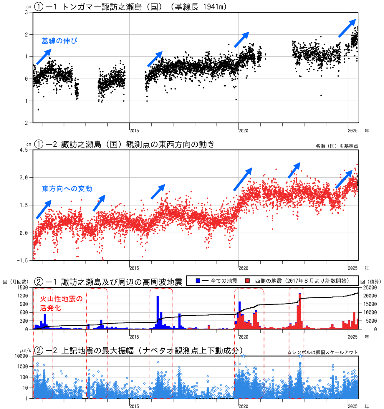
図6 諏訪之瀬島 GNSS連続観測と周辺の火山性地震（2010年8月～2025年6月）
