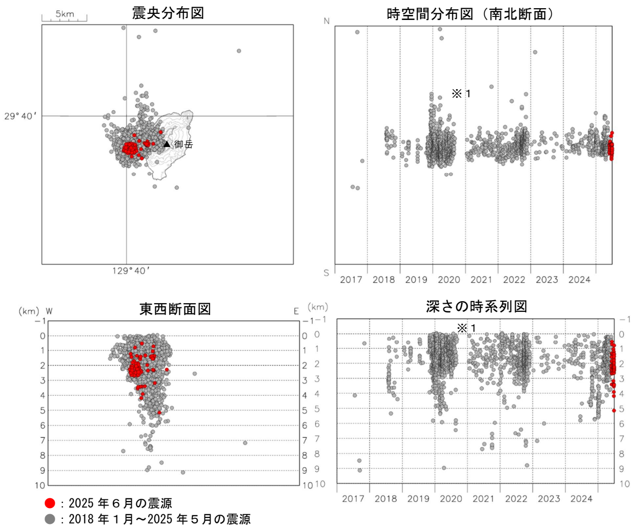
図4 諏訪之瀬島 震源分布図（2017年1月～2025年6月）
