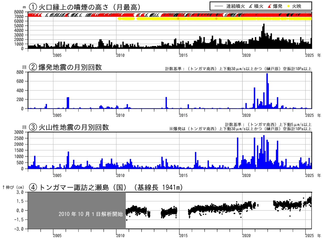
図 2 諏訪之瀬島 長期の火山活動経過図（2003 年 1 月～2025 年 6 月）
