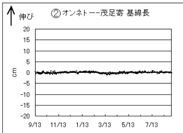
雌阿寒岳基線長グラフ（2001年9月13日～2002年8月31日）
