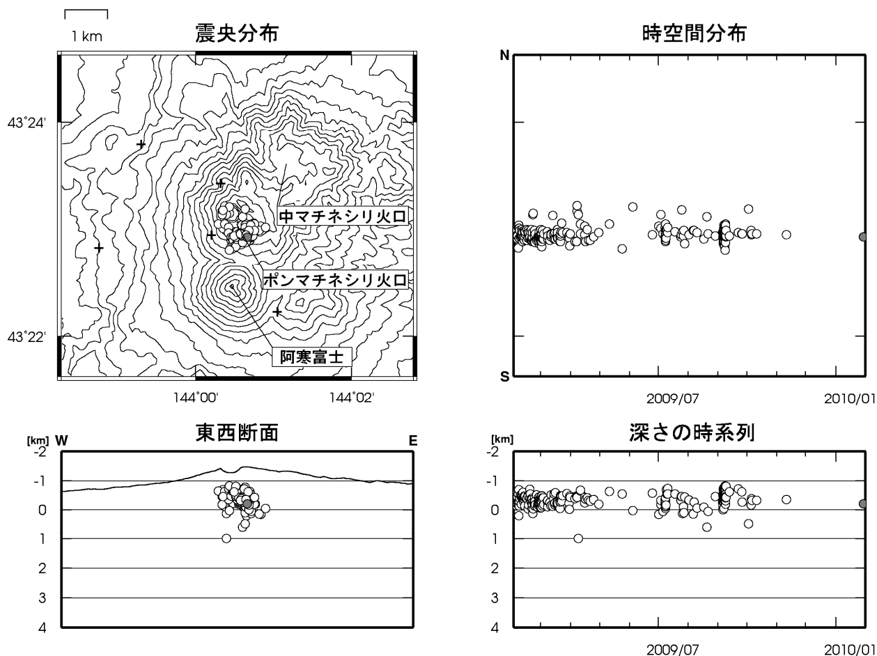
図 6 雌阿寒岳 震源分布図(2009 年 2 月～2010 年 1 月) +は地震観測点
