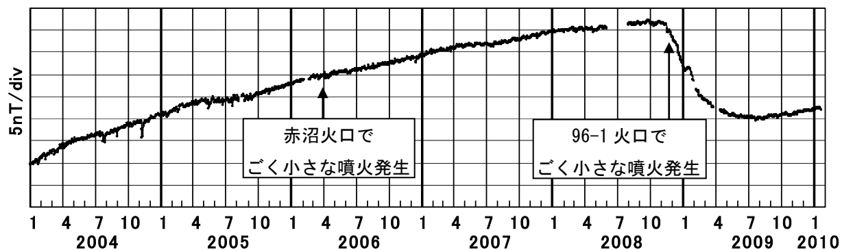
図 4 雌阿寒岳 全磁力連続観測結果（2004 年 1 月 1 日～2010 年 1 月 22 日） MEA と地磁気観測所女満別出張所の全磁力単純差（日平均値） 図 5 の MEA（◎）にて測定
