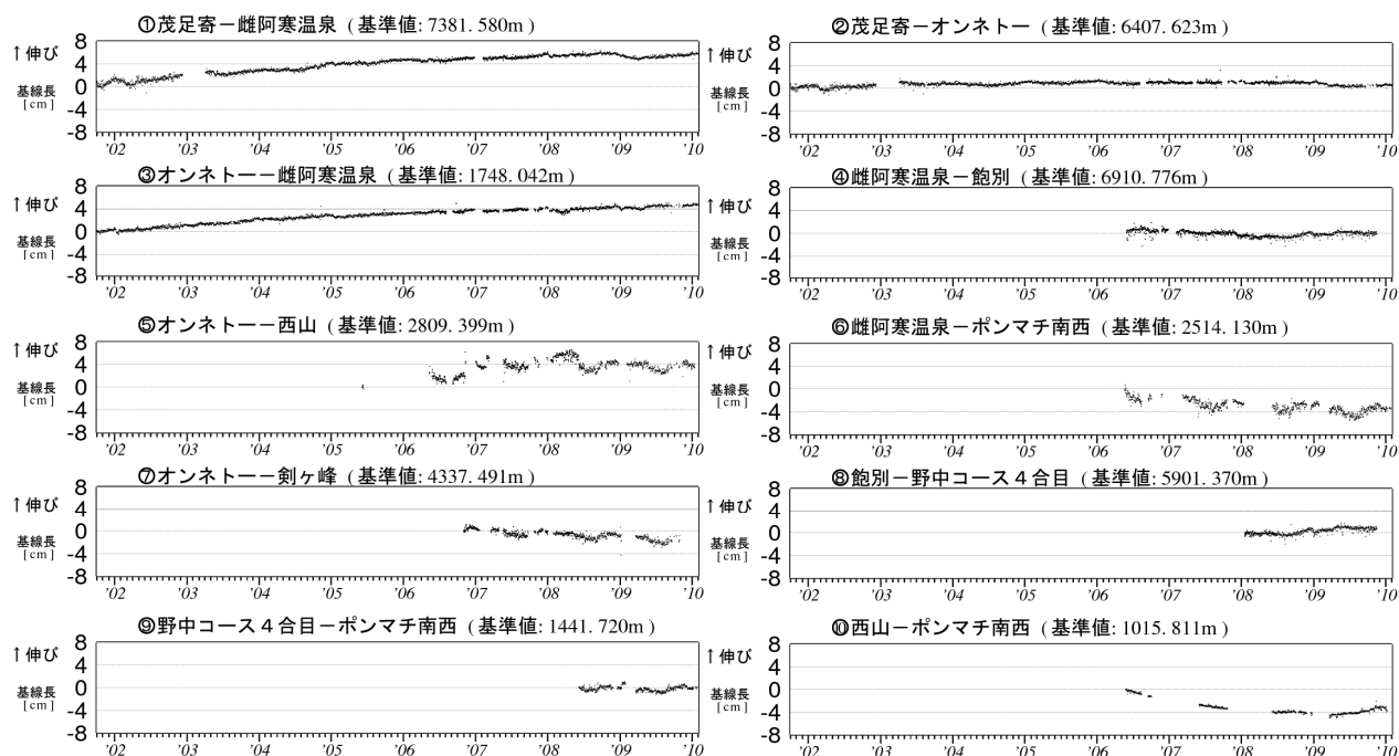
図 7 ※ 雌阿寒岳 GPS 連続観測による基線長変化（2001 年 10 月～2010 年 1 月）
