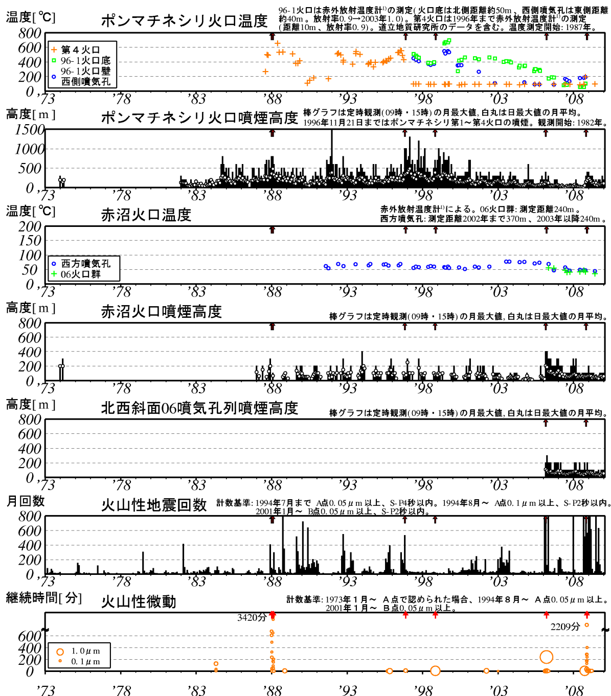
図2※ 雌阿寒岳 長期の火山活動経過図(1973年1月～2010年1月) ↑印は噴火 (1988年、1996年、1998年、2008年:ポンマチネシリ火口南東側からの噴火、2006年:赤沼火口からの噴火)
