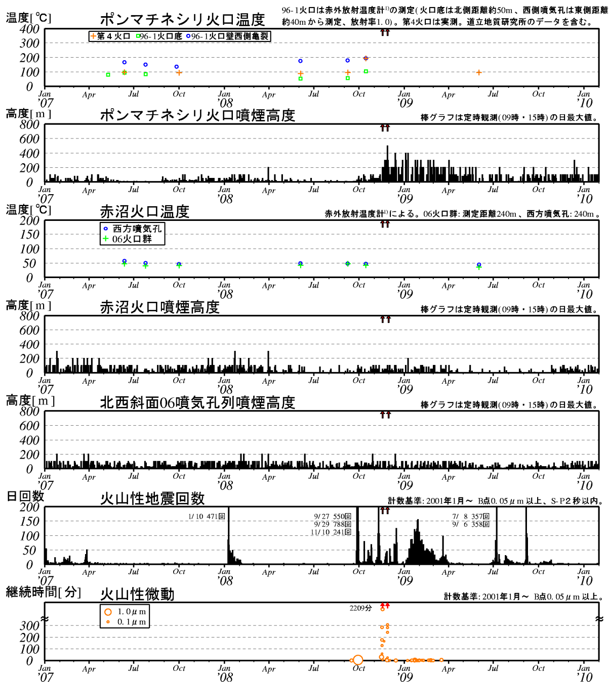
図3※ 雌阿寒岳 最近の火山活動経過図（2007年1月～2010年1月） ↑印は噴火
