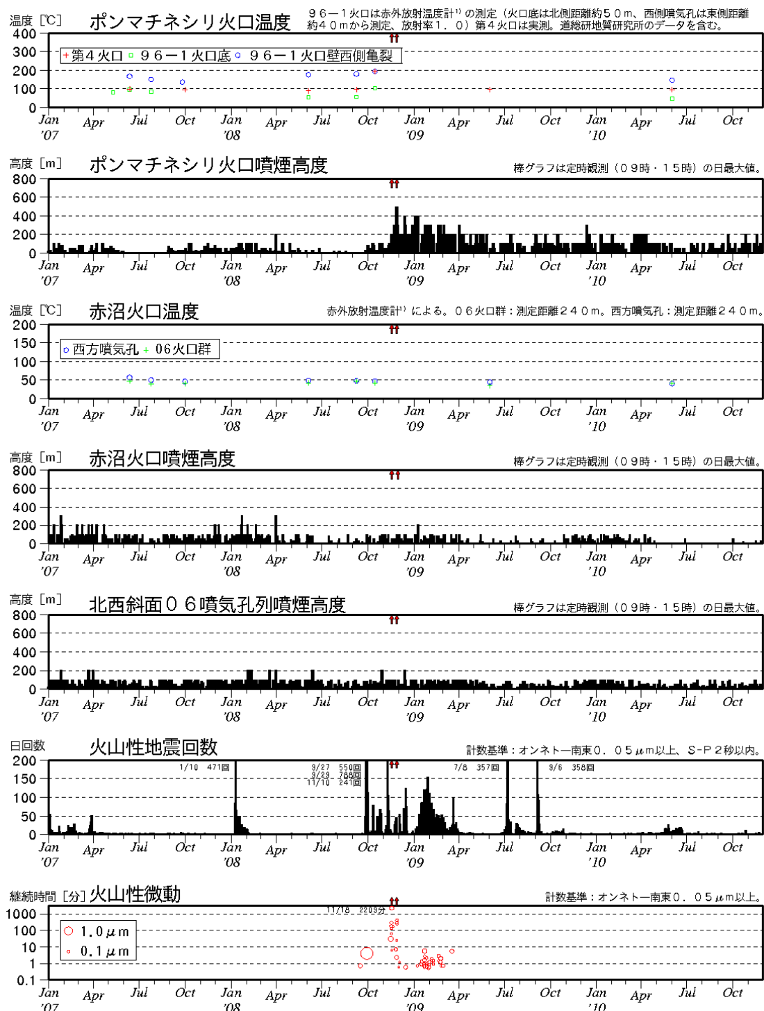
図 2 ※ 雌阿寒岳 最近の火山活動経過図（2007 年 1 月～2010 年 11 月） ↑印は噴火
