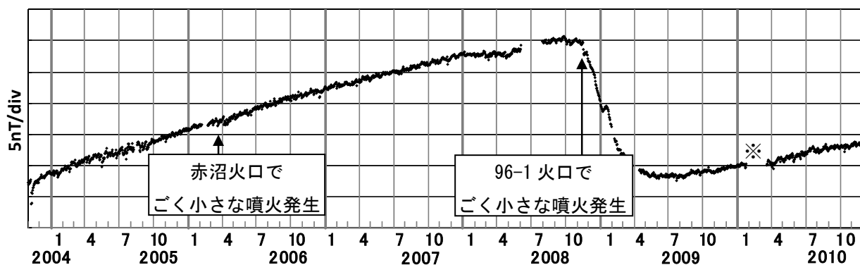
図3 雌阿寒岳 全磁力連続観測結果（2004年10月1日～2010年11月28日） MEAと地磁気観測所女満別出張所の全磁力単純差（日平均値、年周変化補正） 図4のMEA（◎）にて測定 ※ソーラーパネルへの着雪によりバッテリー電圧が低下し、欠測。
