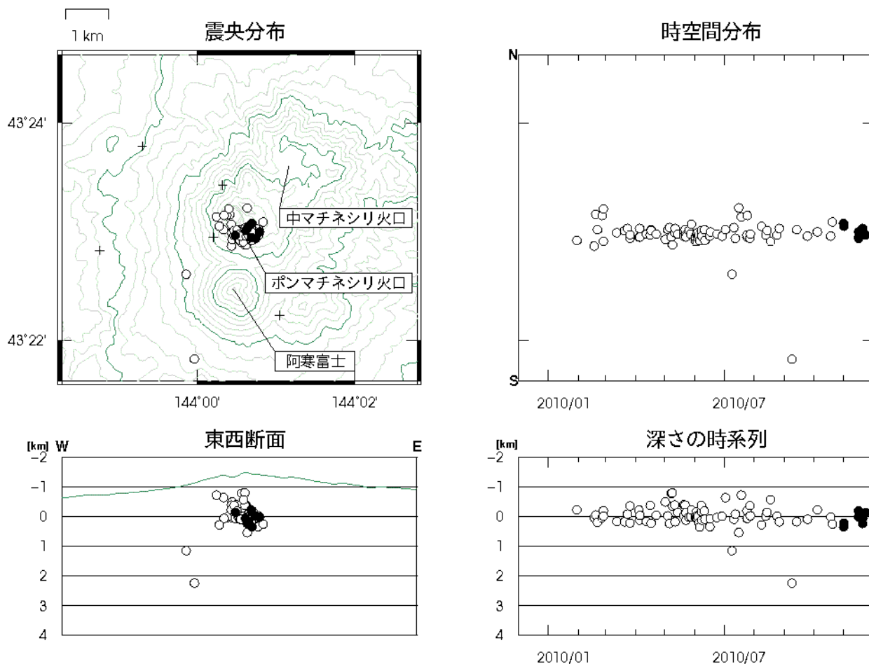
図 5 雌阿寒岳 震源分布図(2009 年 12 月～2010 年 11 月) +は地震観測点
