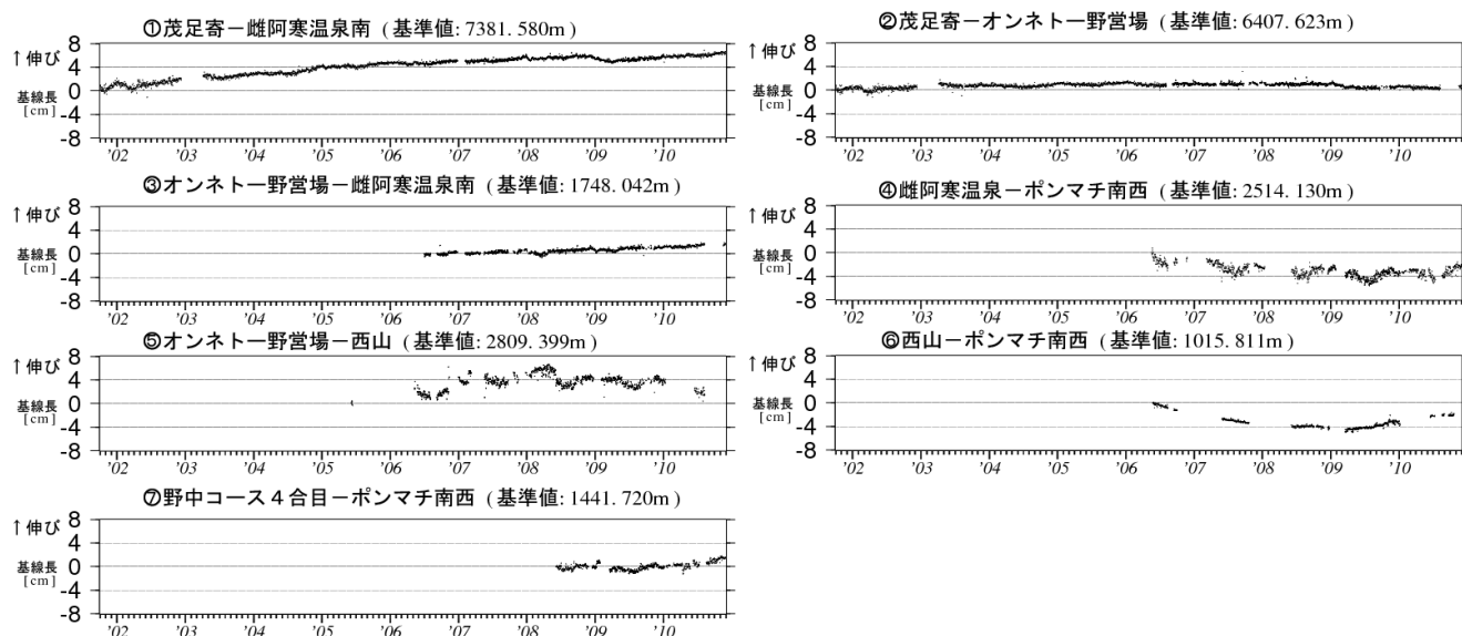
図 6※ 雌阿寒岳 GPS 連続観測による基線長変化（2001 年 10 月～2010 年 11 月）
