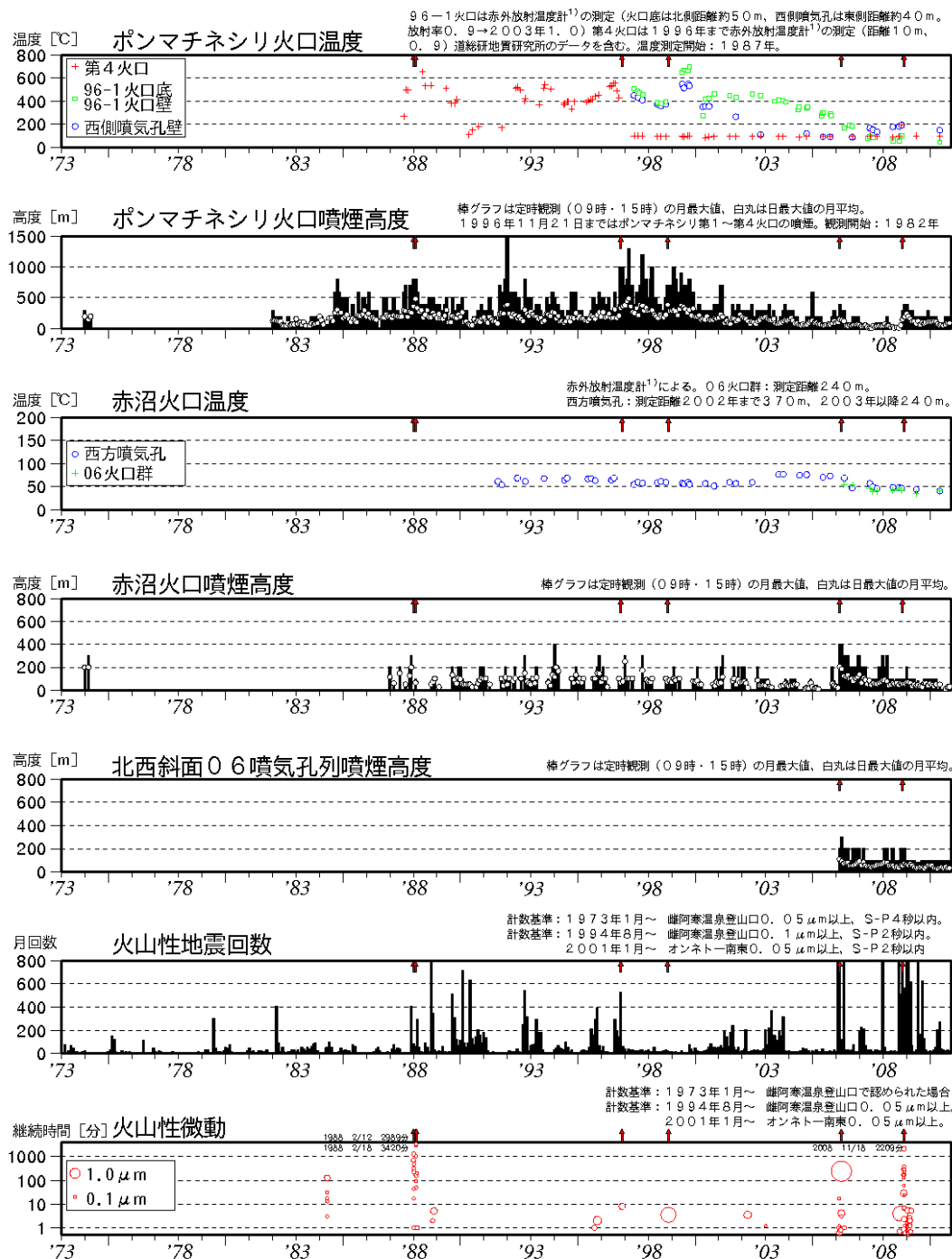
図 1 ※ 雌阿寒岳 長期の火山活動経過図（1973 年 1 月～2010 年 11 月） ↑印は噴火 （1988 年、1996 年、1998 年、2008 年：ポンマチネシリ火口南東側からの噴火、2006 年：赤沼火口からの噴火）
