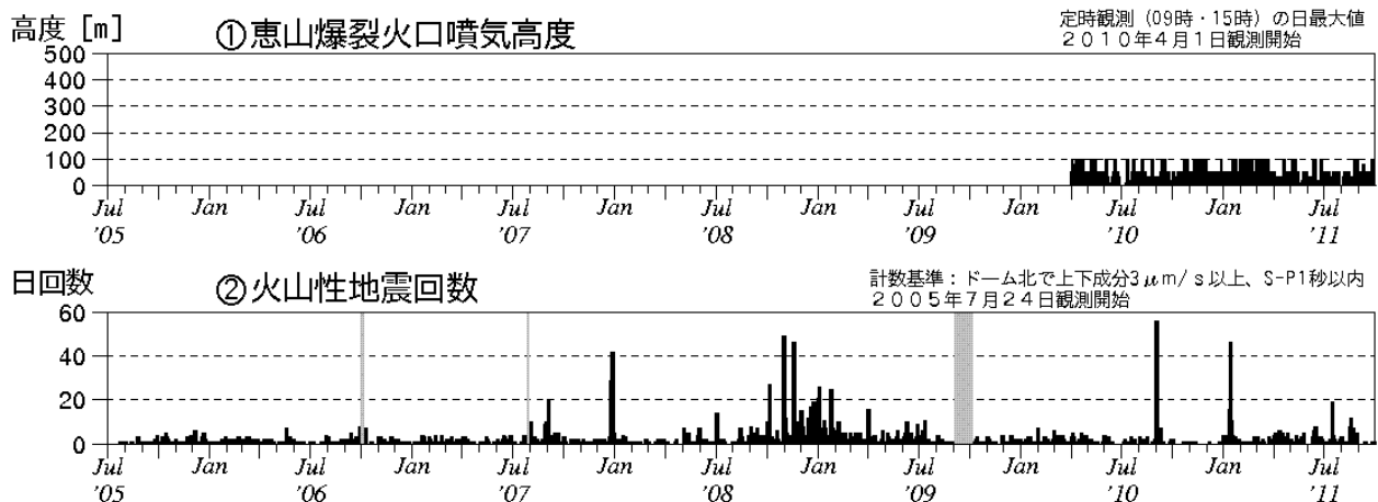
図 1 恵山 火山活動経過図（2005 年 7 月～2011 年 9 月）
