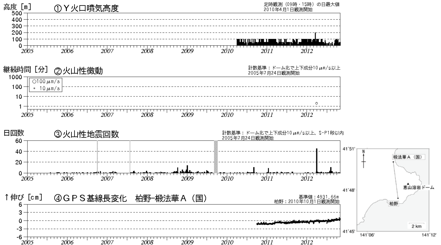
図 2 ※ 恵山 火山活動経過図（2005年 7 月～2012年10月）、GPS連続観測点配置図
