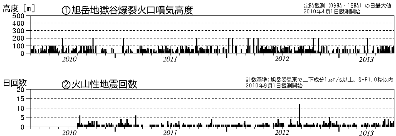
図1 大雪山 火山活動経過図（2010年4月～2013年6月）
