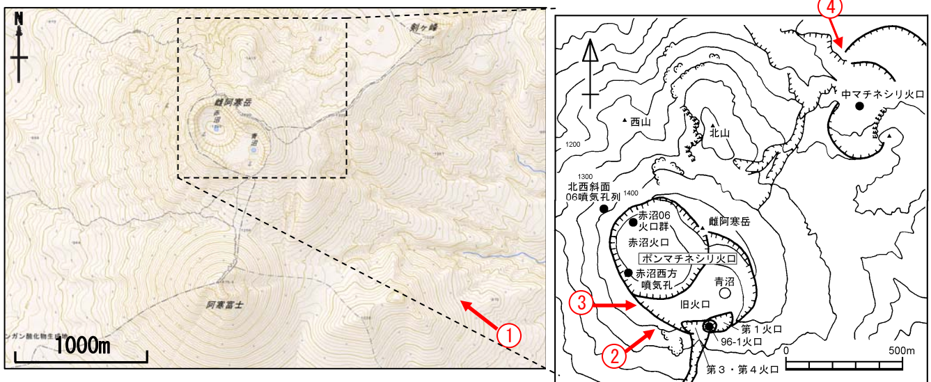
図 3 雌阿寒岳 周辺図（左）と火口周辺図（右）、写真の撮影方向（矢印）
