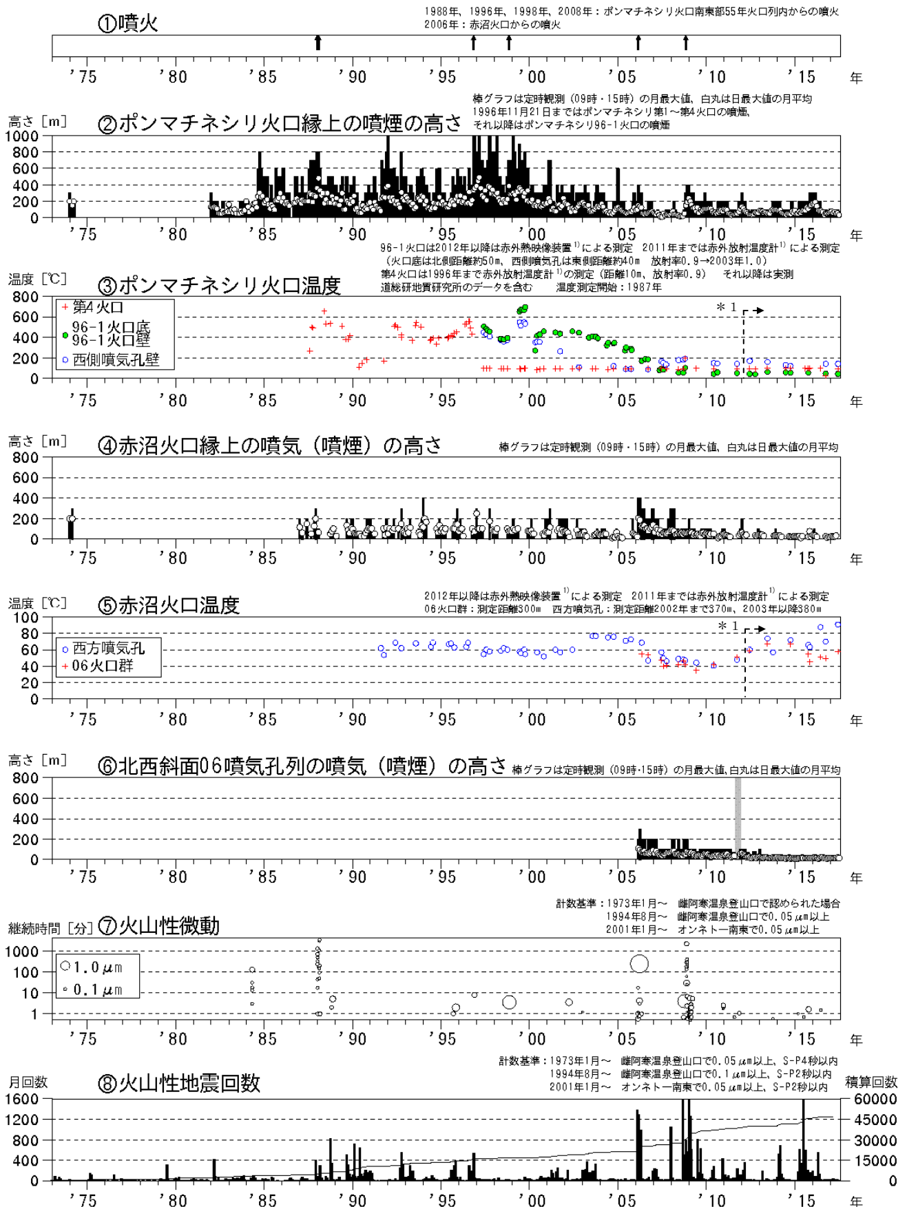
図1 雌阿寒岳 火山活動経過図（1973年1月～2017年7月）
