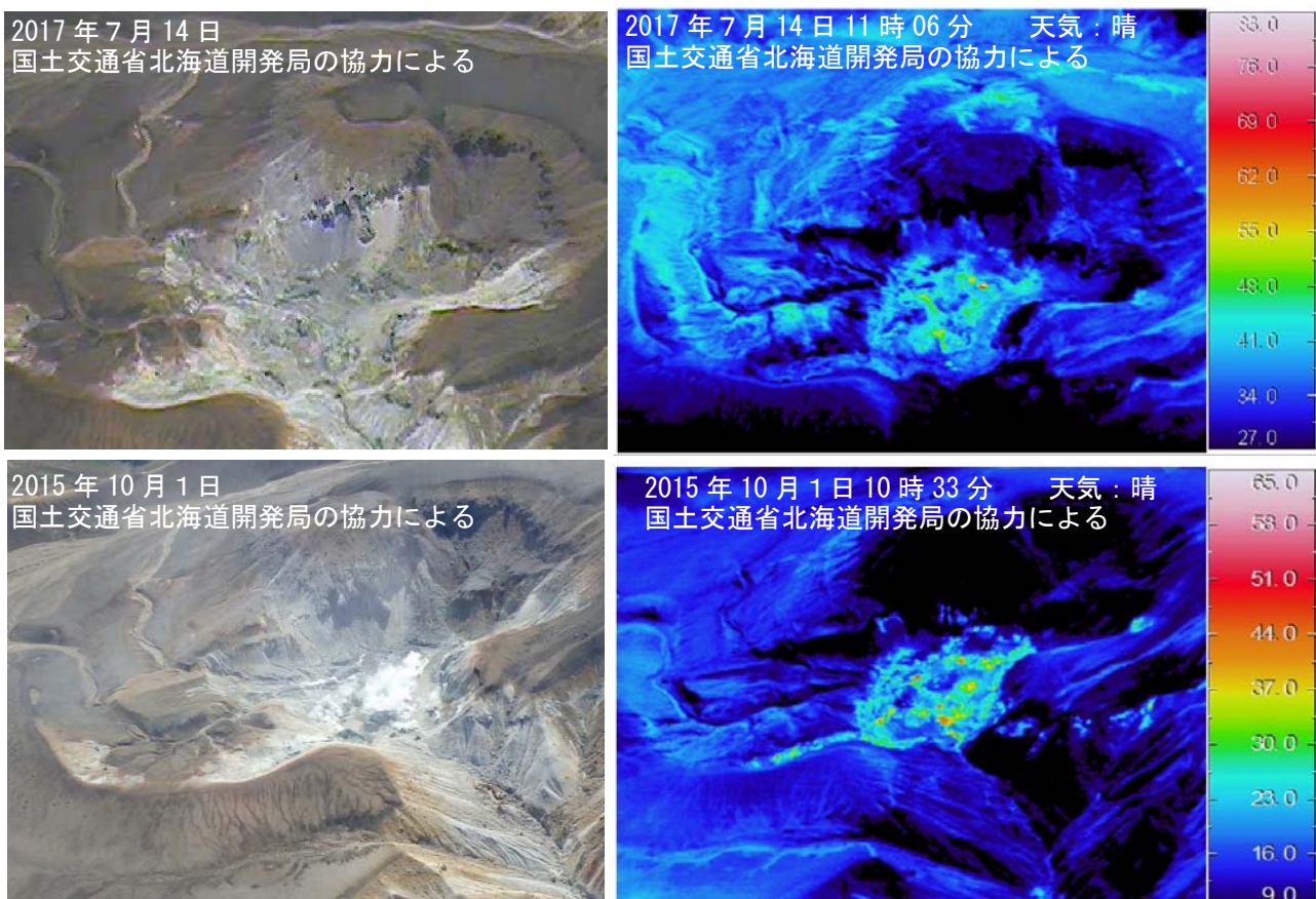
図 6 雌阿寒岳 中マチネシリ火口の地表面温度分布 図 3 の④から撮影
