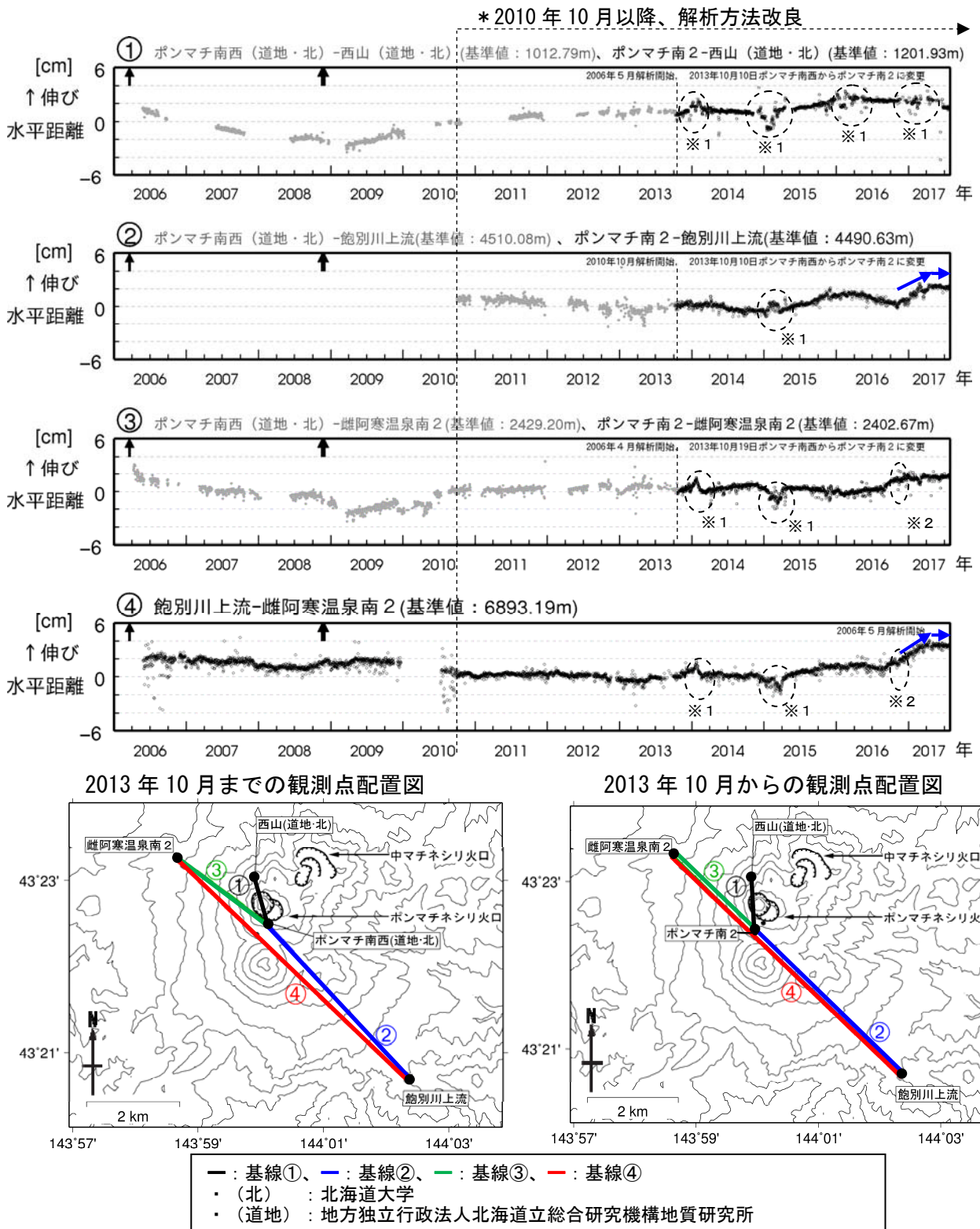
図10 雌阿寒岳 GNSS連続観測による水平距離変化（2006年4月～2017年7月）及び観測点配置図
