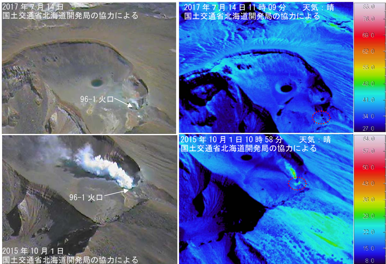
図 5 雌阿寒岳 ポンマチネシリ火口
