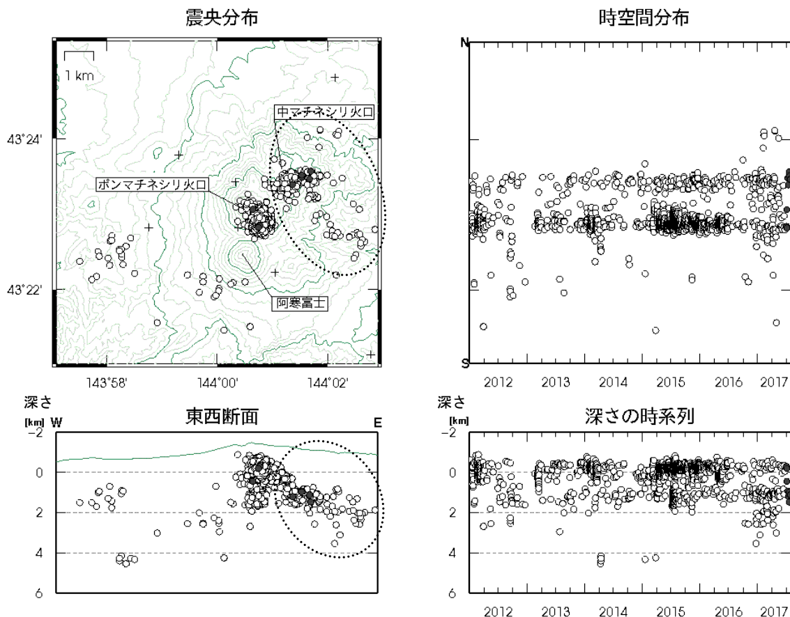
図 9 雌阿寒岳 火山性地震の震源分布（2012年1月～2017年7月）
