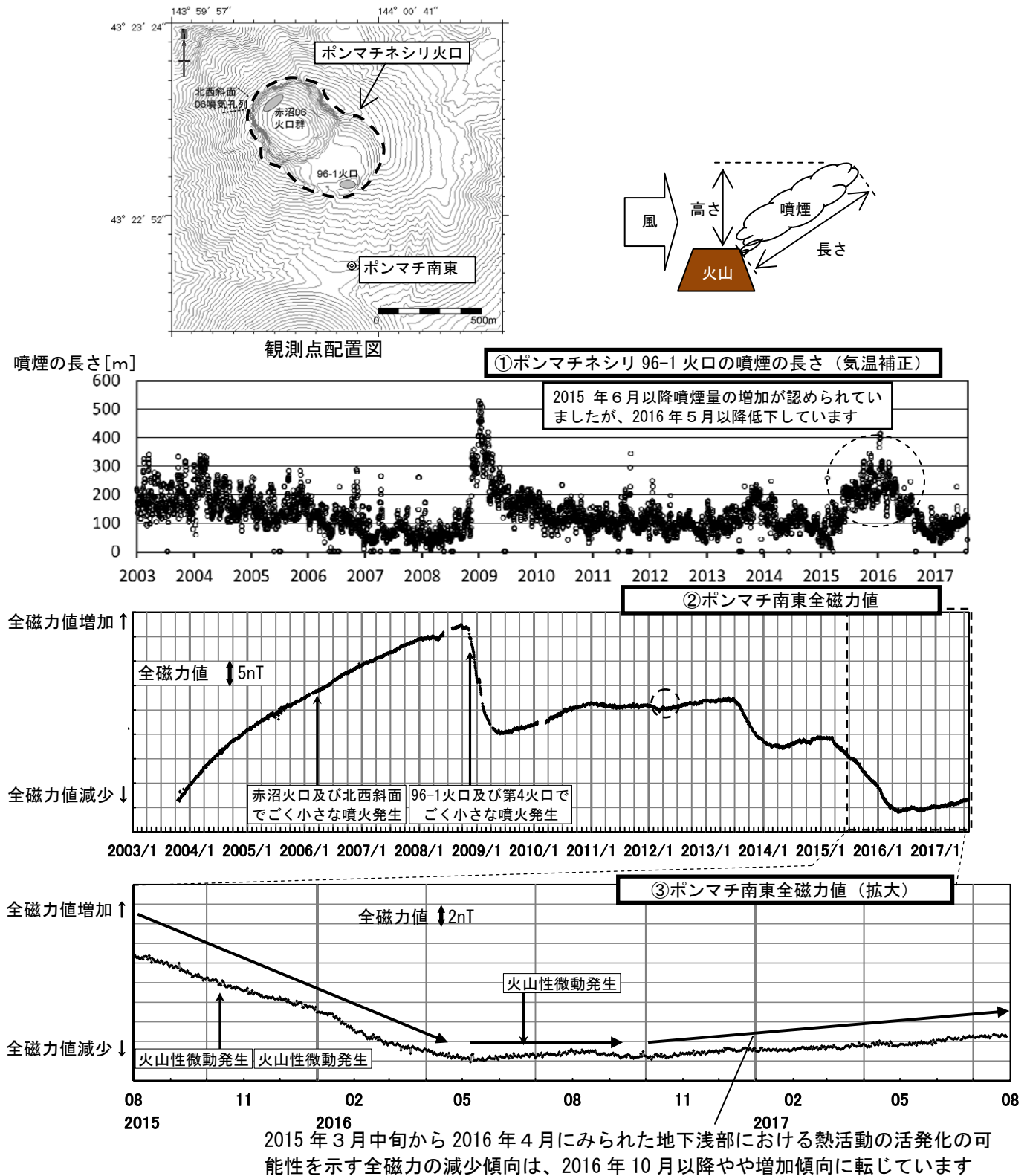
図 7 雌阿寒岳 浅部の火山活動の変化と全磁力観測点配置図
