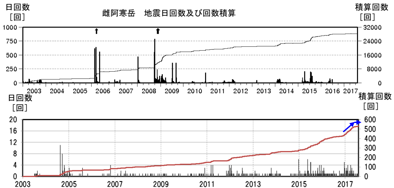
図 8 雌阿寒岳 火山性地震の日回数及び積算回数推移（2003年1月～2017年7月）
