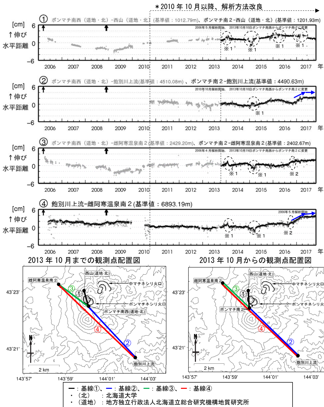
図 7 雌阿寒岳 GNSS連続観測による水平距離変化（2006年4月～2017年10月）及び観測点配置図
