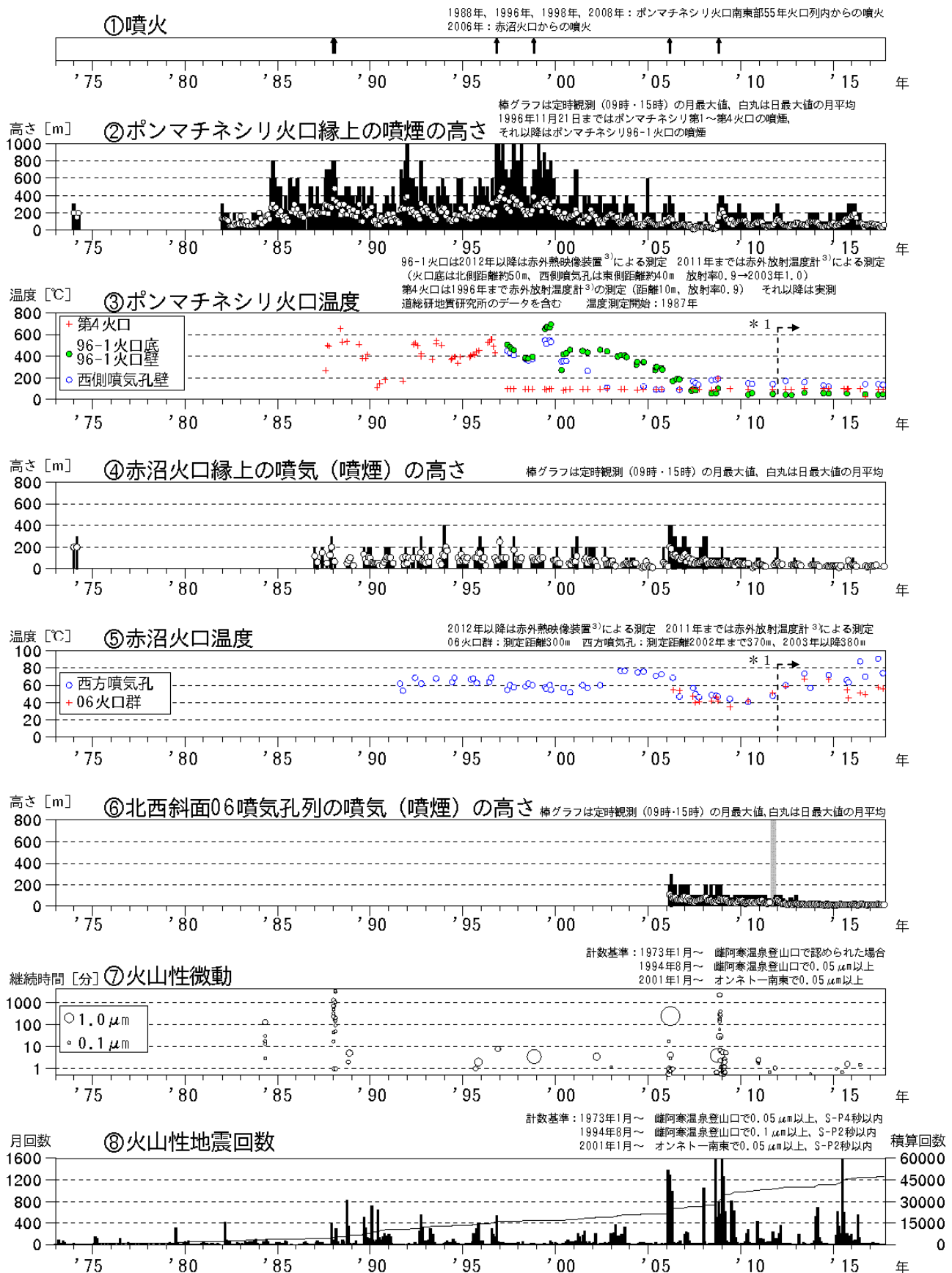
図1 雌阿寒岳 火山活動経過図（1973年1月～2017年10月）
