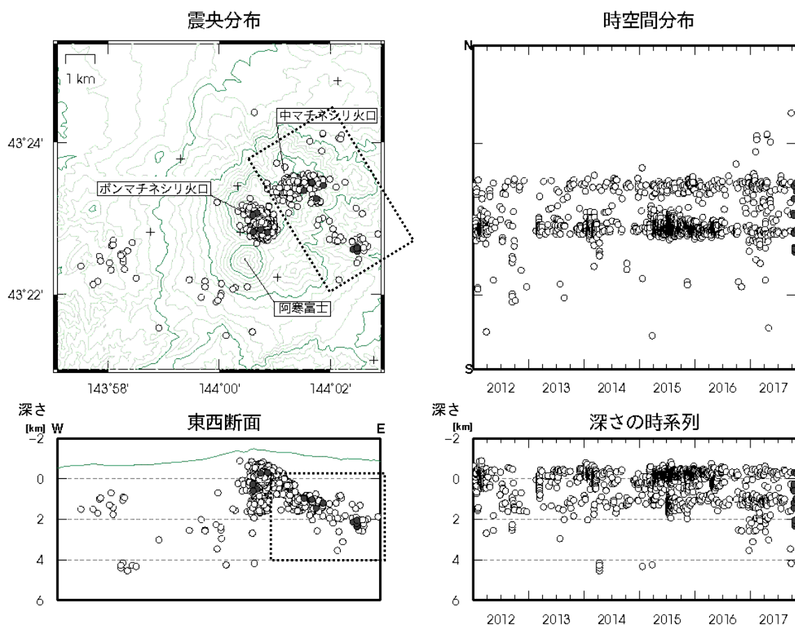
図6 雌阿寒岳 火山性地震の震源分布（2012年1月～2017年10月）
