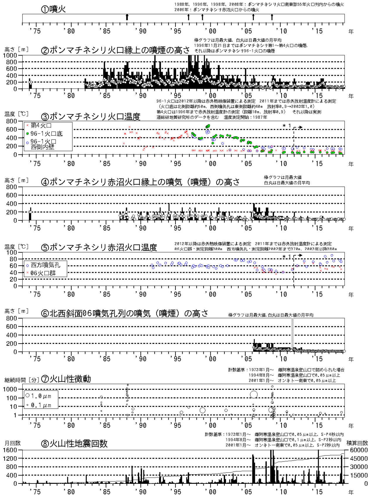
図 1 雌阿寒岳 火山活動経過図（1973年 1 月～2019年 3 月）
