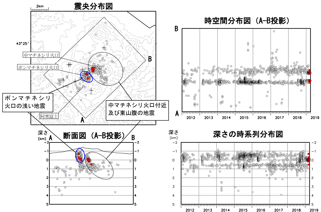
図 6 雌阿寒岳 火山性地震の震源分布（2012年1月～2019年3月）
