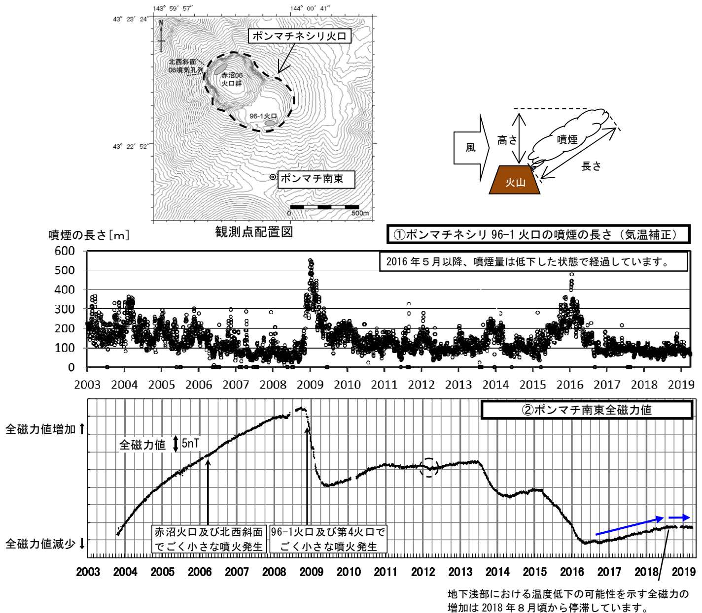
図 4 雌阿寒岳 ポンマチネシリ96-1火口の噴煙の長さ、全磁力の比較及び全磁力観測点配置図
