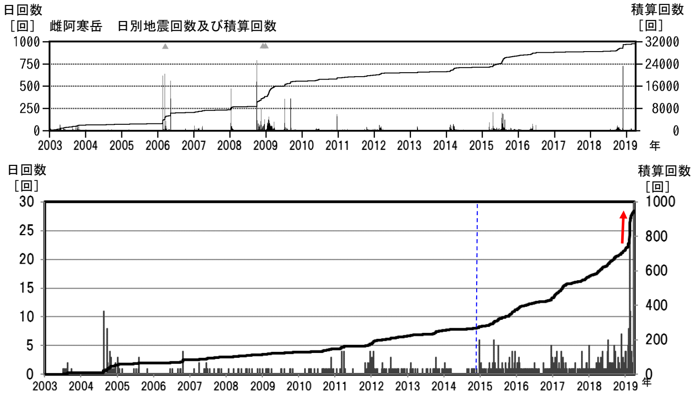
図 5 雌阿寒岳 火山性地震の日別回数及び積算回数（2003年 1 月～2019年 3 月）
