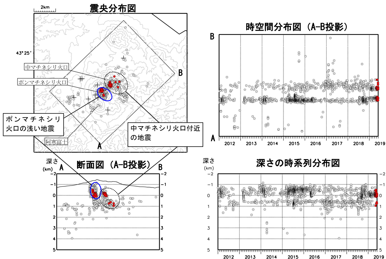
図9 雌阿寒岳 火山性地震の震源分布（2012年1月～2019年5月）
