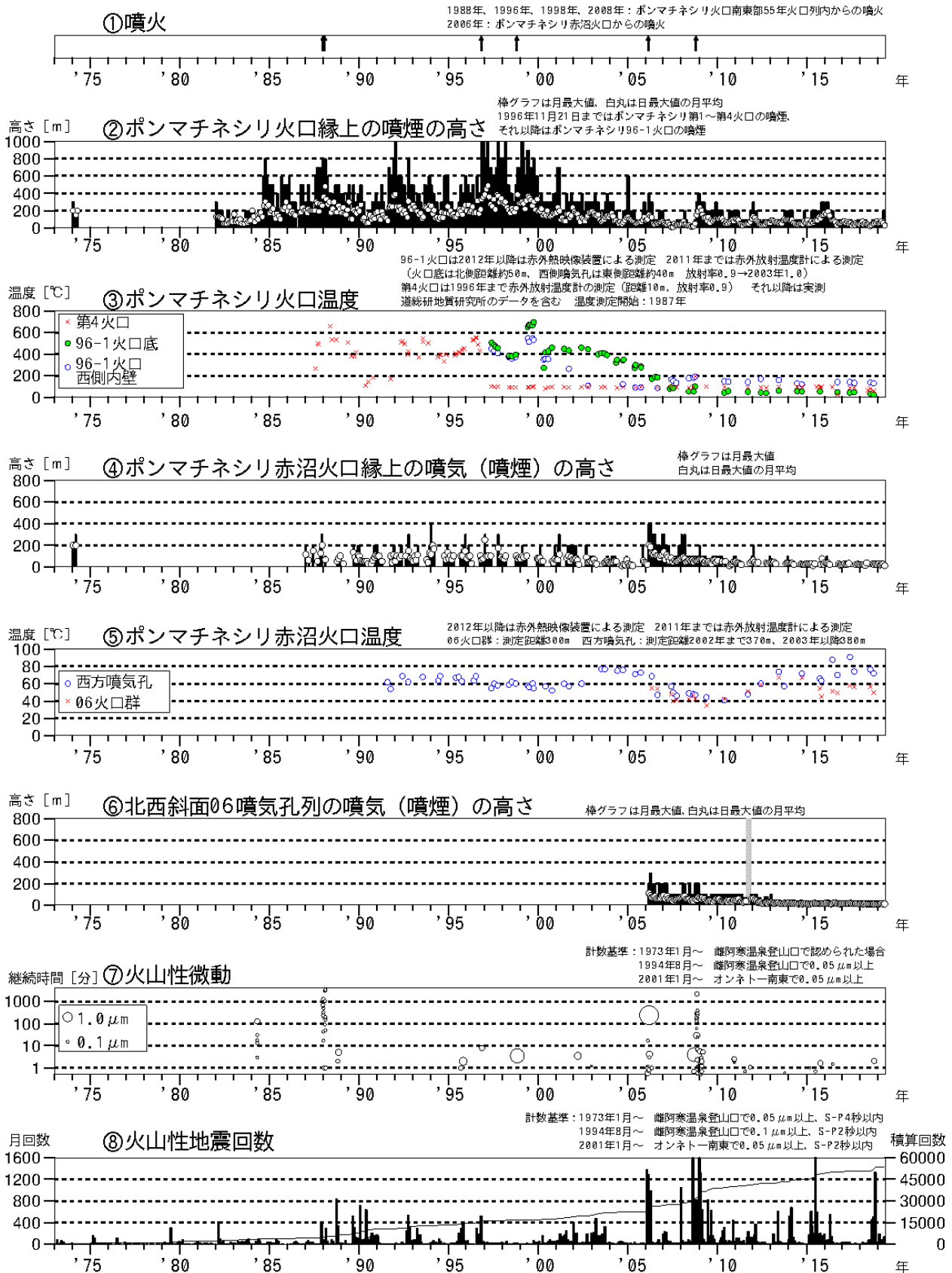
図1 雌阿寒岳 火山活動経過図（1973年1月～2019年5月）
