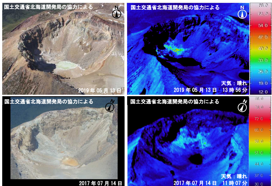
図5 雌阿寒岳 赤外熱映像装置による赤沼火口の地表面温度分布 上：南側上空（図2の②）から撮影 下：南東側上空（図2の①）から撮影
