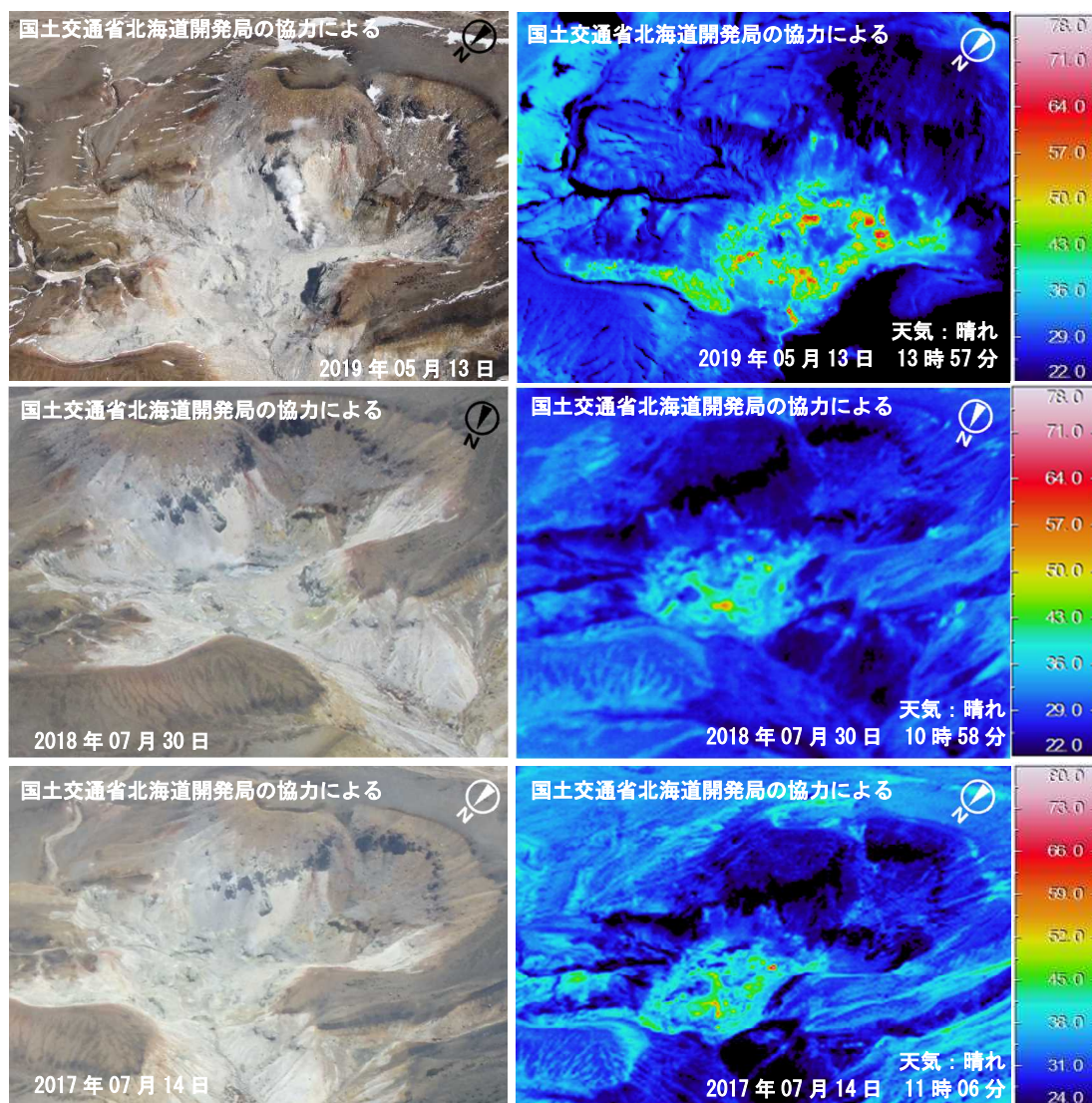
図6 雌阿寒岳 赤外熱映像装置による中マチネシリ火口の地表面温度分布 上、中、下：北西側上空（図2の③）から撮影 ・中マチネシリ火口内の地表面温度分布に特段の変化は認められませんでした。
