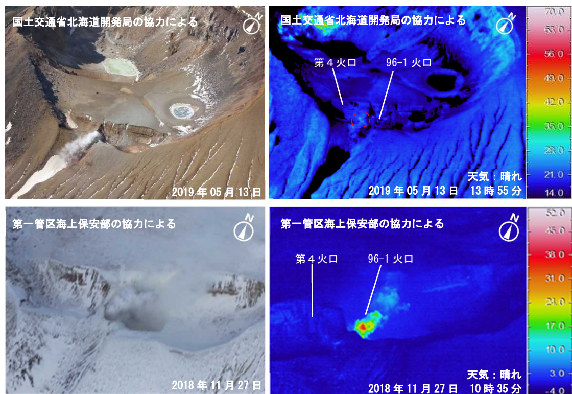
図4 雌阿寒岳 赤外熱映像装置によるポンマチネシリ96-1火口及び第4火口の地表面温度分布 上、下：南東側上空（図2の①）から撮影
