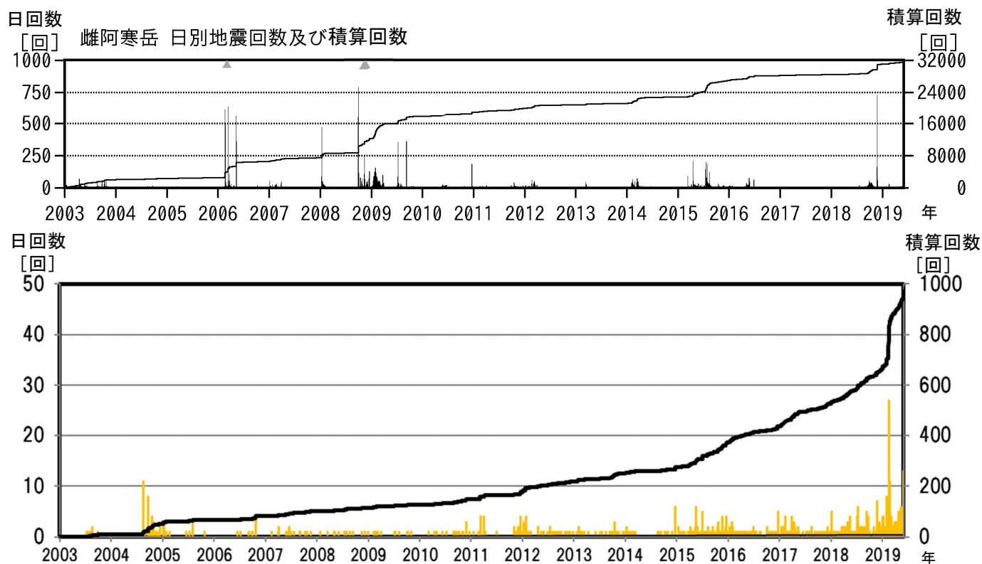
図8 雌阿寒岳 火山性地震の日別回数及び積算回数（2003年1月～2019年5月）
