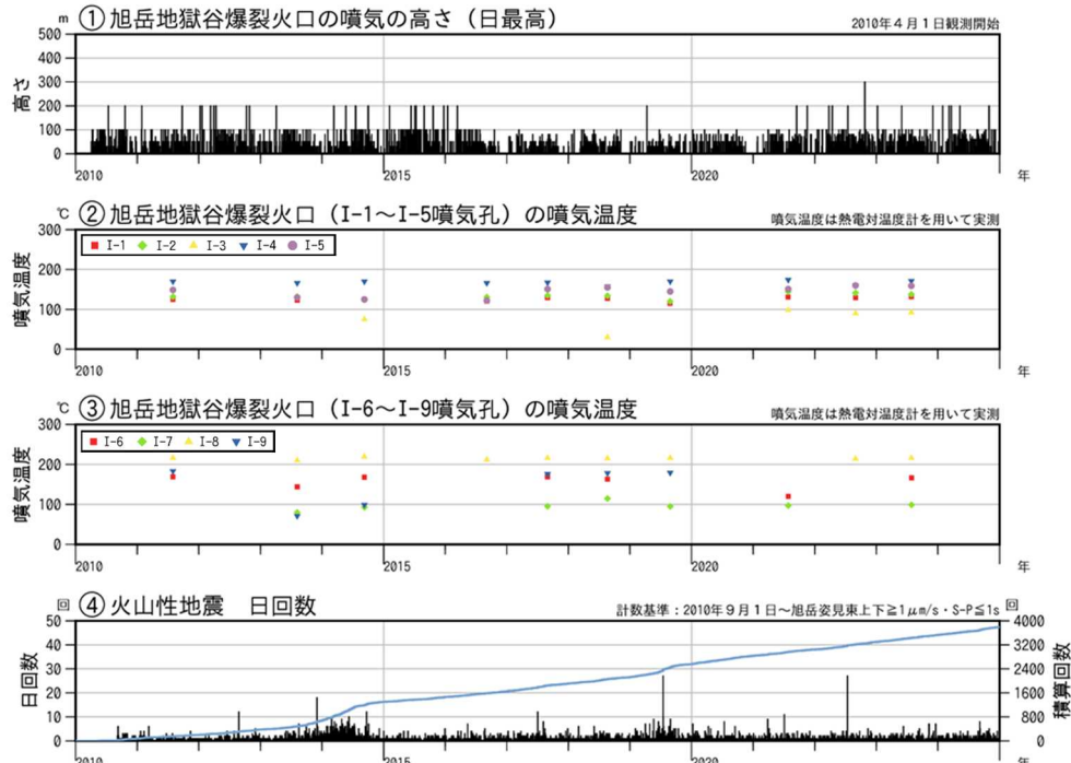
図1 大雪山 火山活動経過図（2010年4月～2024年12月）
