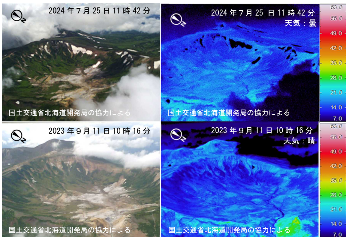
図5 大雪山 赤外熱映像観測装置による御鉢平の地表面温度分布 上段：北東側上空（図3の③）から撮影 下段：北東側上空（図3の④）から撮影 ・2023年9月の観測結果と比べて、地表面温度分布に特段の変化は認められませんでした。
