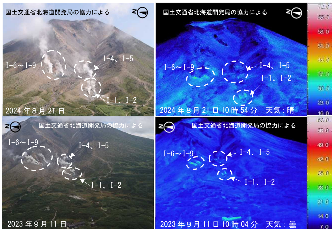
図4 大雪山 赤外熱映像観測装置による旭岳地獄谷爆裂火口の地表面温度分布 上段：西側上空（図3の①）から撮影 下段：西側上空（図3の②）から撮影 ・2023年9月の観測結果と比較して、旭岳地獄谷爆裂火口の噴気の状態や地表面温度分布に特段の変化は認められませんでした。
