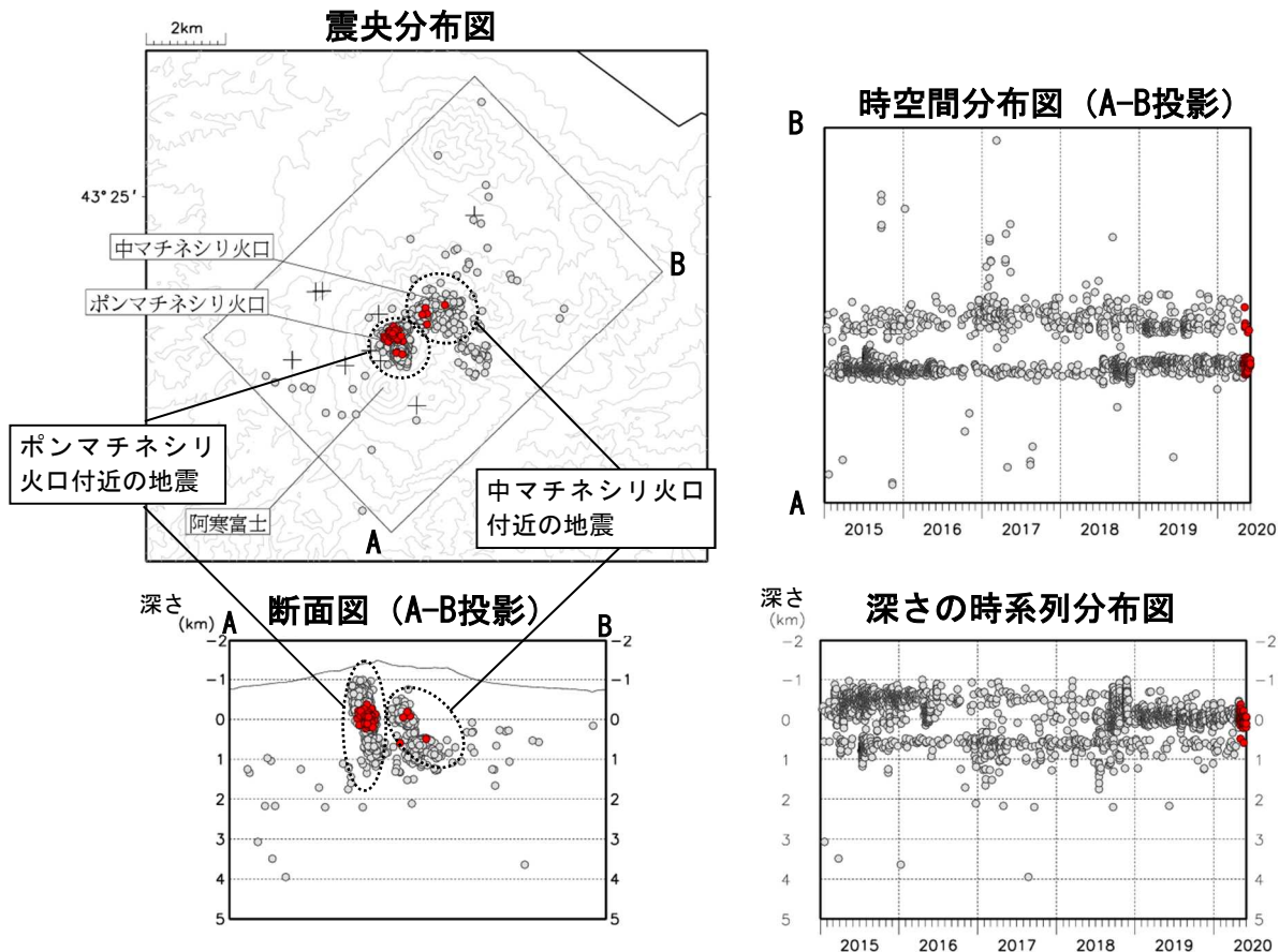
図6 雌阿寒岳 火山性地震の震源分布（2015年1月～2020年5月）
