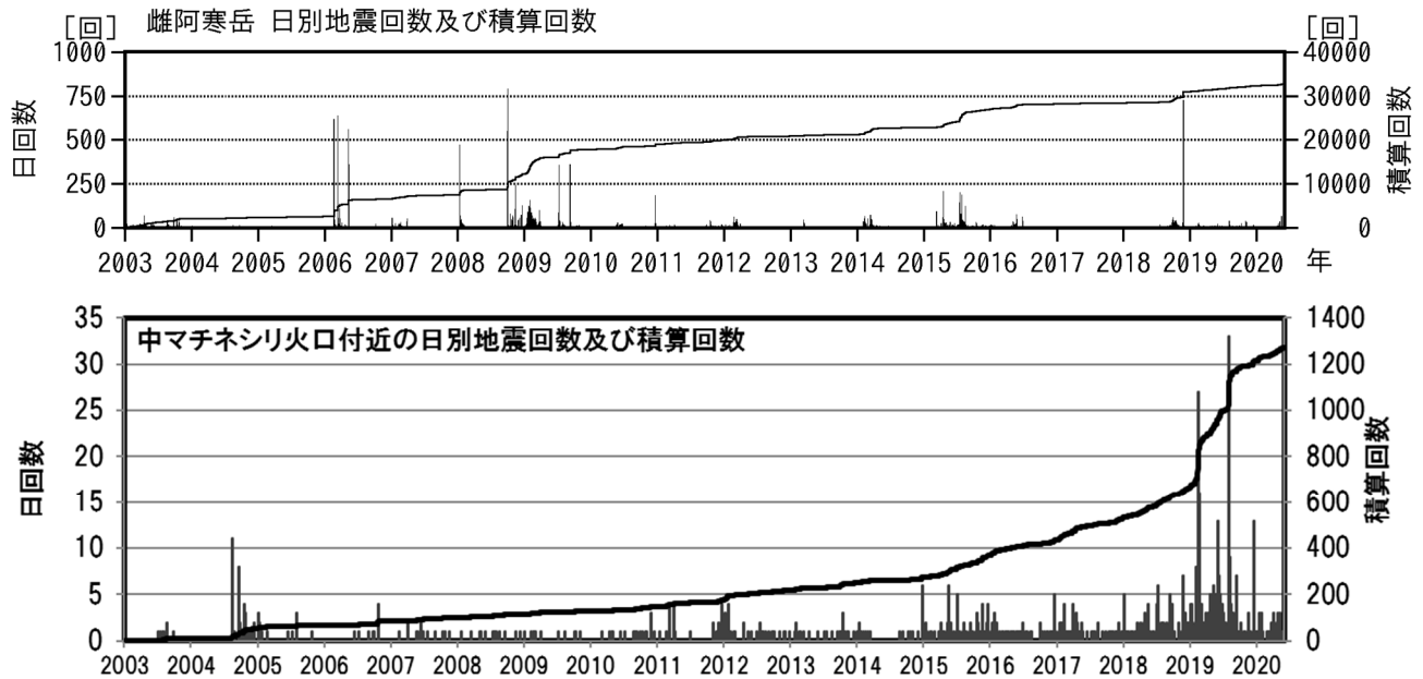
図5 雌阿寒岳 中マチネシリ火口付近の日別地震回数（2003年～2020年5月）
