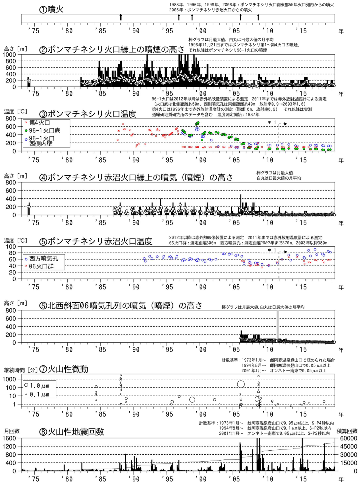
図1 雌阿寒岳 火山活動経過図（1973年1月～2020年5月）
