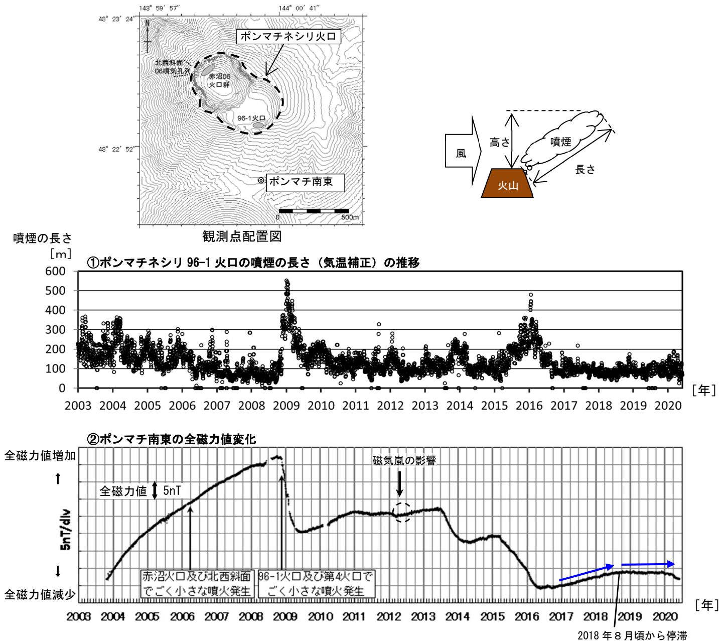
図4 雌阿寒岳 ポンマチネシリ96-1火口の噴煙の長さ（気温補正）の推移と全磁力の比較及び全磁力観測点配置図
