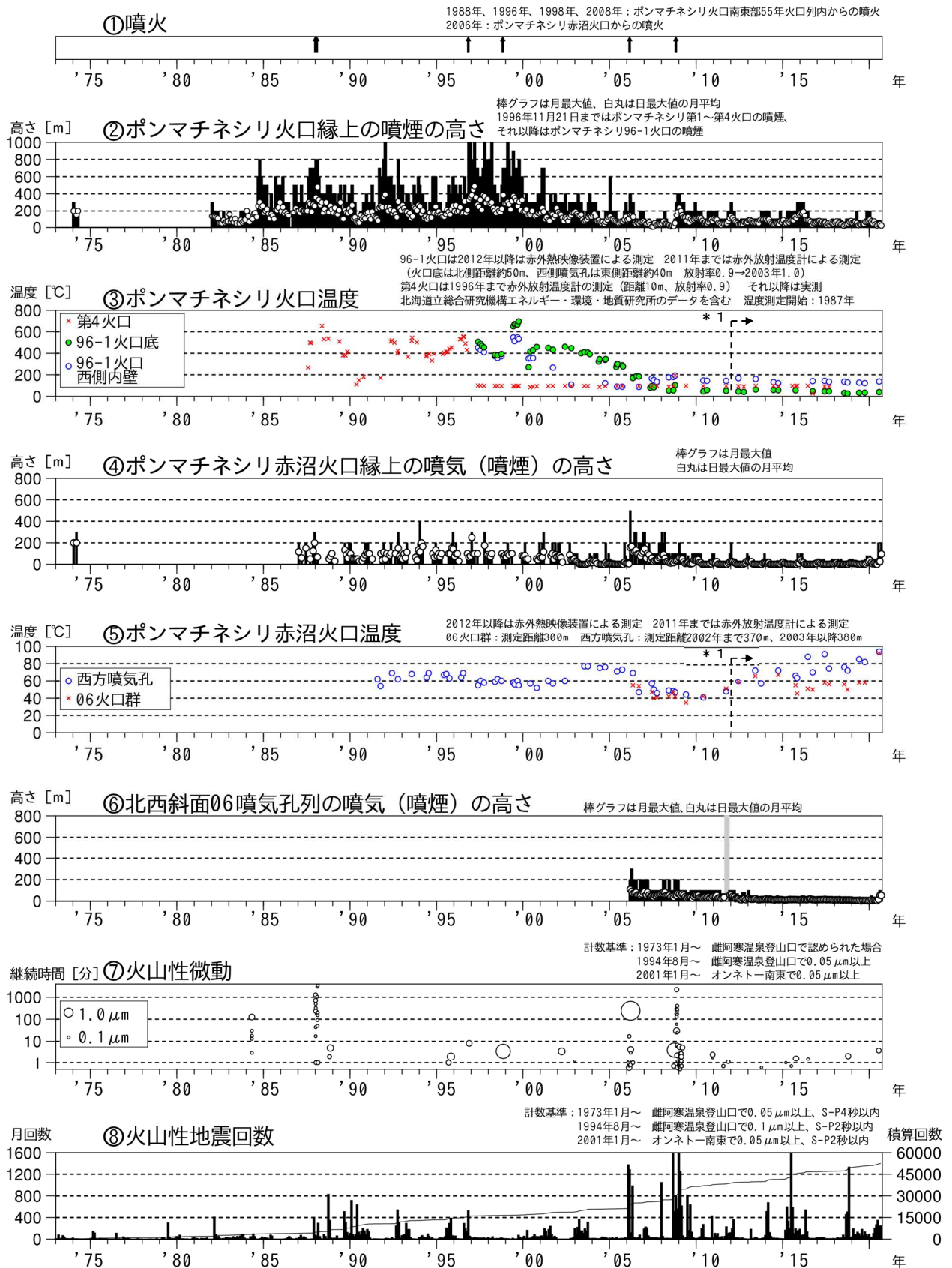
図1 雌阿寒岳 火山活動経過図（1973年1月～2020年9月）
