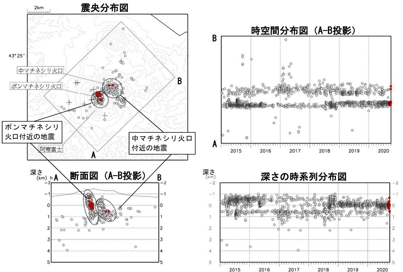
図7 雌阿寒岳 火山性地震の震源分布（2015年1月～2020年9月）
