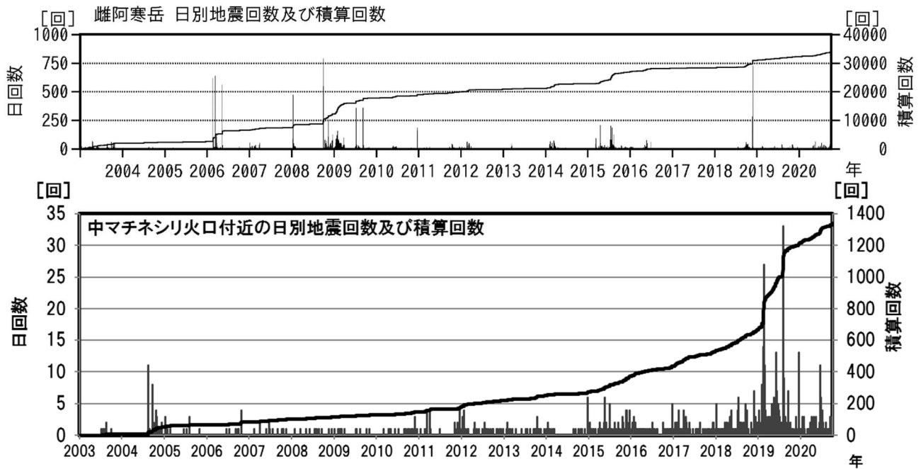
図6 雌阿寒岳 中マチネシリ火口付近の日別地震回数（2003年～2020年9月）
