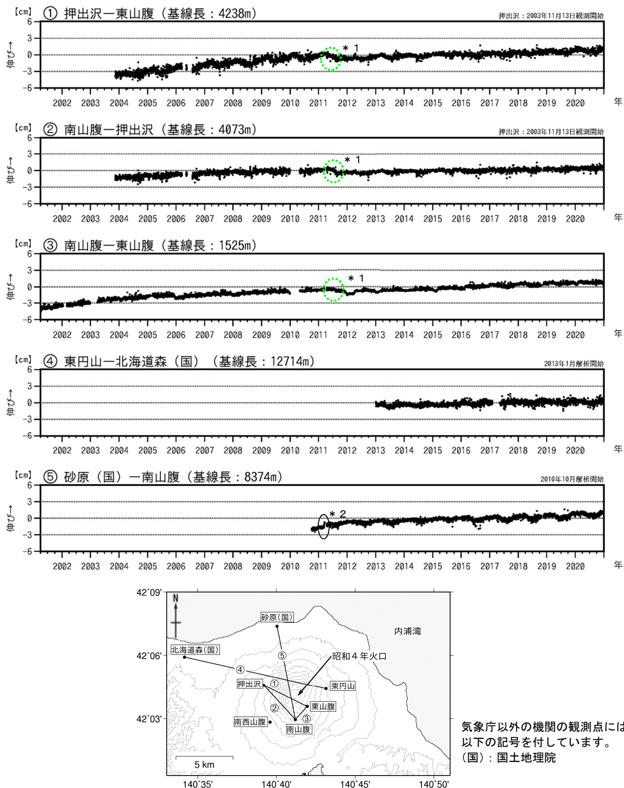
図5 北海道駒ヶ岳 GNSS連続観測による基線長変化（2001年4月～2020年12月）及び観測点配置図
