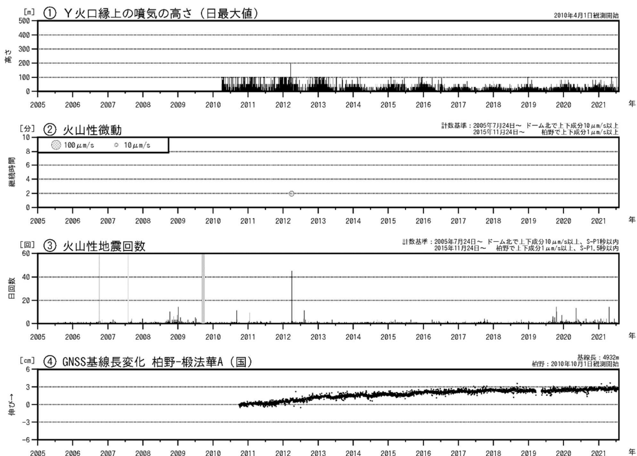
図2 恵山 火山活動経過図（2005年7月～2021年7月）
