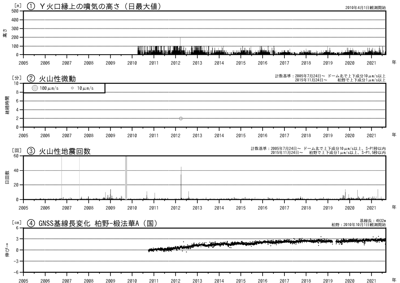
図2 恵山 火山活動経過図（2005年7月～2021年8月）
