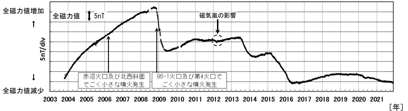
図6 雌阿寒岳 ポンマチネシリ96-1火口の噴煙の長さ（2003年～2021年11月）と全磁力の比較及び全磁力観測点配置図
