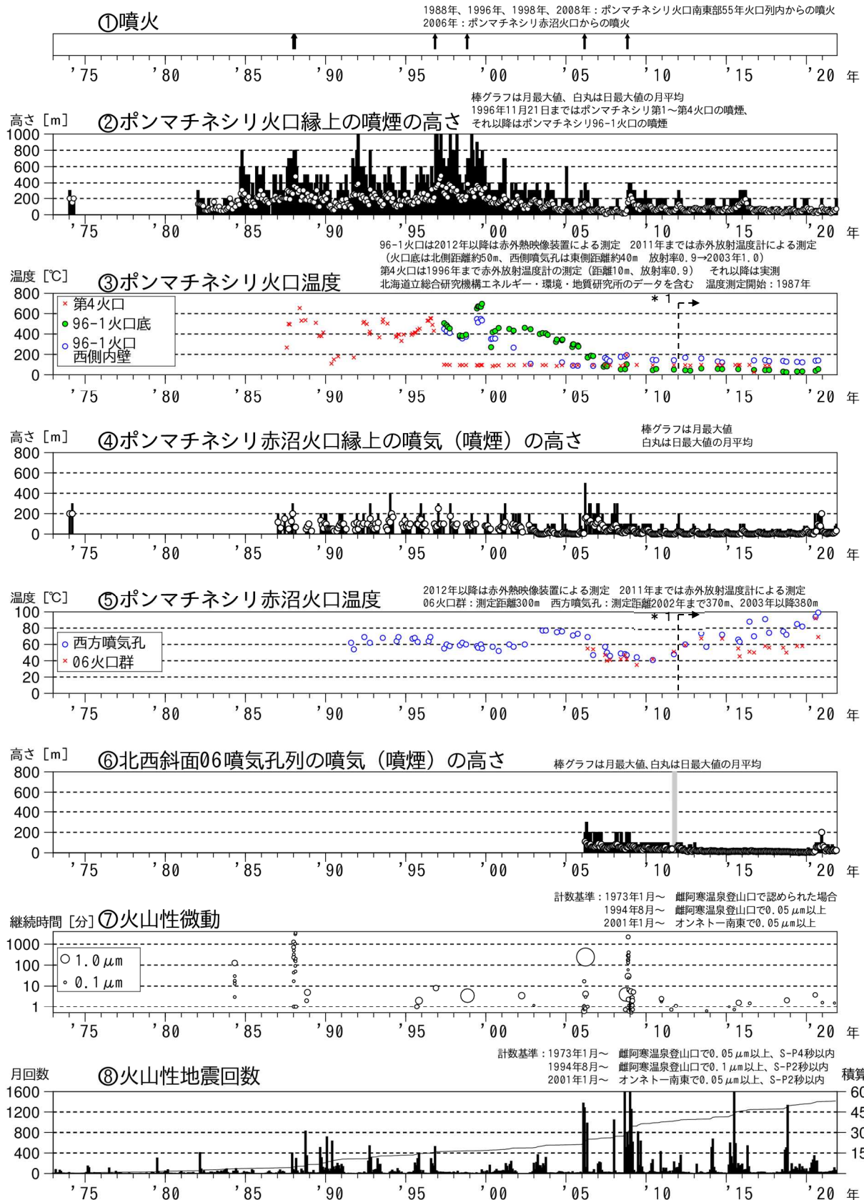
図1 雌阿寒岳 火山活動経過図（1973年1月～2021年11月）
