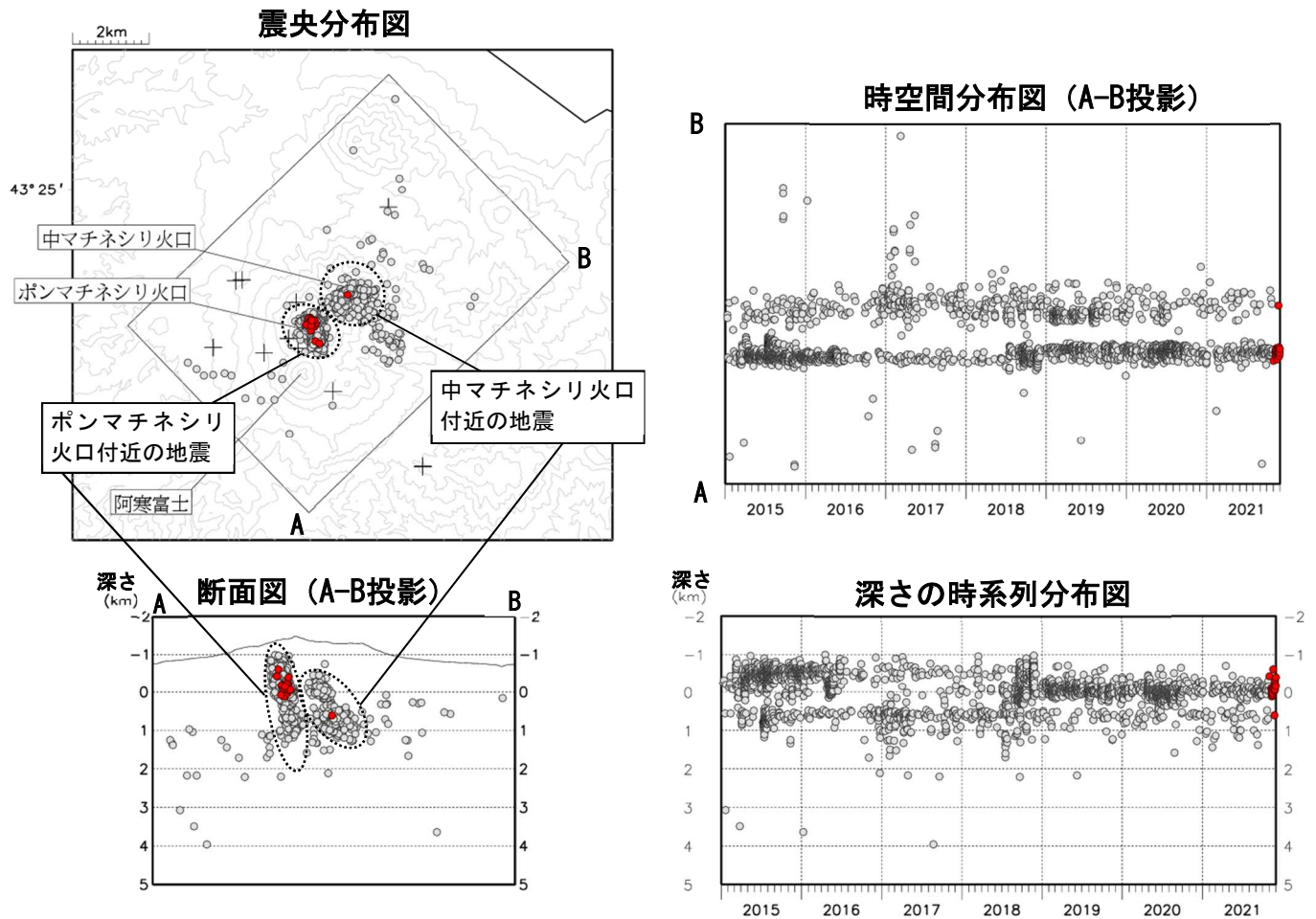
図7 雌阿寒岳 火山性地震の震源分布（2015年1月～2021年11月）
