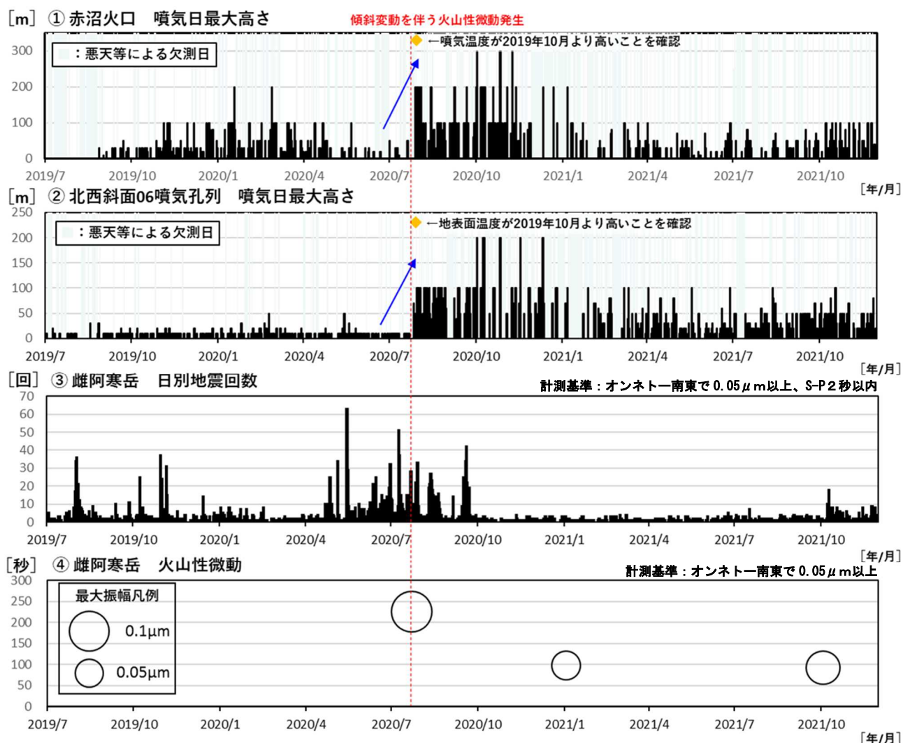
図5 雌阿寒岳 2020年7月の火山性微動以降の噴気活動及び地震活動等の活動経過
