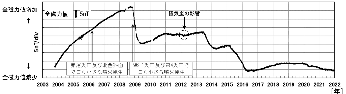
図6 雌阿寒岳 ポンマチネシリ96-1火口の噴煙の長さ と全磁力の比較及び全磁力観測点配置図
