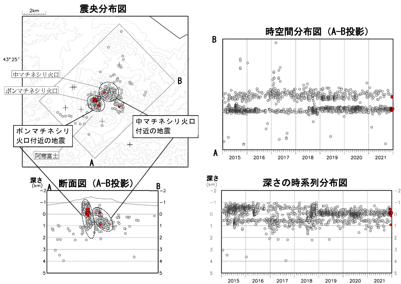
図7 雌阿寒岳 火山性地震の震源分布（2015年1月～2021年12月）
