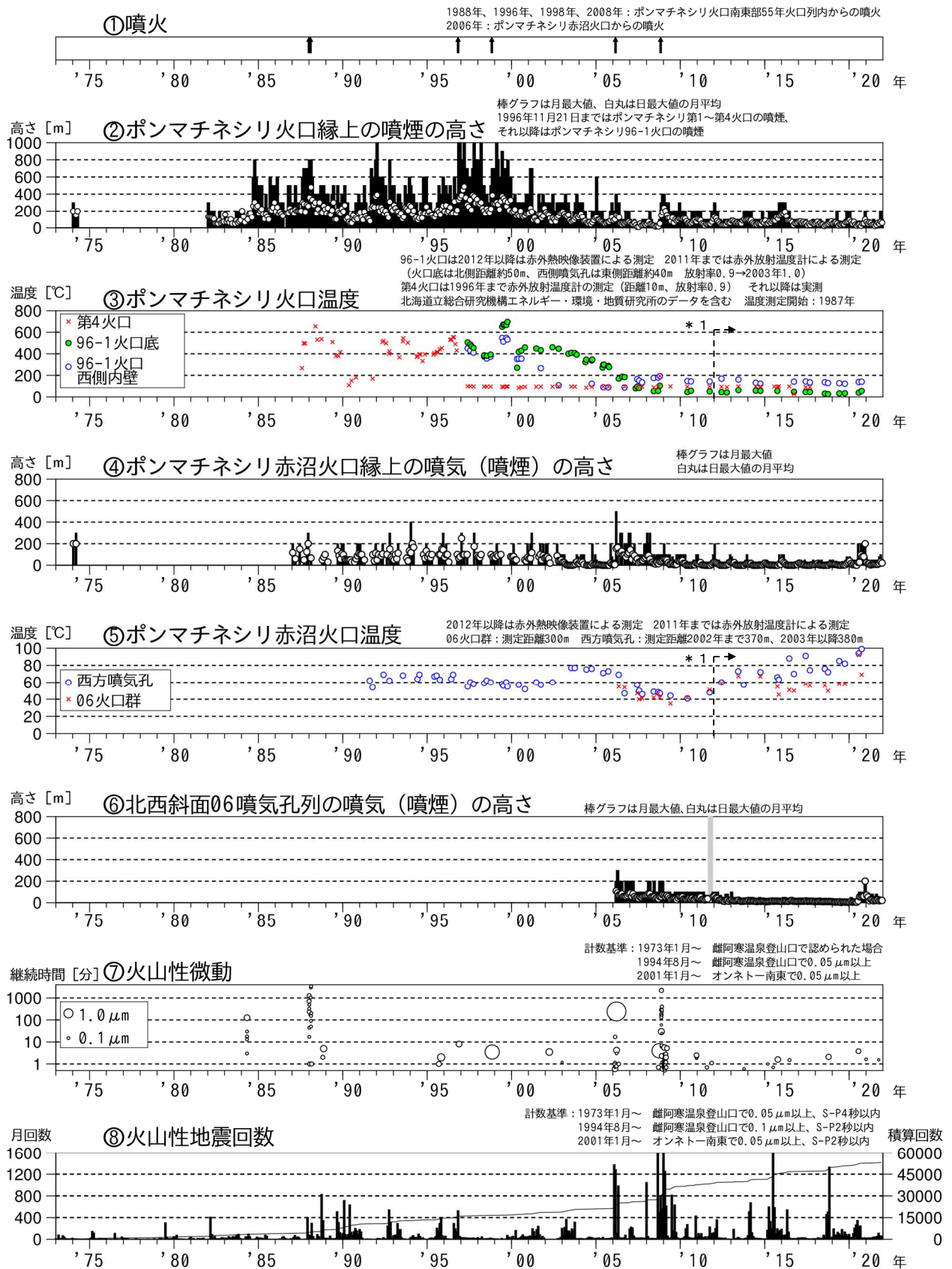
図1 雌阿寒岳 火山活動経過図（1973年1月～2021年12月）
