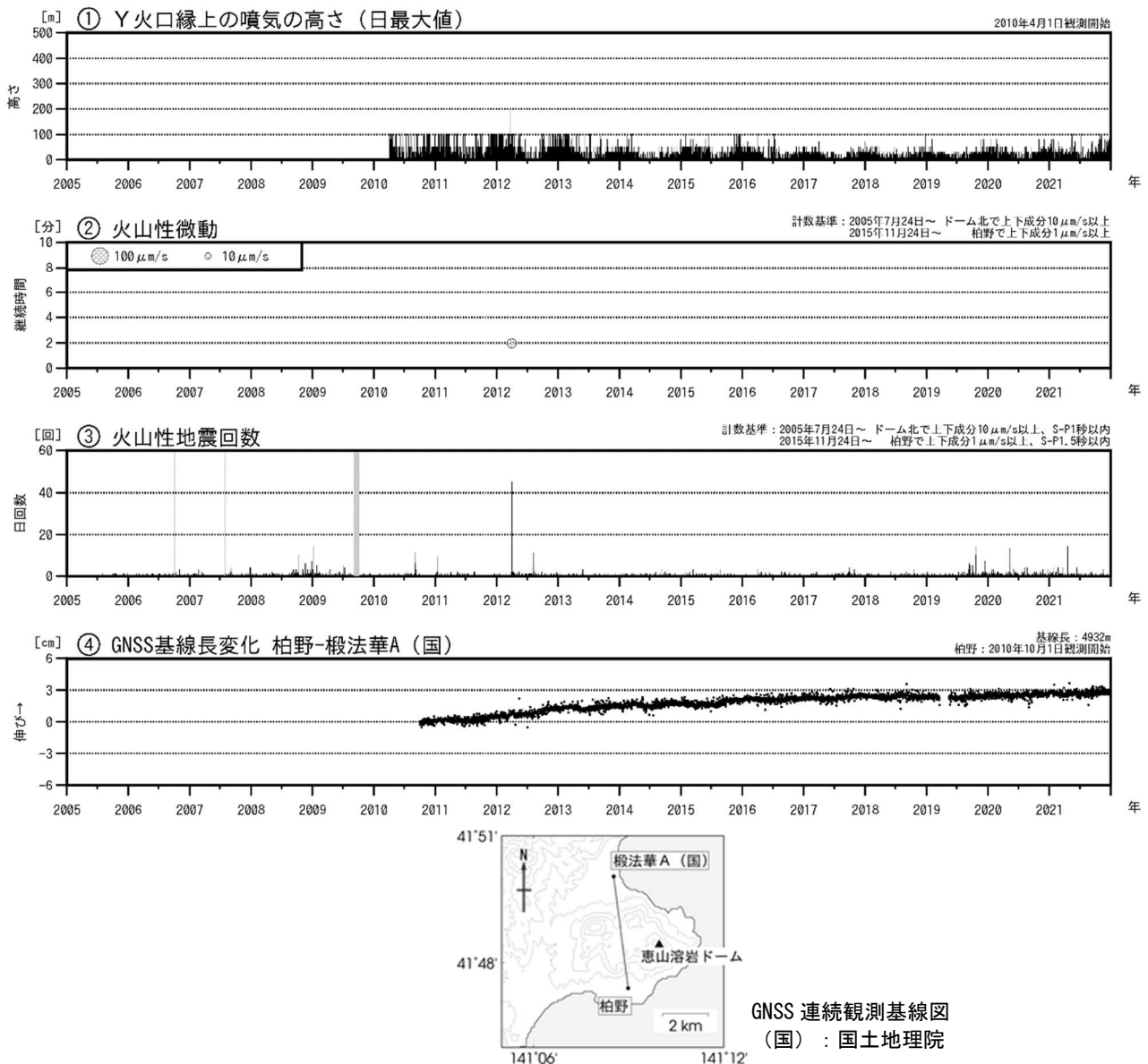
図2 恵山 火山活動経過図（2005年7月～2021年12月）
