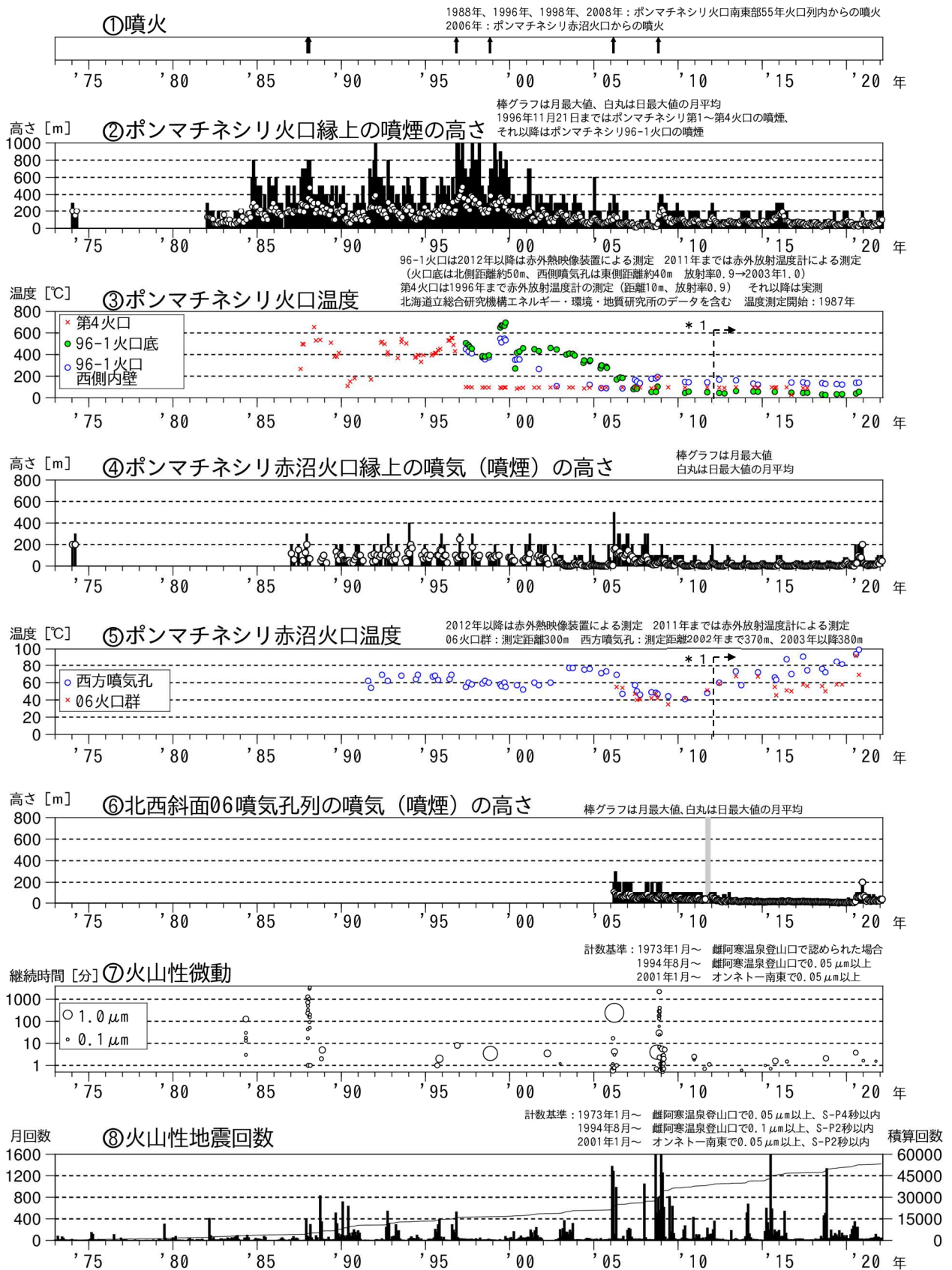
図1 雌阿寒岳 火山活動経過図（1973年1月～2022年2月）
