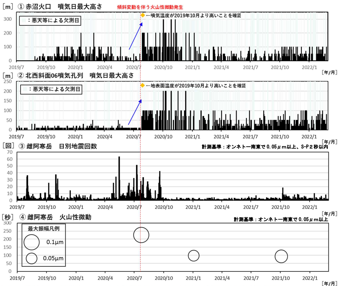
図5 雌阿寒岳 2020年7月の火山性微動以降の噴気活動及び地震活動等の活動経過
