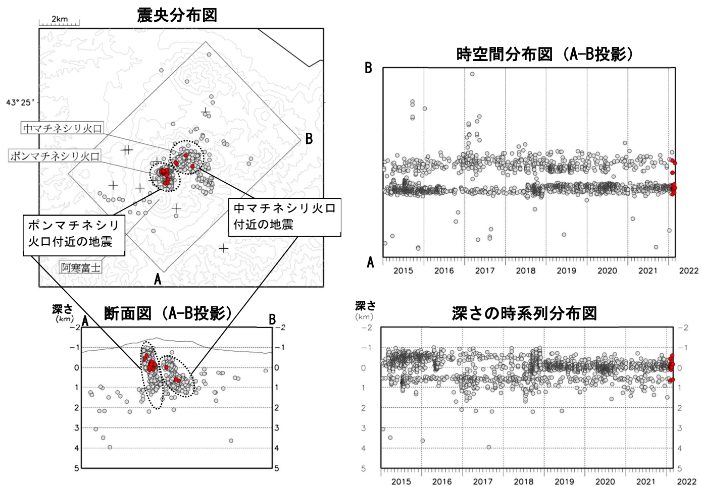
図7 雌阿寒岳 火山性地震の震源分布（2015年1月～2022年2月）
