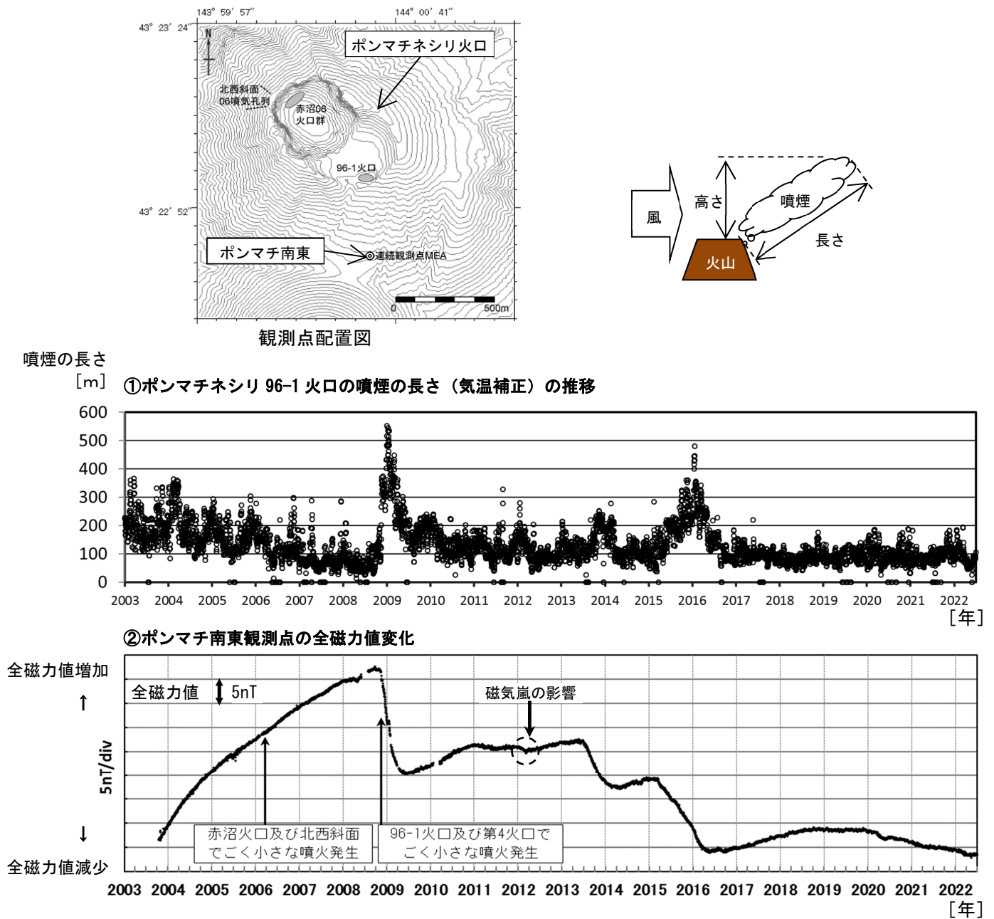
図5 雌阿寒岳 ポンマチネシリ96-1火口の噴煙の長さ と全磁力値の経過及び全磁力観測点配置図 (2003年～2022年6月)
