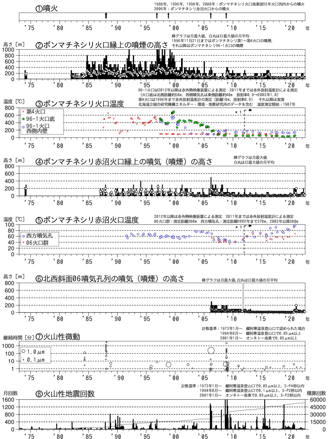
図1 雌阿寒岳 火山活動経過図（1973年1月～2022年6月）
