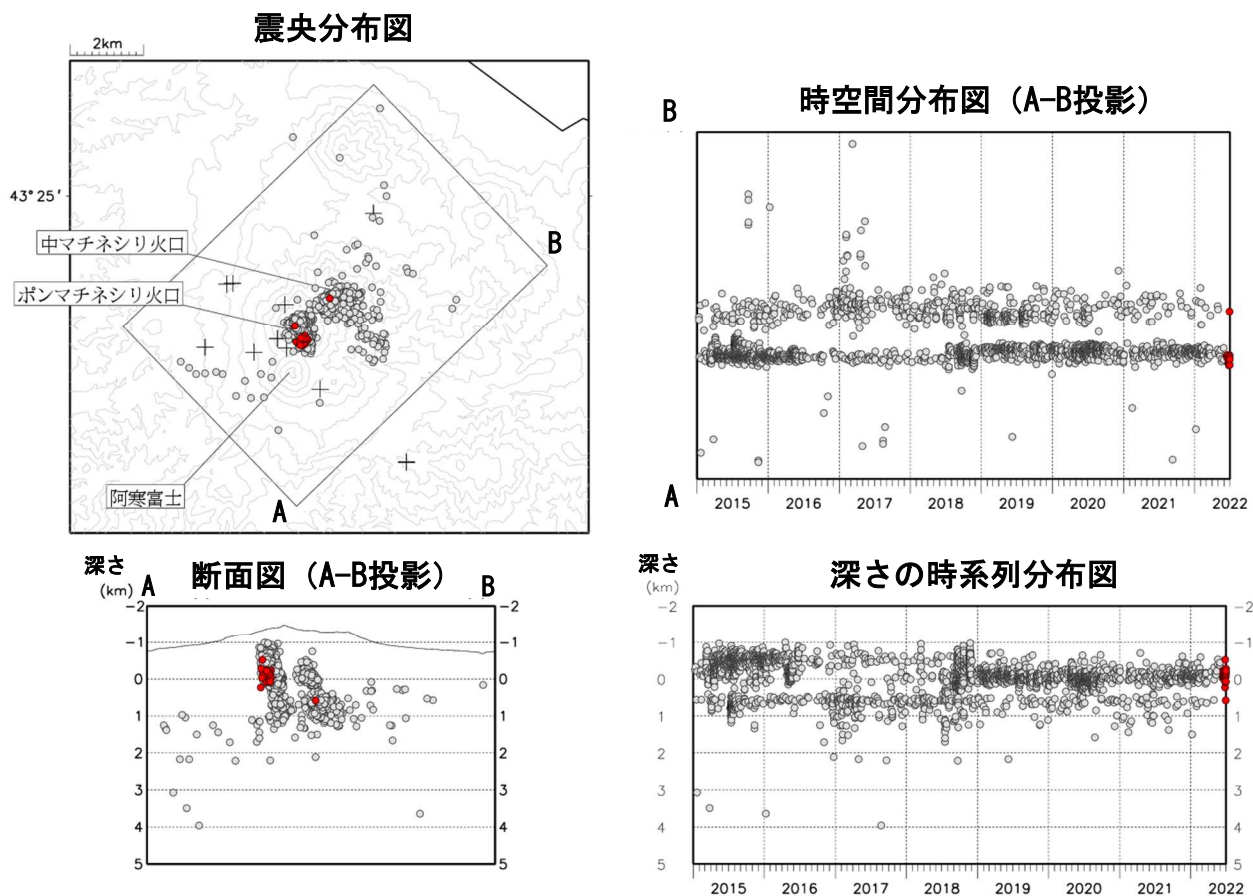
図6 雌阿寒岳 火山性地震の震源分布（2015年1月～2022年6月） ●印：2015年1月～2022年5月の震源 ●印：2022年6月の震源 +印：地震観測点
