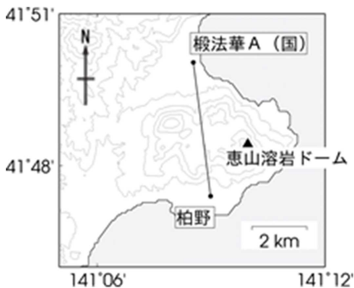
図2 恵山 火山活動経過図（2005年7月～2022年6月） ③の灰色部分は機器障害による欠測期間を示します。 ④のグラフは上図の基線に対応しています。 ④のグラフの空白部分は欠測を示します。
