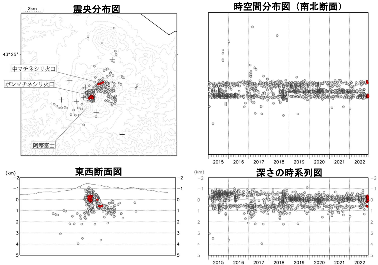
図5 雌阿寒岳 火山性地震の震源分布（2015年1月～2022年11月） ●：2015年1月～2022年10月の震源 ●：2022年11月の震源 ＋：地震観測点
