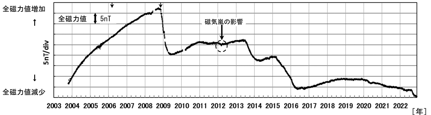
図4 雌阿寒岳 ポンマチネシリ96-1火口の噴煙の長さ と 全磁力値の経過及び全磁力観測点配置図 (2003年～2022年11月)
