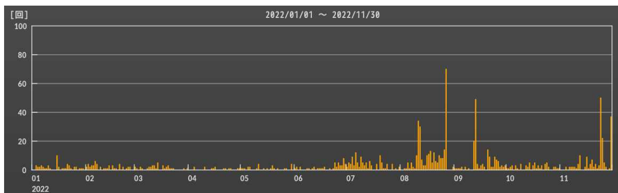
図6 雌阿寒岳 火山性地震の日別地震回数（2022年1月～2022年11月） ・24日に50回、25日に22回、30日に37回の地震をそれぞれ観測しました。 ・地震は主にポンマチネシリ火口付近で発生しました。
