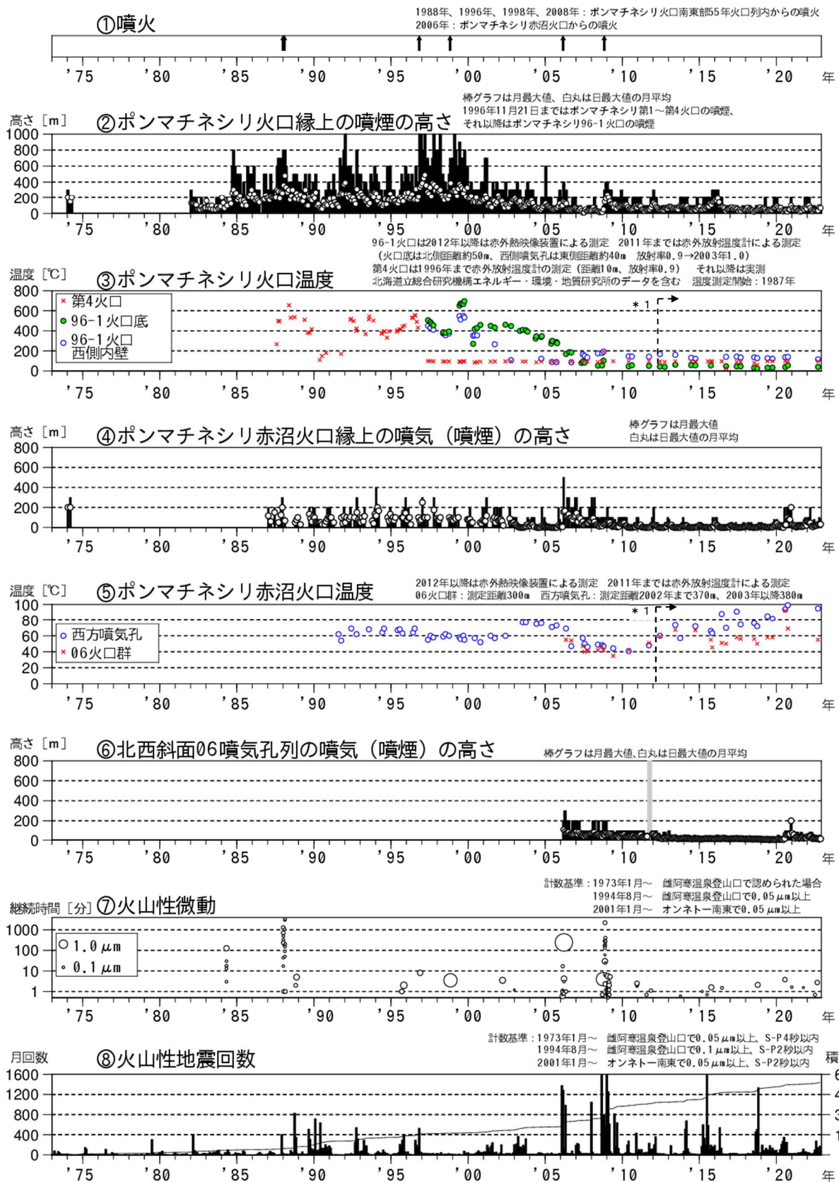
図1 雌阿寒岳 火山活動経過図（1973年1月～2022年11月）
