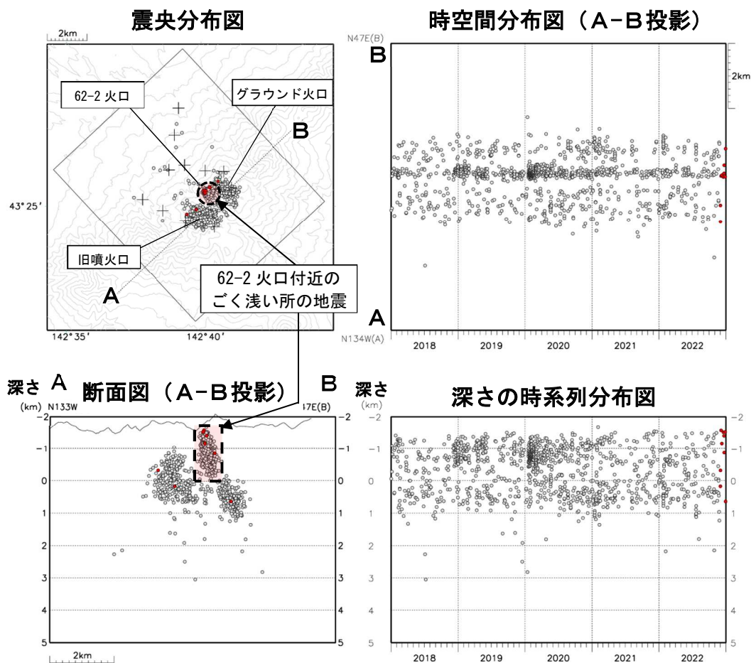
図4 十勝岳 火山性地震の震源分布（2018年1月～2022年12月） ●：2018年1月～2022年11月の震源 ●：2022年12月の震源 ＋：地震観測点
