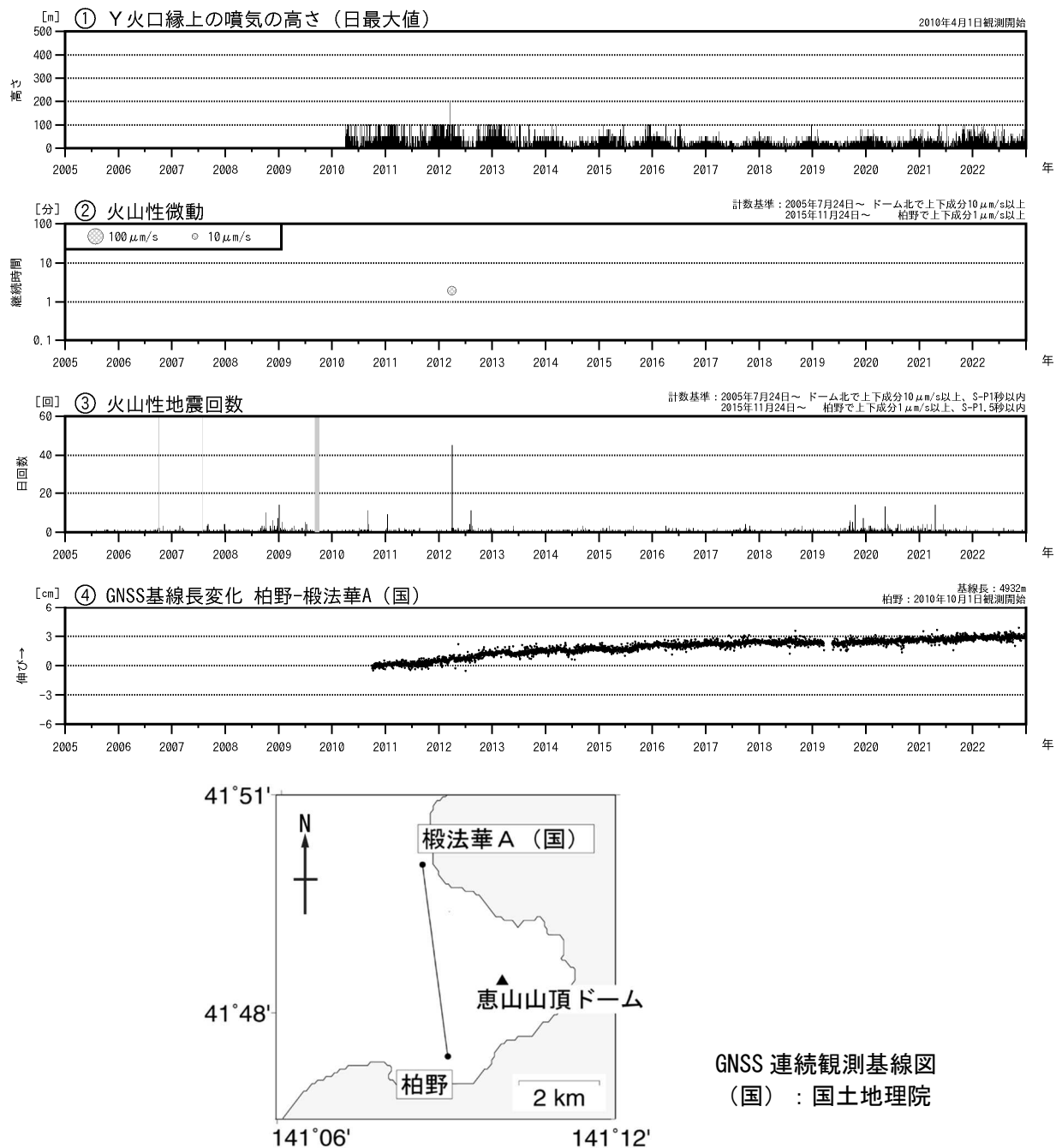
図2 恵山 火山活動経過図（2005年7月～2022年12月）
