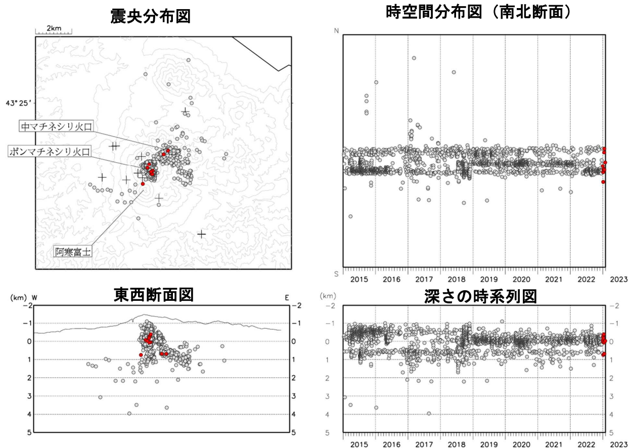
図5 雌阿寒岳 火山性地震の震源分布（2015年1月～2023年1月）
