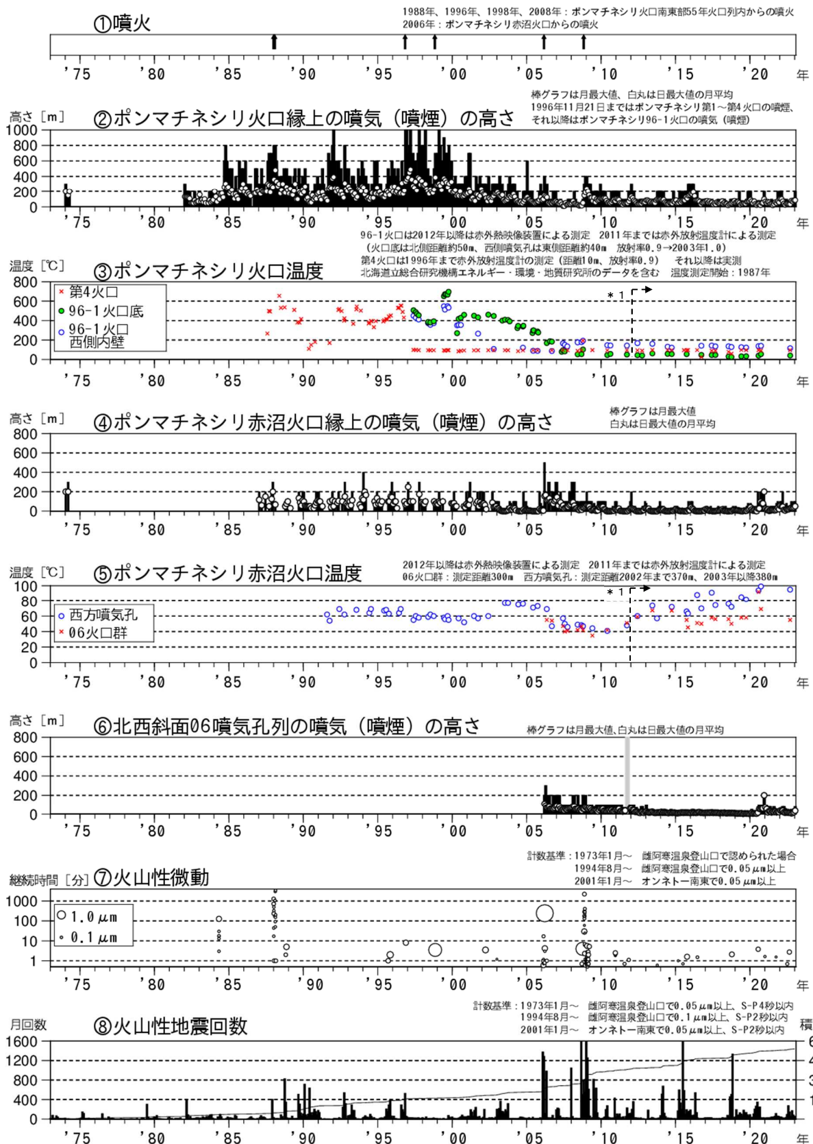
図1 雌阿寒岳 火山活動経過図（1973年1月～2023年1月）
