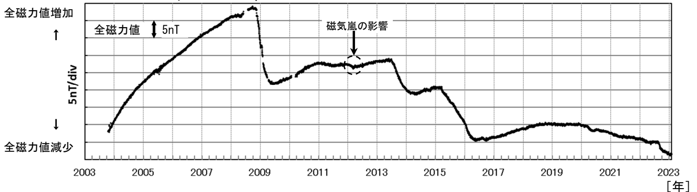
図4 雌阿寒岳 ポンマチネシリ96-1火口の噴気（噴煙）の長さとお磁力値の経過及び全磁力観測点配置図（2003年～2023年1月）
