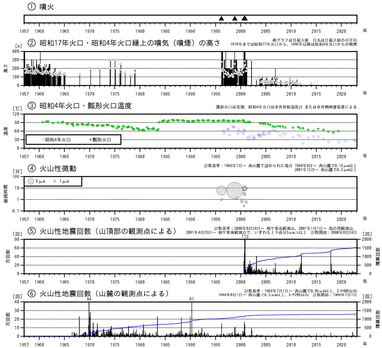
図1 北海道駒ヶ岳 火山活動経過図（1957年1月～2023年1月）
