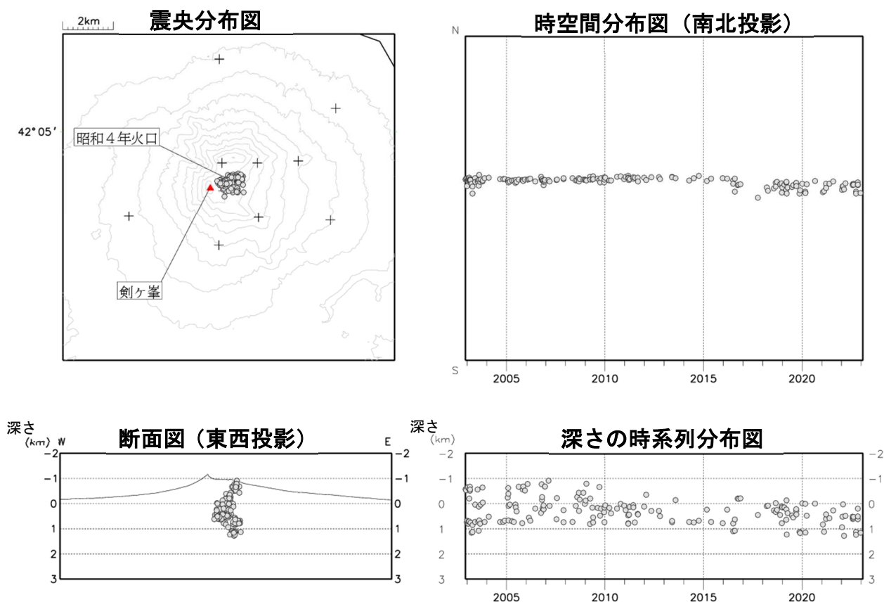
図4 北海道駒ヶ岳 火山性地震の震源分布（2002年12月～2023年1月）
