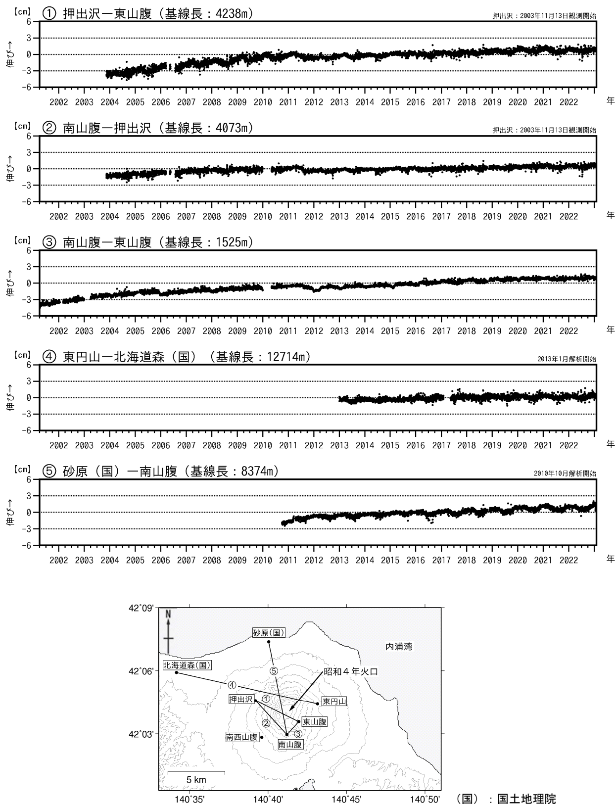
図5 北海道駒ヶ岳 GNSS連続観測による基線長変化（2001年4月～2023年1月）及び観測点配置図 グラフ①～⑤は観測点配置図の基線①～⑤に対応しています。 グラフの空白部分は欠測を示します。
