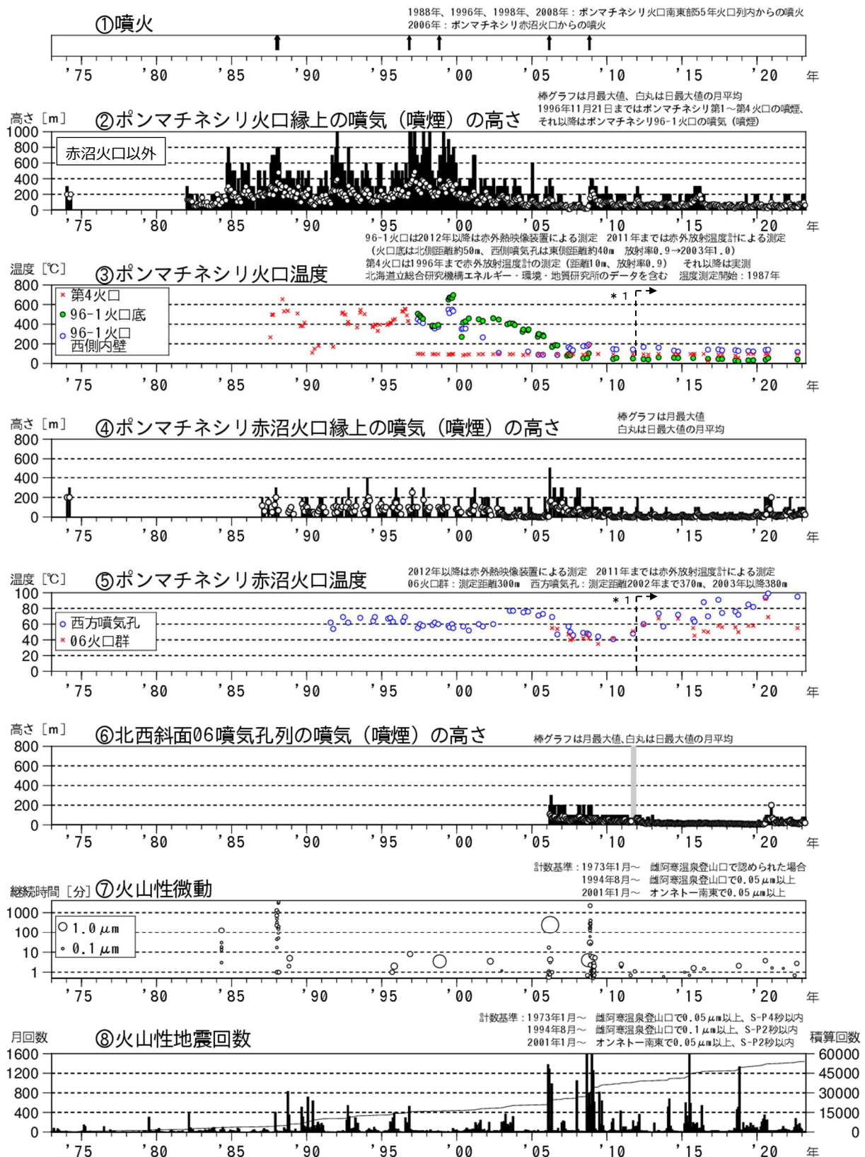
図1 雌阿寒岳 火山活動経過図（1973年1月～2023年3月）
