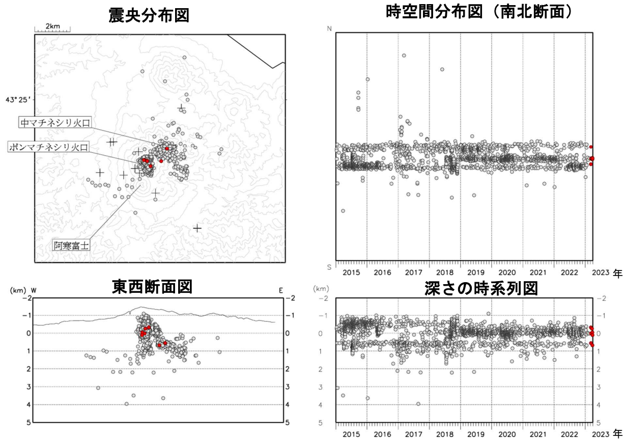
図5 雌阿寒岳 火山性地震の震源分布（2015年1月～2023年3月）
