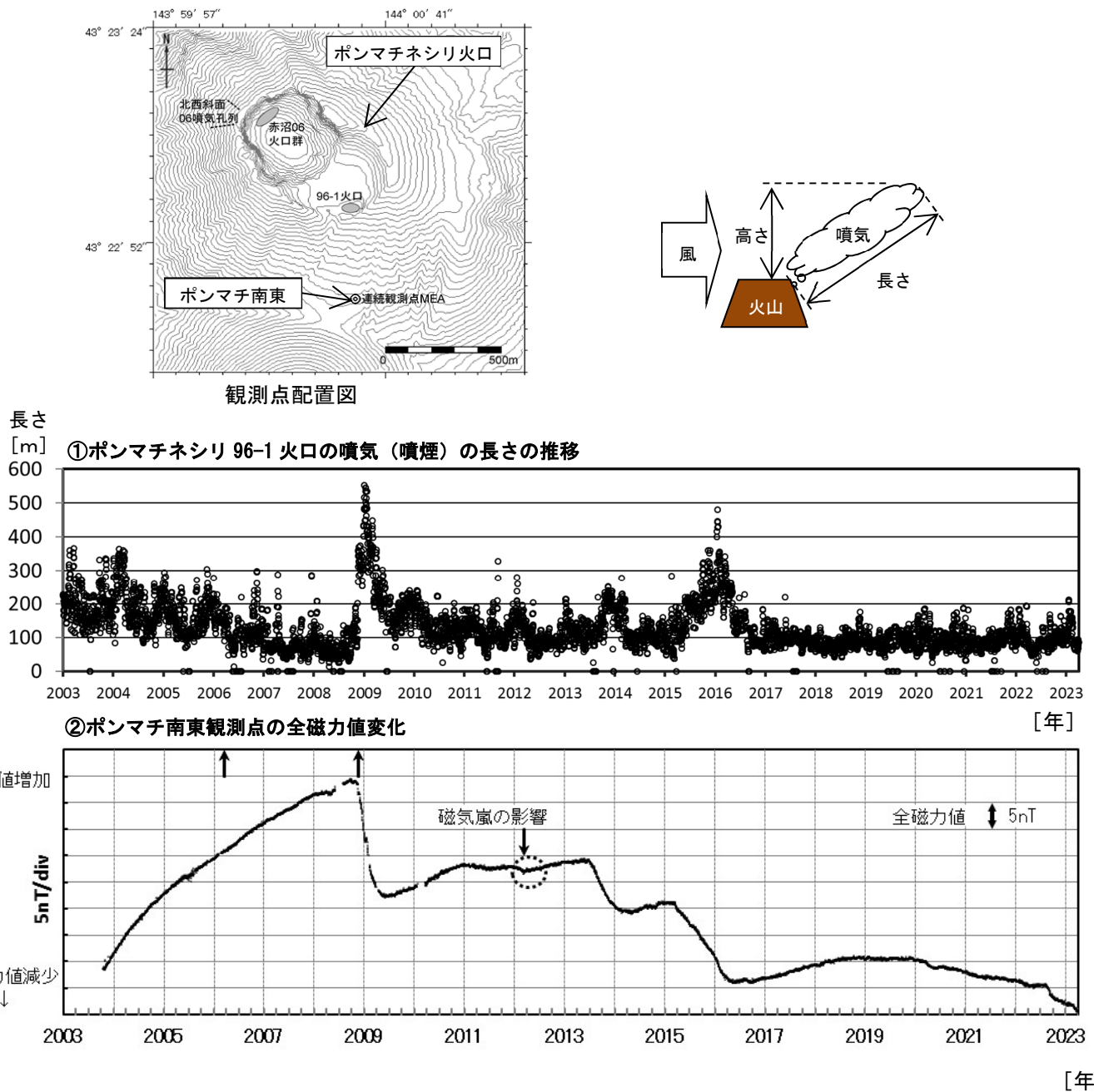
図4 雌阿寒岳 ポンマチネシリ96-1火口の噴気（噴煙）の長さ、全磁力値の経過及び全磁力観測点配置図（2003年～2023年3月）
