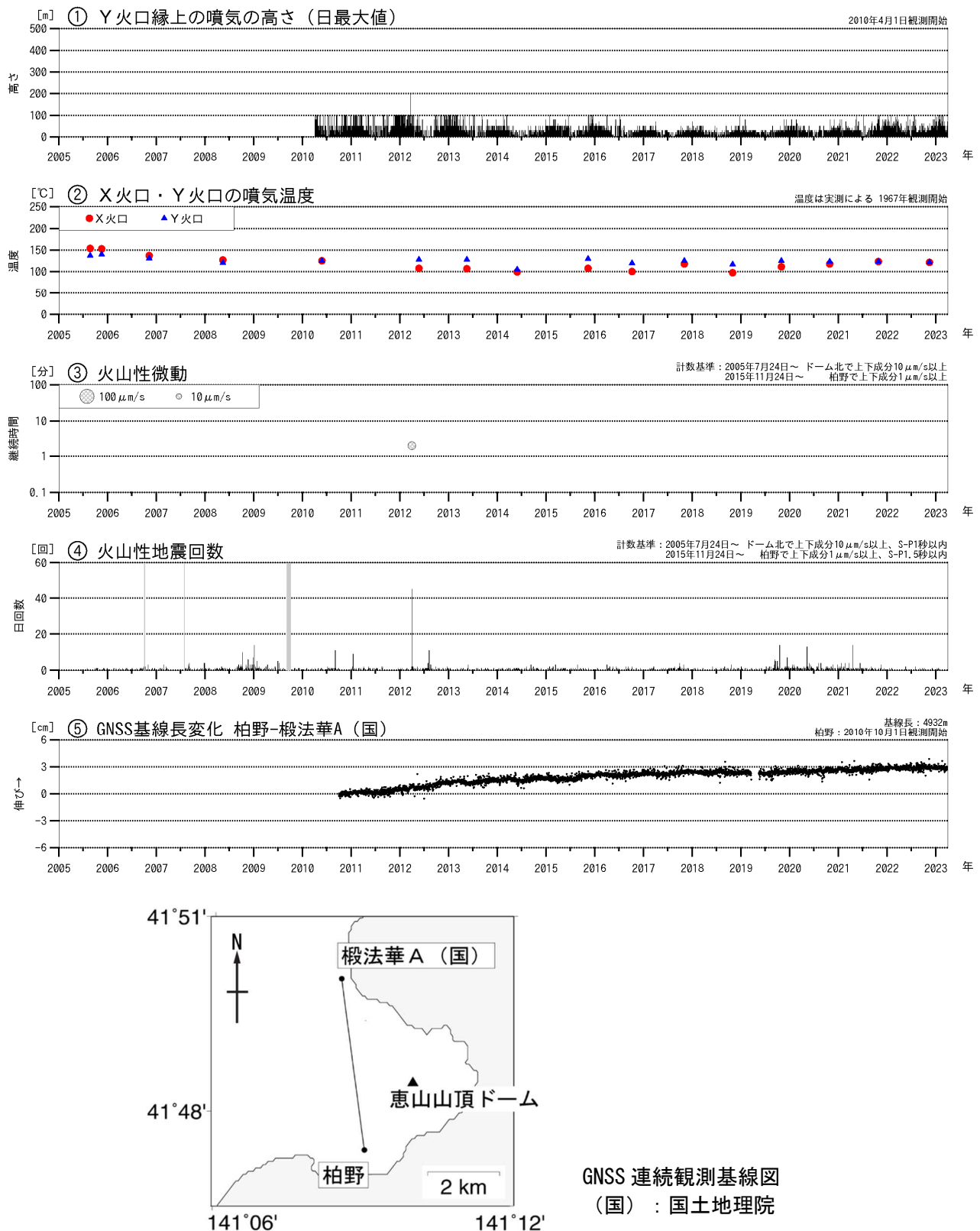
図2 恵山 火山活動経過図（2005年7月～2023年3月） ③の灰色部分は機器障害による欠測期間を示します。 ④のグラフは上図の基線に対応しています。 ④のグラフの空白部分は欠測を示します。
