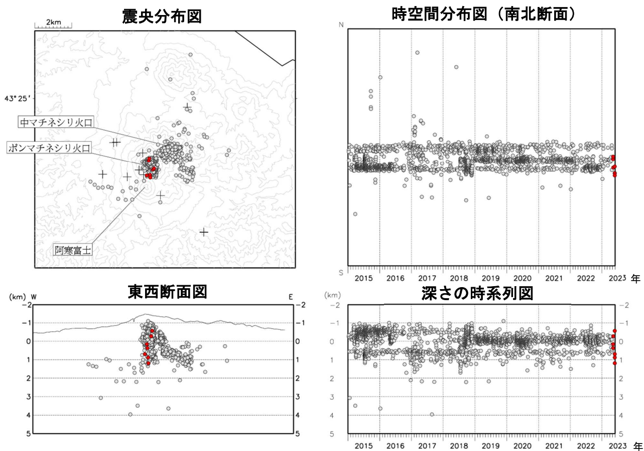
図5 雌阿寒岳 火山性地震の震源分布（2015年1月～2023年5月）
