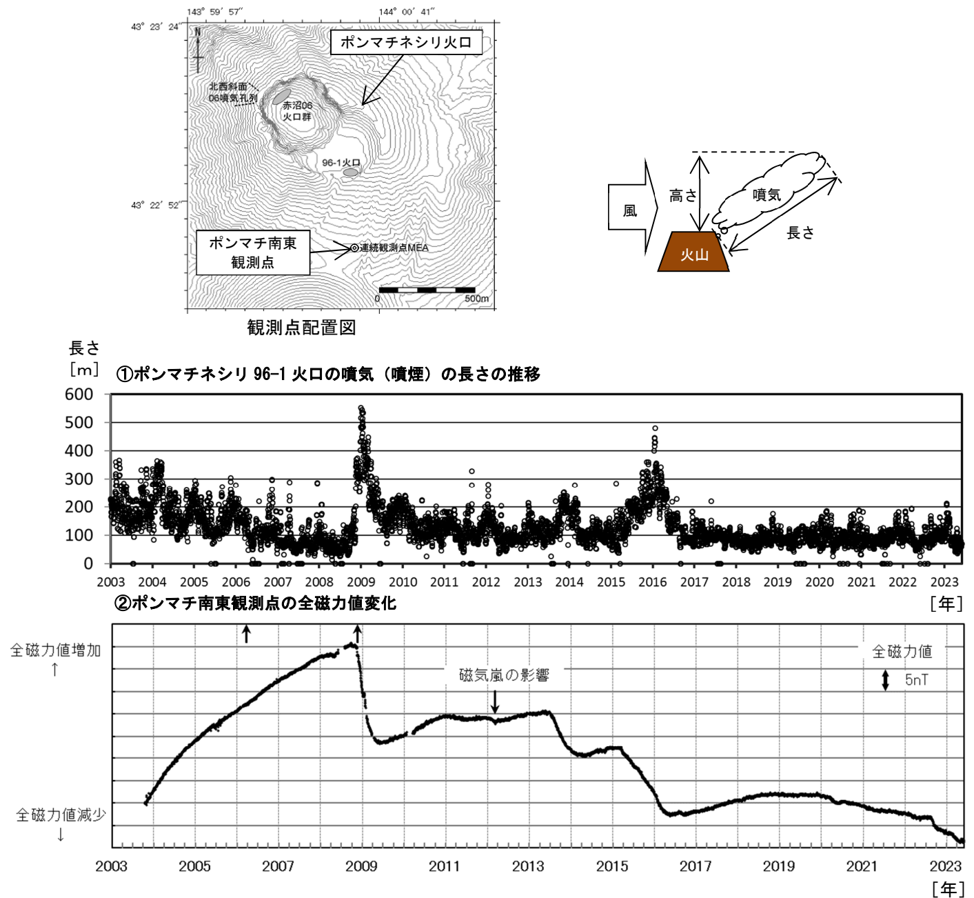
図4 雌阿寒岳 ポンマチネシリ96-1火口の噴気（噴煙）の長さ、全磁力値の経過及び全磁力観測点配置図（2003年～2023年5月）
