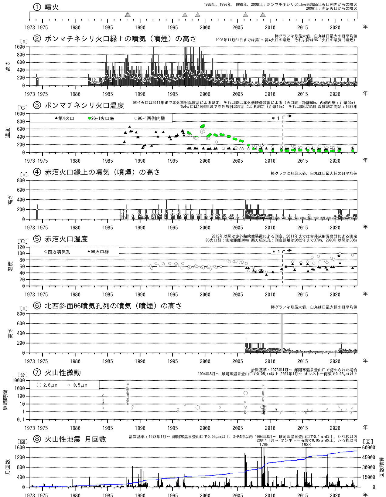
図1 雌阿寒岳 火山活動経過図（1973年1月～2023年5月）
