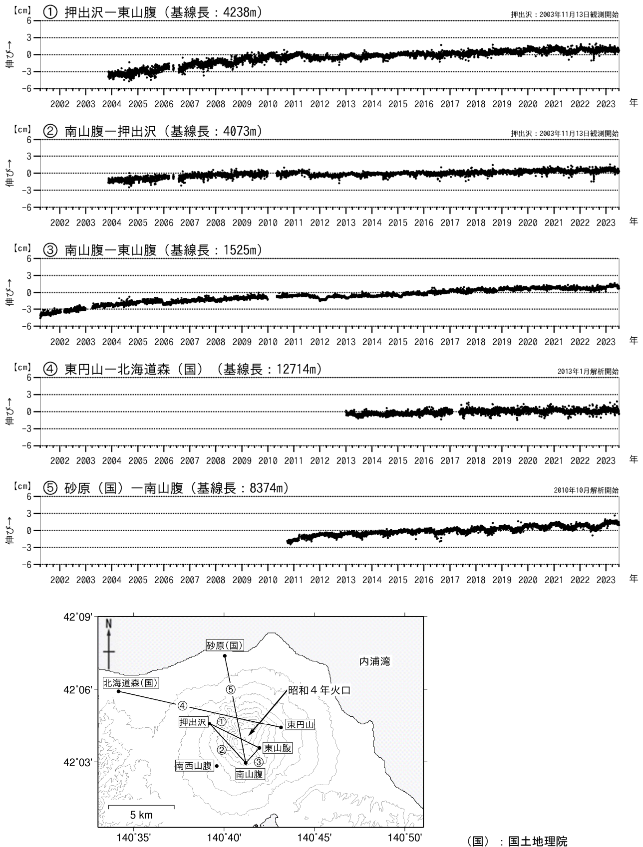
図5 北海道駒ヶ岳 GNSS連続観測による基線長変化（2001年4月～2023年6月）及び観測点配置図 グラフ①～⑤は観測点配置図の基線①～⑤に対応しています。 グラフの空白部分は欠測を示します。
