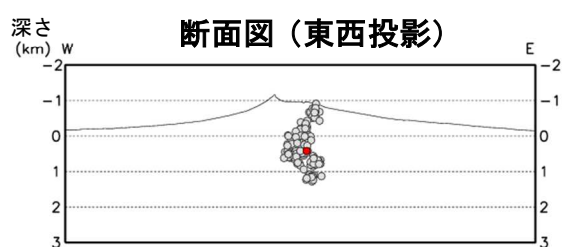
図4 北海道駒ヶ岳 火山性地震の震源分布（2002年12月～2023年6月）
