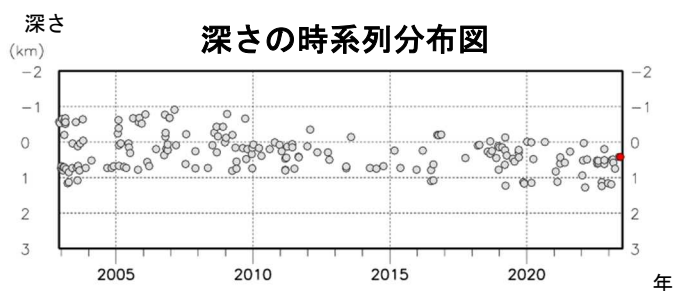
図4 北海道駒ヶ岳 火山性地震の震源分布（2002年12月～2023年6月）
