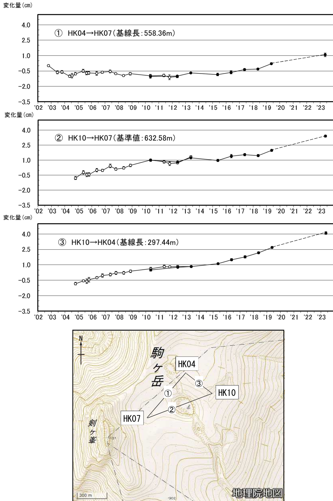
図6 北海道駒ヶ岳 GNSS繰り返し観測による火口付近の基線長変化（2002年4月～2023年6月）及び観測点配置図
