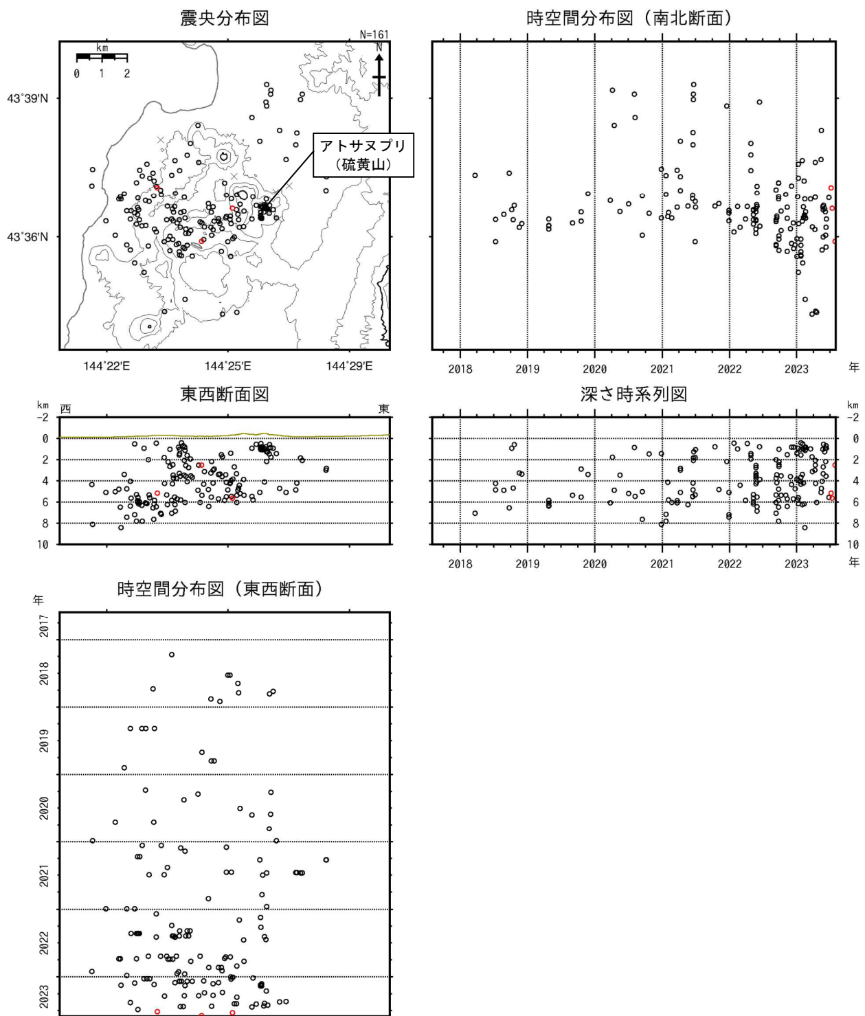
図3 アトサヌプリ 火山性地震の震源分布（2017年8月～2023年7月）
