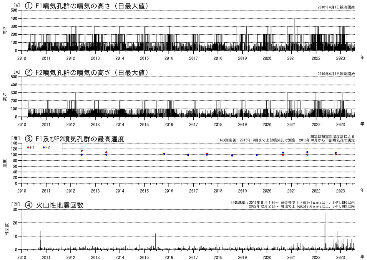
図1 アトサヌプリ 火山活動経過図（2010年4月～2023年7月）
