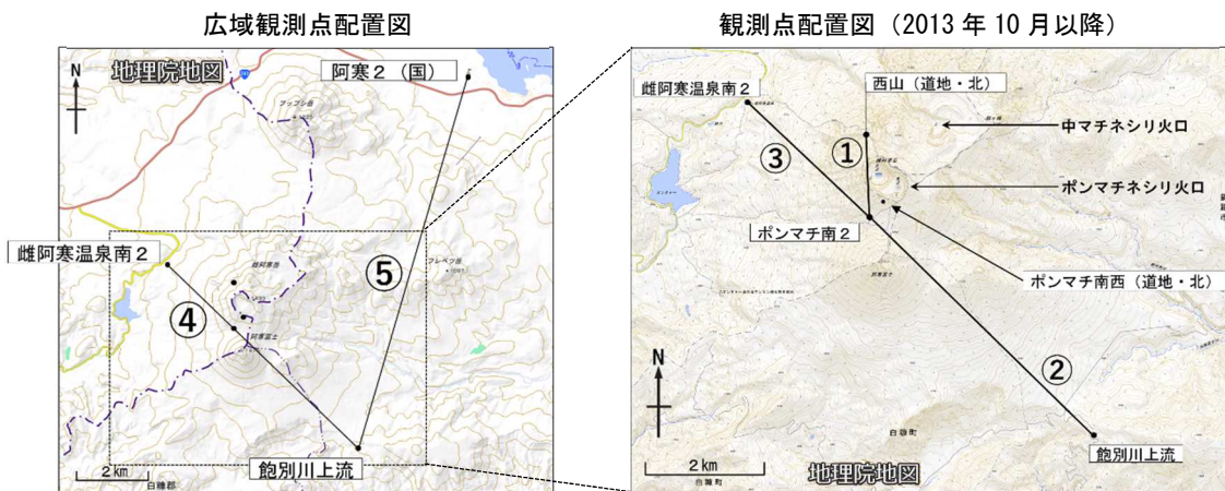
図9 雌阿寒岳 GNSS連続観測による基線長変化(2006年4月～2023年7月)及び観測点配置図
