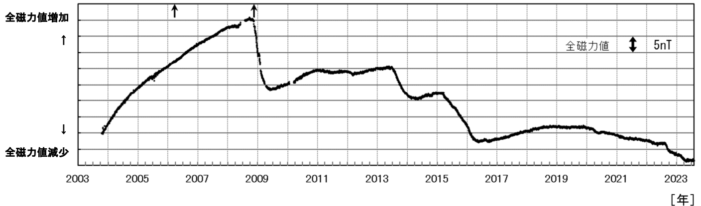
図4 雌阿寒岳 ポンマチネシリ96-1火口の噴気（噴煙）の長さや全磁力値の経過及び全磁力観測点配置図（2003年～2023年7月）
