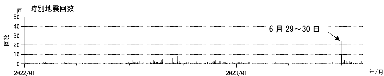
図8 雌阿寒岳 火山性地震の特別回数（2022年1月～2023年7月） ・ 6月29～30日に特別地震回数が20回を超える一時的な増加があり、7月以降の地震回数は地震増加以前に比べるとわずかに多い状態が続いています。
