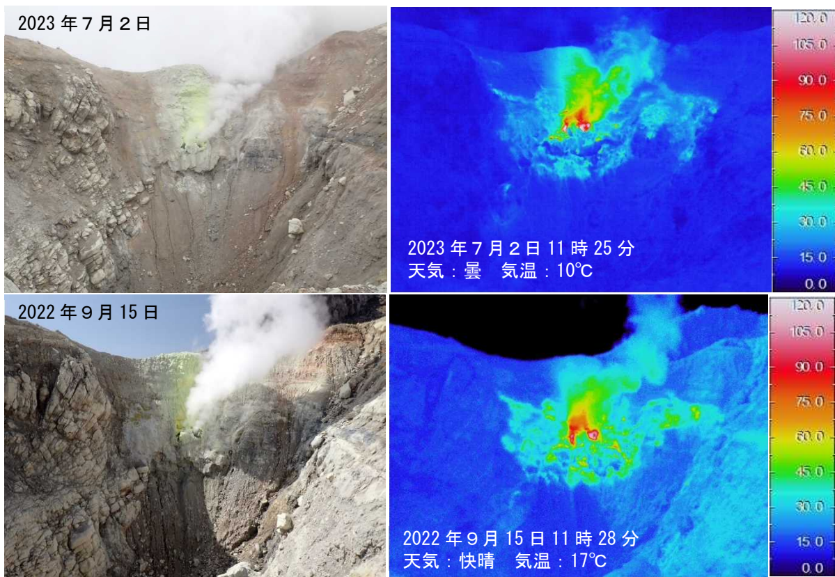
図5 雌阿寒岳 赤外熱映像装置によるポンマチネシリ96-1火口内西壁の地表面温度分布 (図11の①から撮影)
