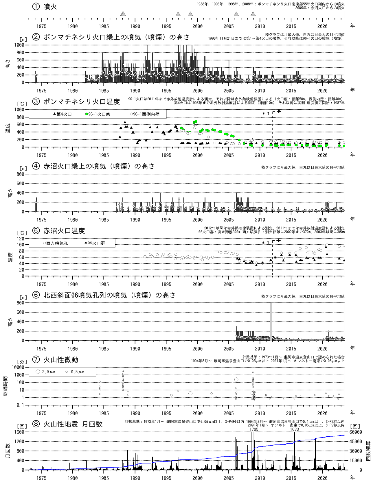
図1 雌阿寒岳 火山活動経過図（1973年1月～2023年7月）
