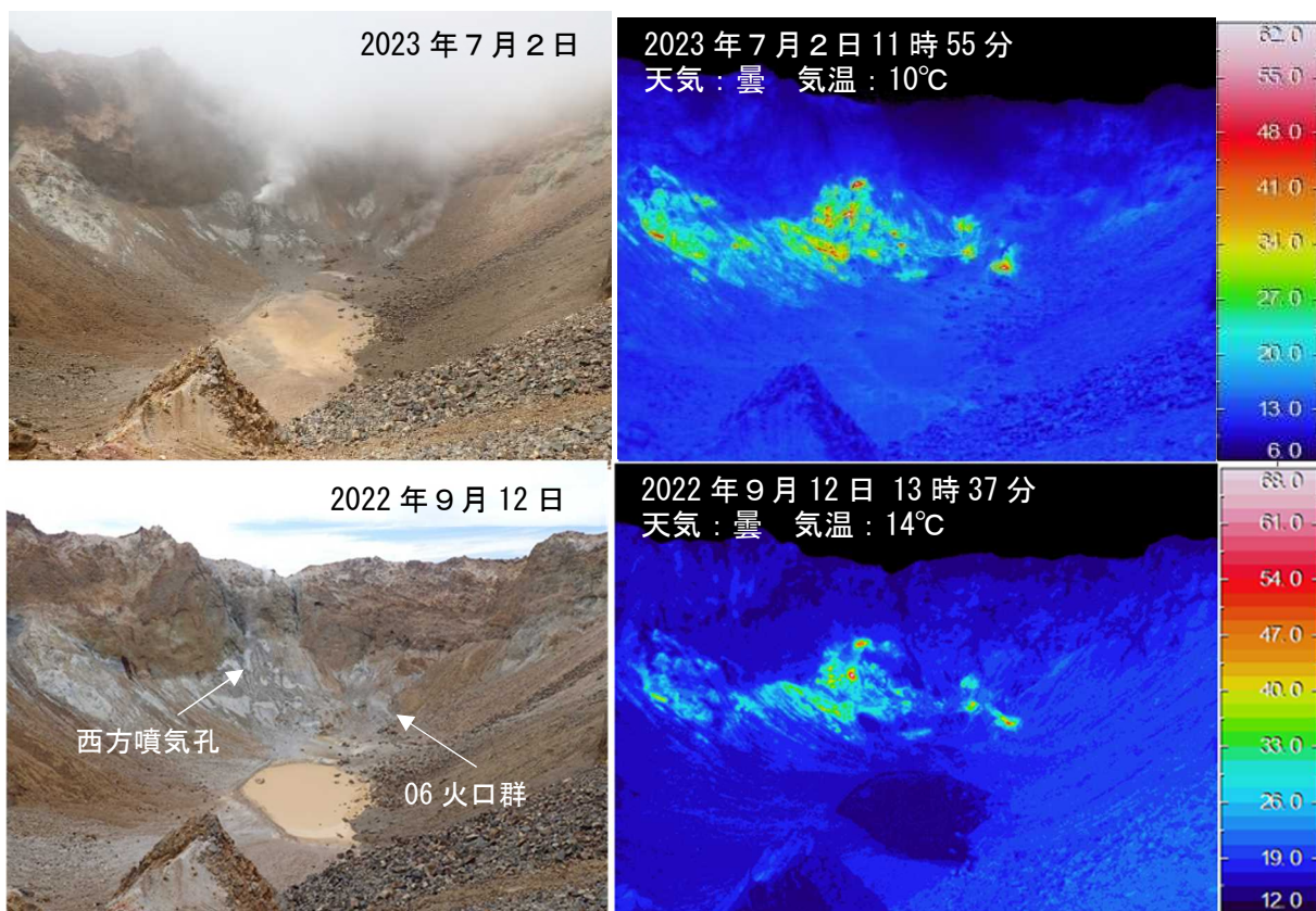
図6 雌阿寒岳 赤外熱映像装置によるポンマチネシリ赤沼火口内の地表面温度分布 (図11の②から撮影)
