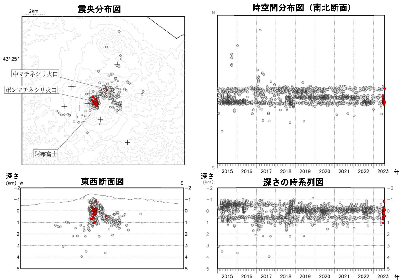
図7 雌阿寒岳 火山性地震の震源分布（2015年1月～2023年7月） ●：2015年1月～2023年6月の震源 ●：2023年7月の震源 ＋：地震観測点
