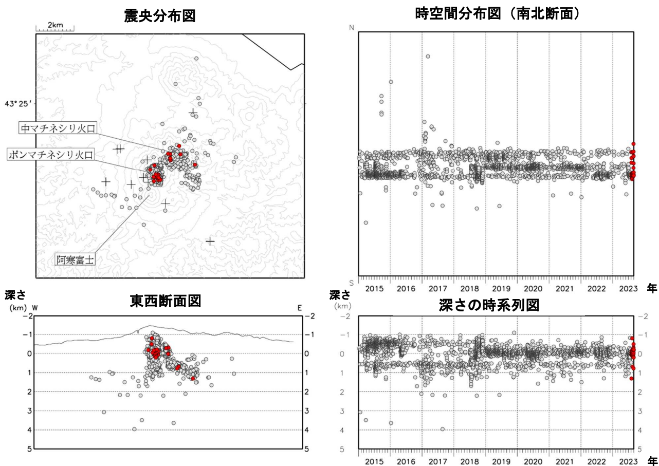
図5 雌阿寒岳 火山性地震の震源分布（2015年1月～2023年8月） ●：2015年1月～2023年7月の震源 ●：2023年8月の震源 +：地震観測点
