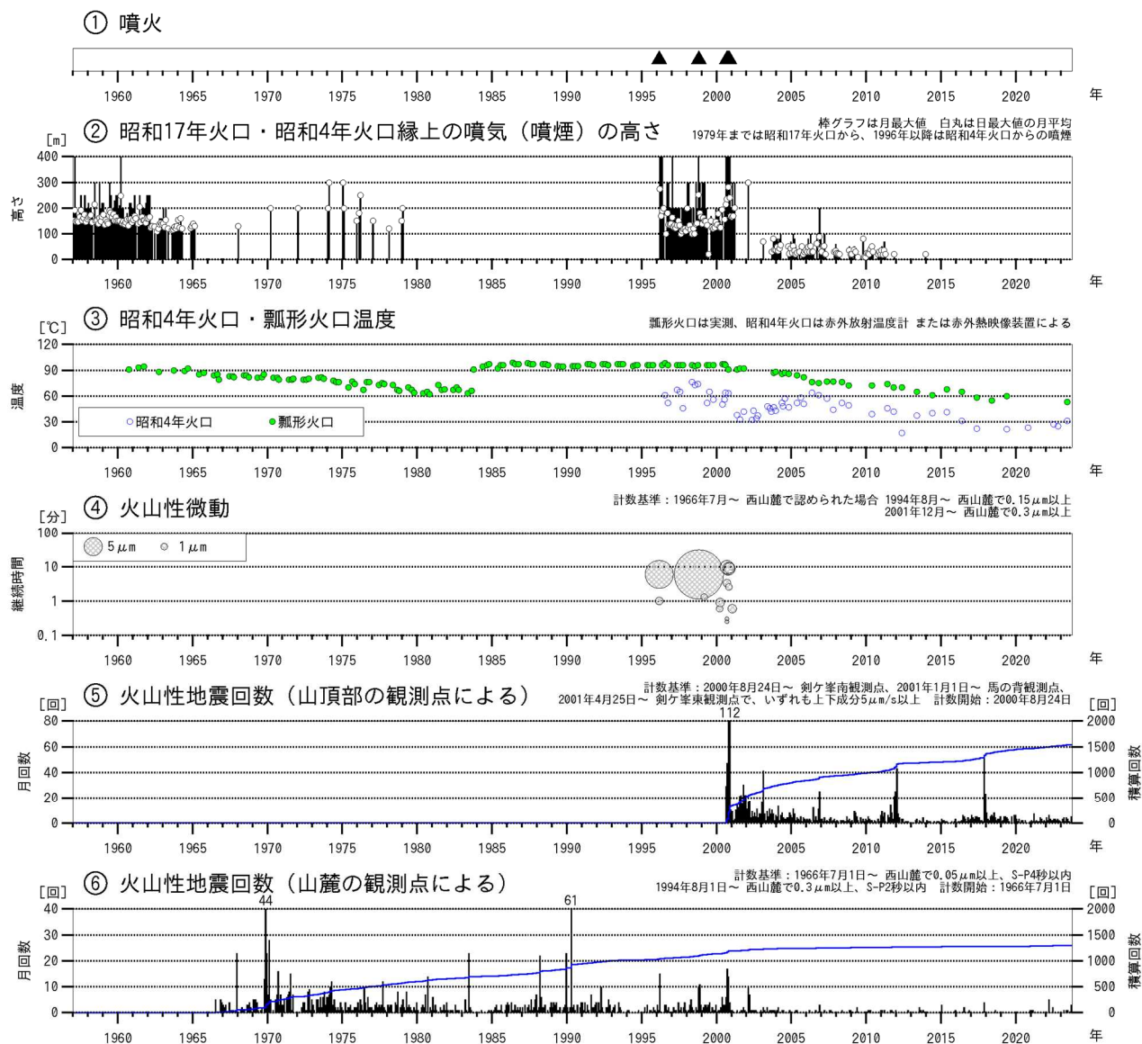
図1 北海道駒ヶ岳 火山活動経過図（1957年1月～2023年9月）
