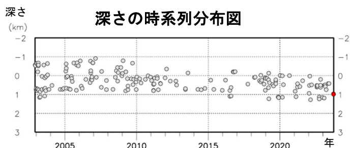
図4 北海道駒ヶ岳 火山性地震の震源分布（2002年12月～2023年9月） ●：2002年12月～2023年8月の震源 ●：2023年9月の震源 +：地震観測点
