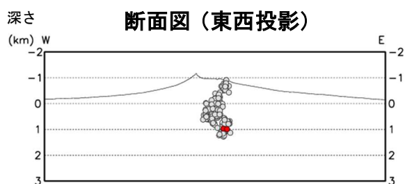
図4 北海道駒ヶ岳 火山性地震の震源分布（2002年12月～2023年9月） ●：2002年12月～2023年8月の震源 ●：2023年9月の震源 +：地震観測点
