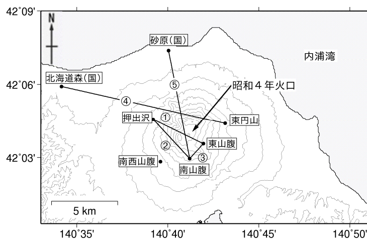
図5 北海道駒ヶ岳 GNSS連続観測による基線長変化（2001年4月～2023年9月）及び観測点配置図 グラフ①～⑤は観測点配置図の基線①～⑤に対応しています。 グラフの空白部分は欠測を示します。
