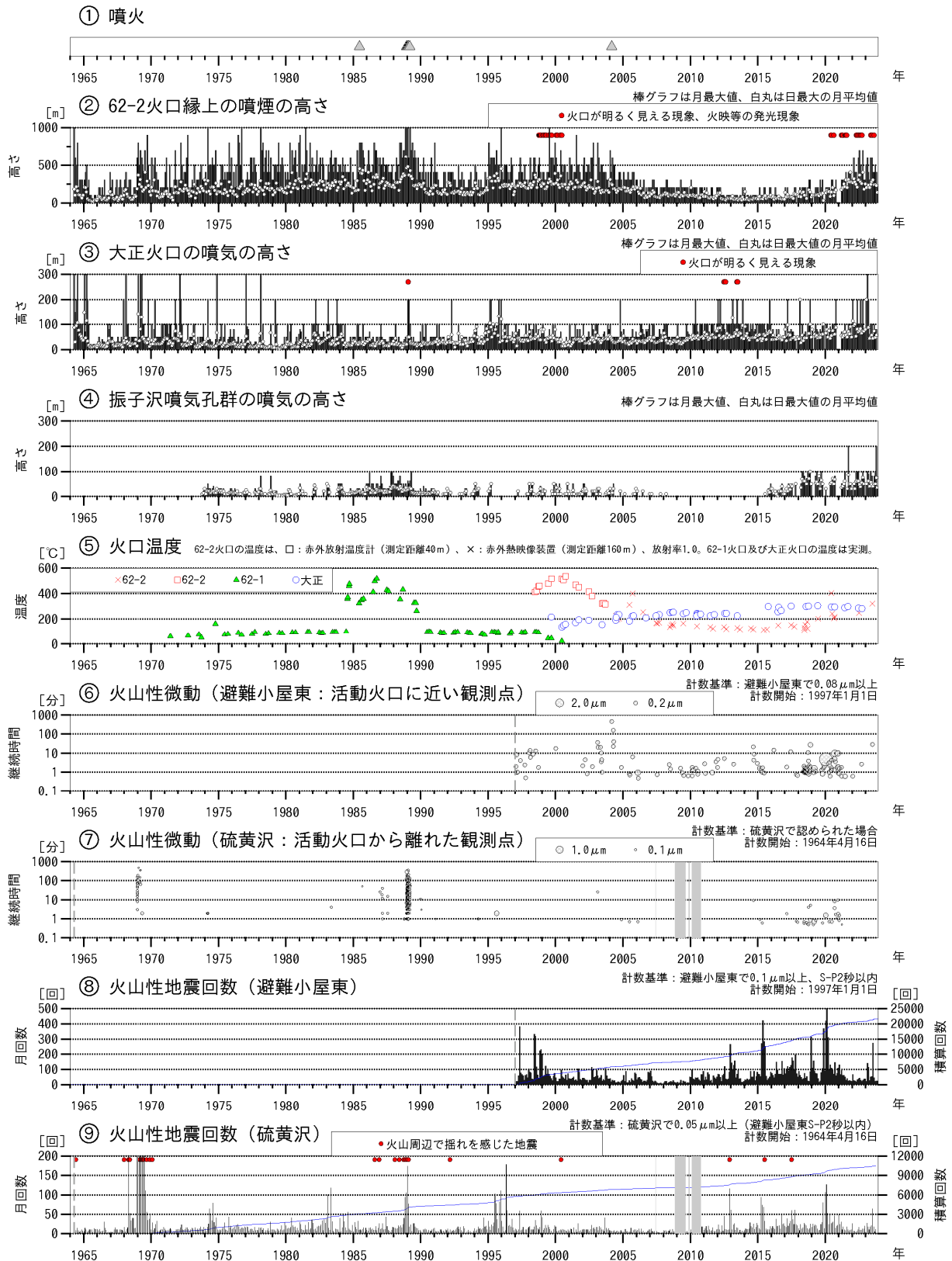
図1 十勝岳 火山活動経過図（1964年1月～2023年11月）
