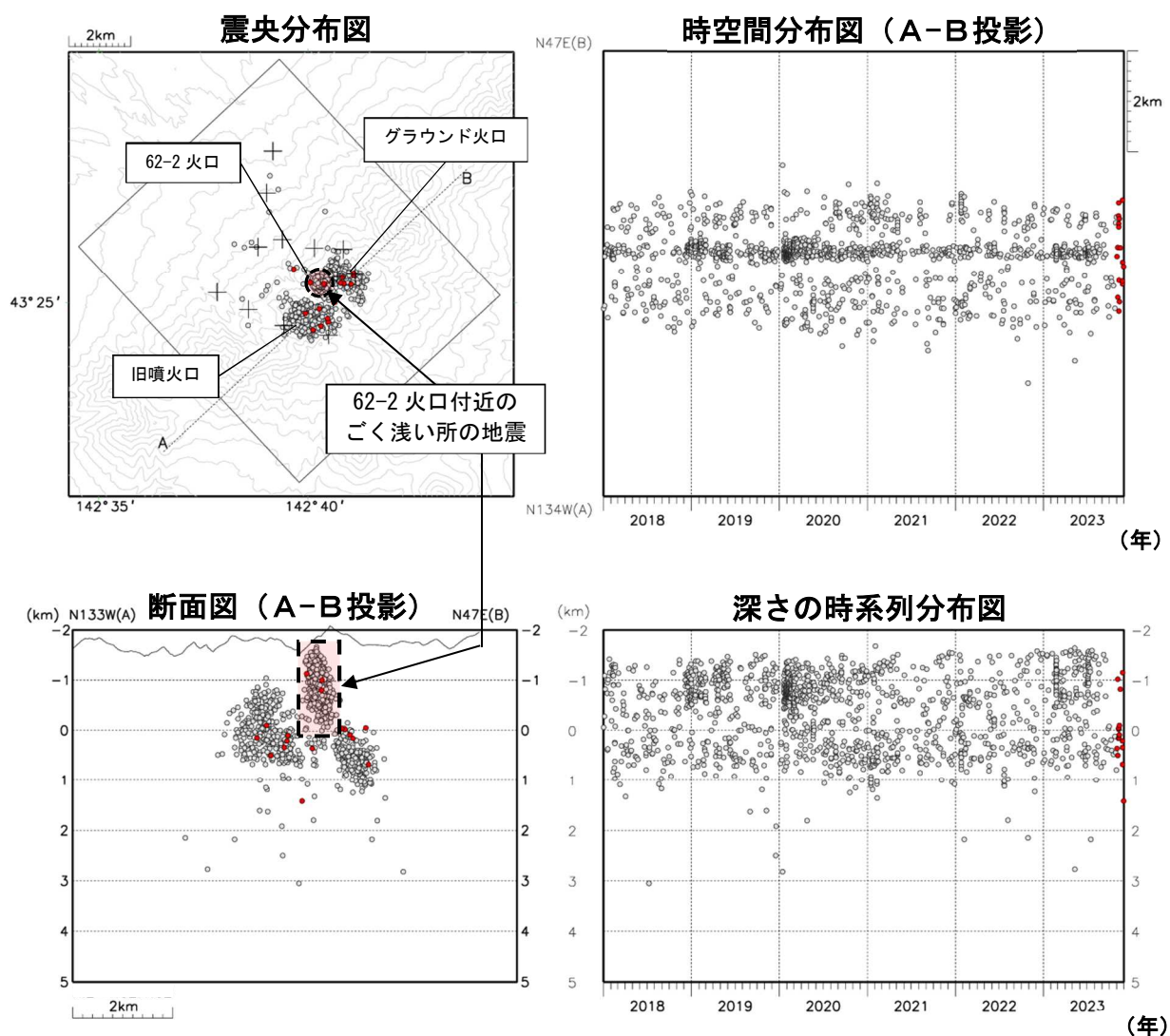
図4 十勝岳 火山性地震の震源分布（2018年1月～2023年11月）
