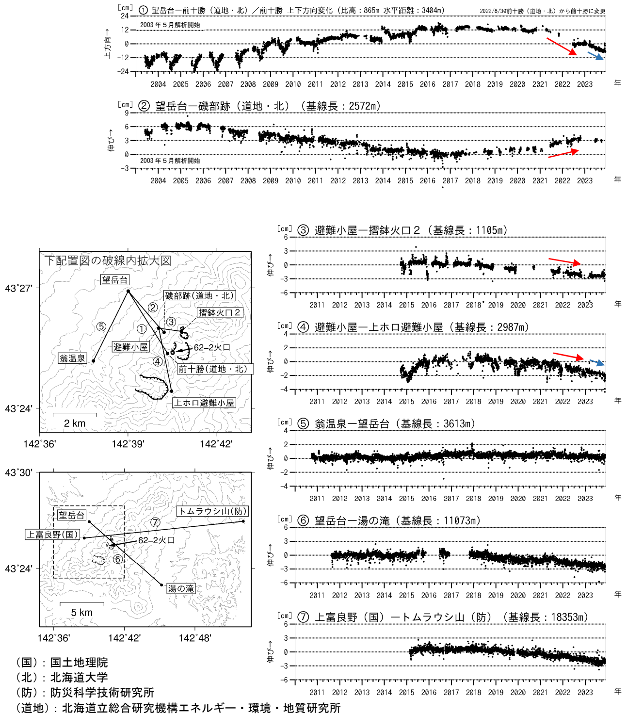
図5 十勝岳 GNSS連続観測による上下方向変化及び基線長変化（2003年5月～2023年11月）及び観測点配置図
