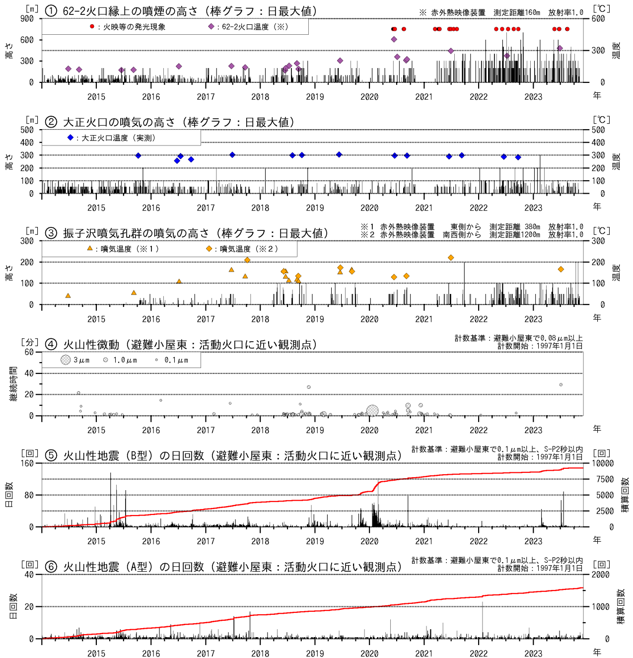
図2 十勝岳 火山活動経過図（2014年1月～2023年11月）
