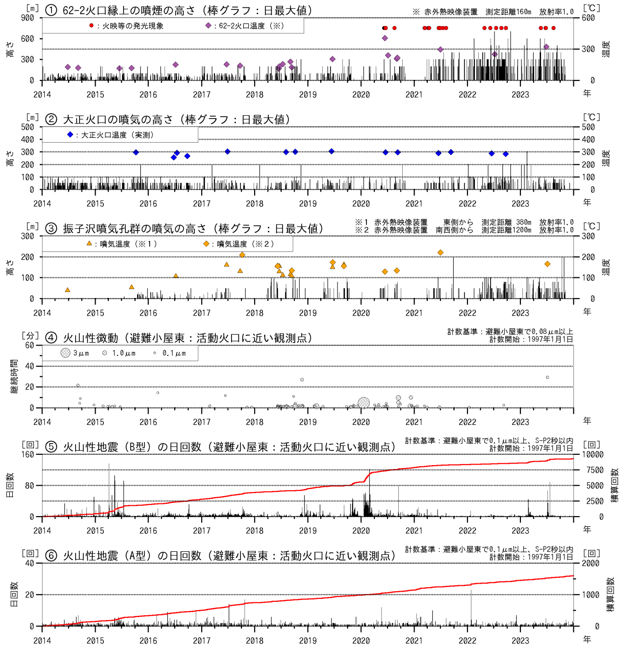
図2 十勝岳 火山活動経過図（2014年1月～2023年12月）
