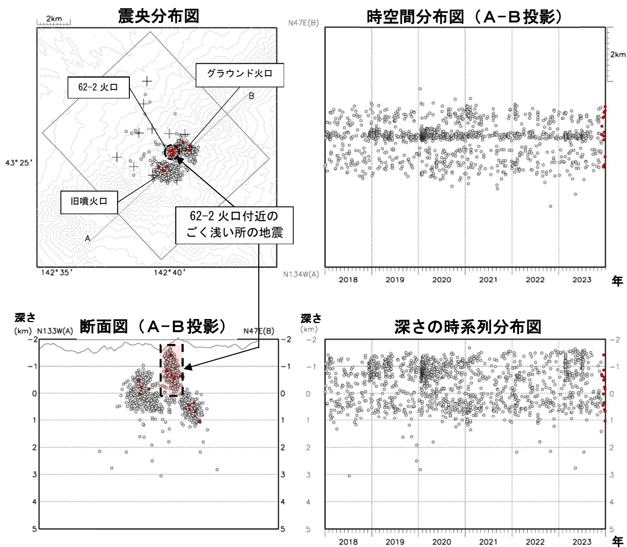
図4 十勝岳 火山性地震の震源分布（2018年1月～2023年12月）
