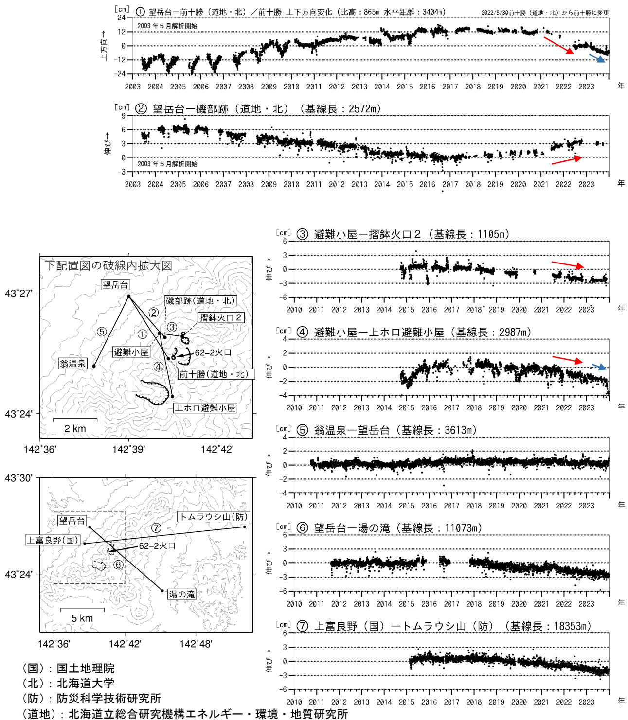
図5 十勝岳 GNSS連続観測による上下方向変化及び基線長変化（2003年5月～2023年12月）及び観測点配置図
