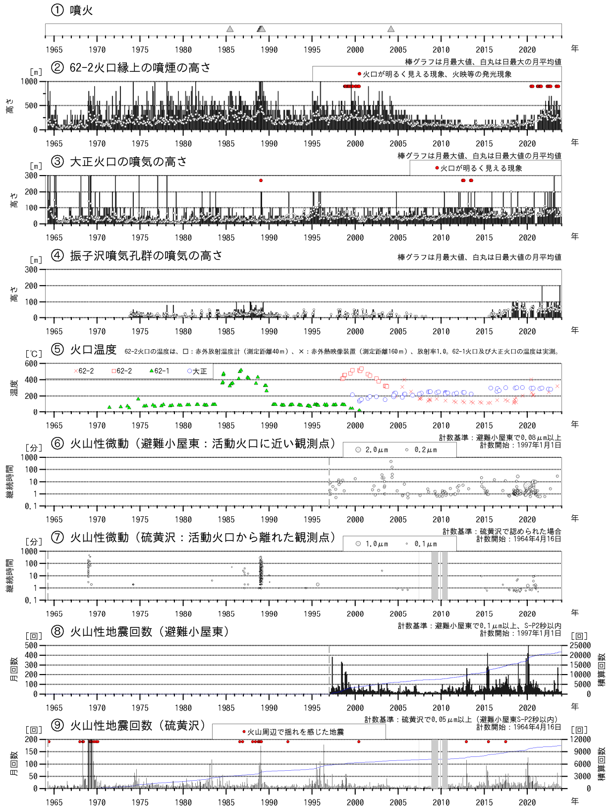
図1 十勝岳 火山活動経過図（1964年1月～2023年12月）
