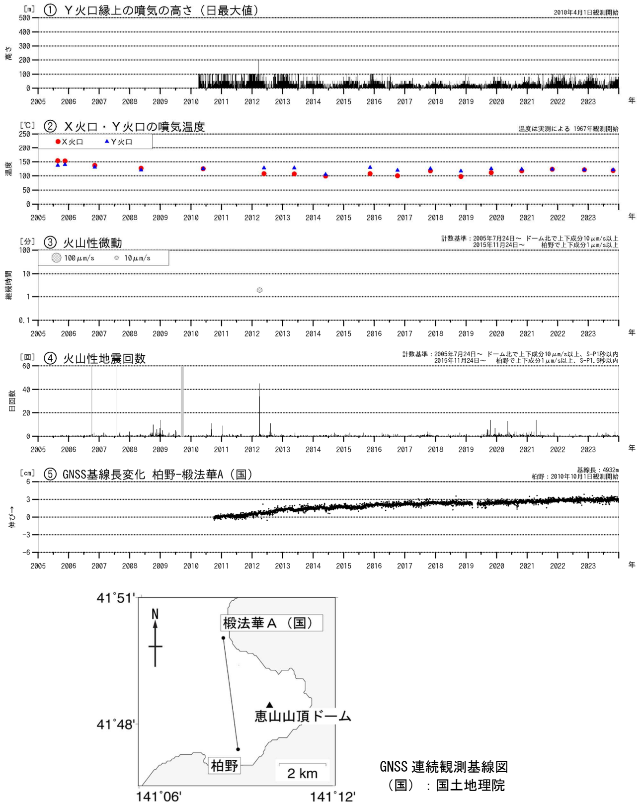
図2 恵山 火山活動経過図（2005年7月～2023年12月） ④の灰色部分は機器障害による欠測期間を示します。 ⑤のグラフは上図の基線に対応しています。 ⑤のグラフの空白部分は欠測を示します。
