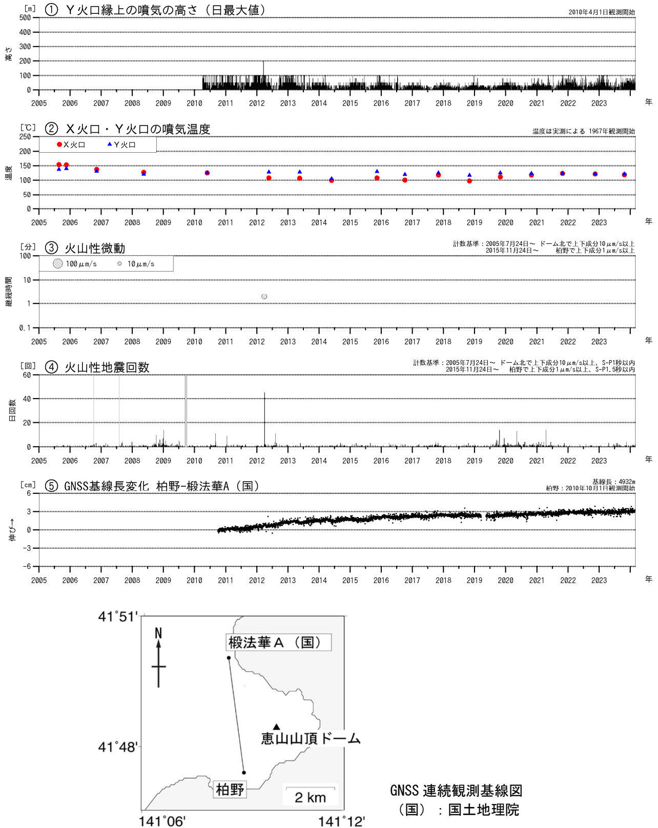
図2 恵山 火山活動経過図（2005年7月～2024年2月） ④の灰色部分は機器障害による欠測期間を示します。 ⑤のグラフは上図の基線に対応しています。 ⑤のグラフの空白部分は欠測を示します。
