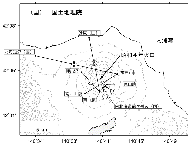
図6 北海道駒ヶ岳 GNSS連続観測による基線長変化（2001年4月～2024年4月）及び観測点配置図
