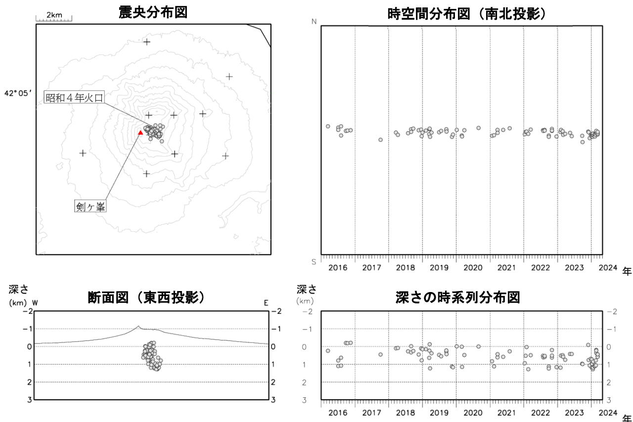
図4 北海道駒ヶ岳 火山性地震の震源分布（2016年1月～2024年4月）
