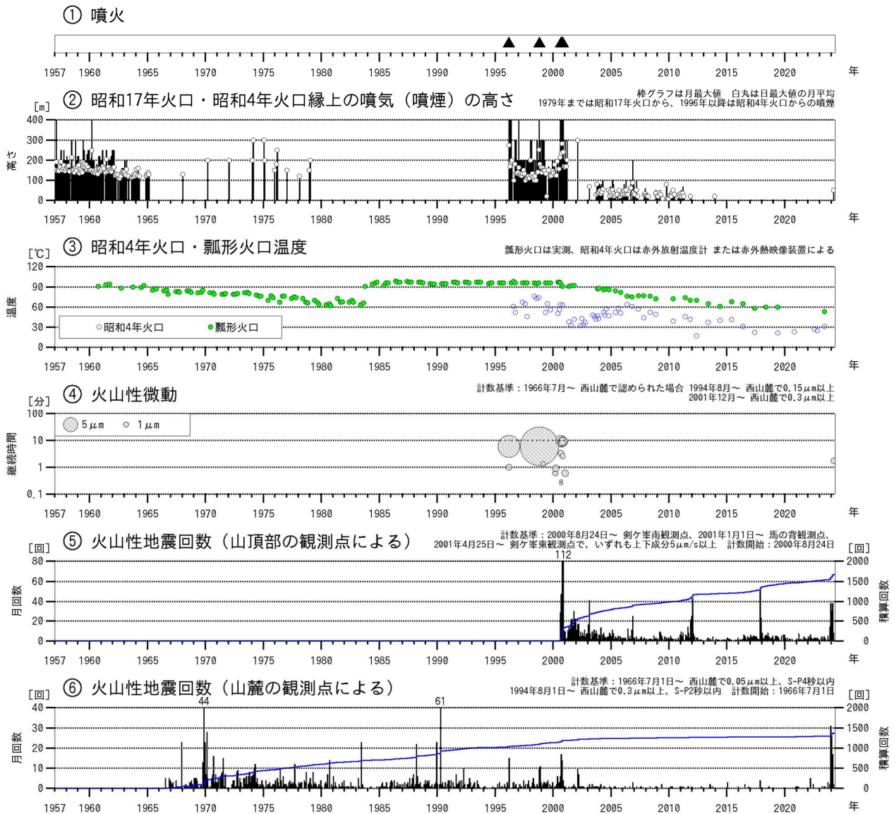
図1 北海道駒ヶ岳 火山活動経過図（1957年1月～2024年4月） 各火口の位置は図8を参照してください。
