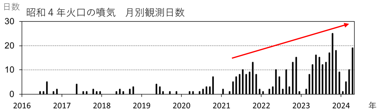
図2 北海道駒ヶ岳 昭和4年火口のごく弱い噴気を観測した日数（2016年1月～2024年4月） 山頂部に設置した剣ヶ峰監視カメラ及び駒ヶ岳山頂（道）監視カメラ（位置は図7～8参照）による観測結果です。 冬季は雪氷付着のため欠測日が多くなる傾向があります。
