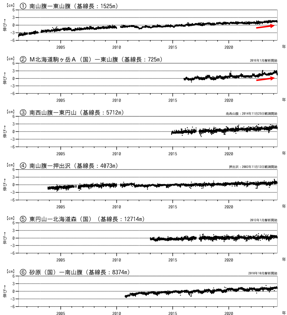
図6 北海道駒ヶ岳 GNSS連続観測による基線長変化（2001年4月～2024年4月）及び観測点配置図
