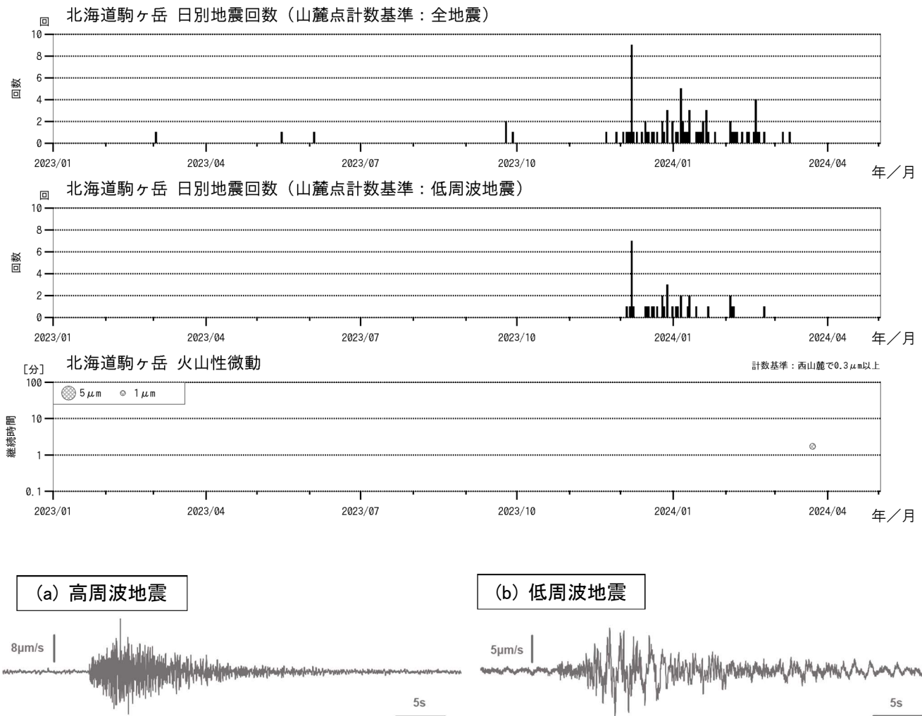
図5 北海道駒ヶ岳 日別地震回数と火山性微動の振幅、継続時間（上段：全地震 中段：低周波地震 下段：火山性微動 2023年1月～2024年4月）及び火山性地震の波形例（a：高周波地震 b：低周波地震）
