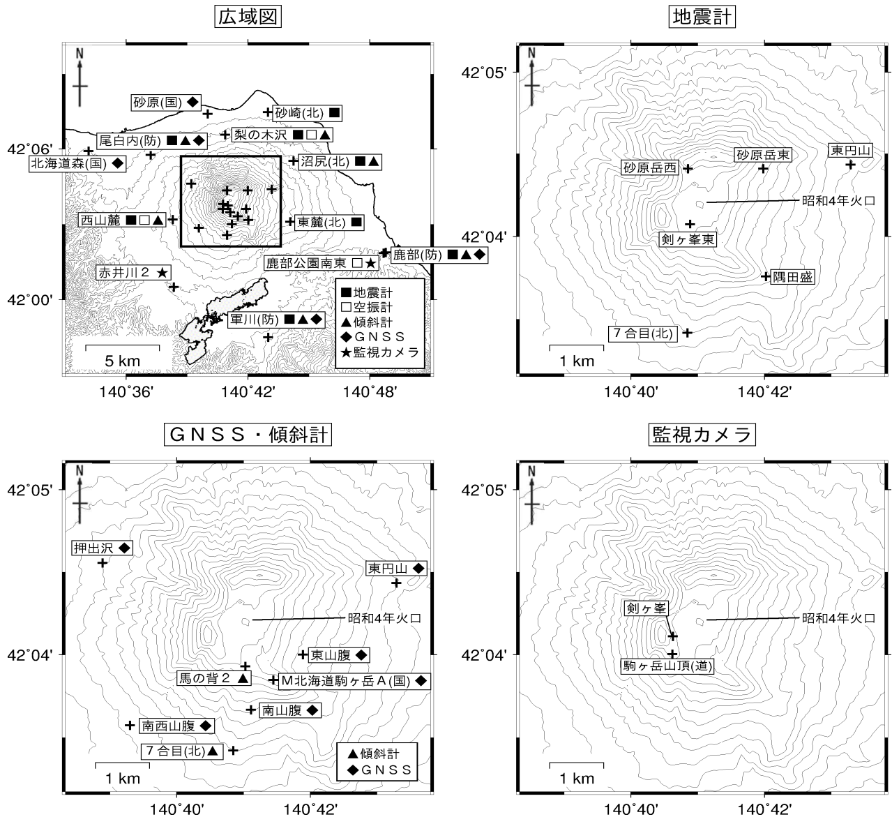
図7 北海道駒ヶ岳 観測点配置図
