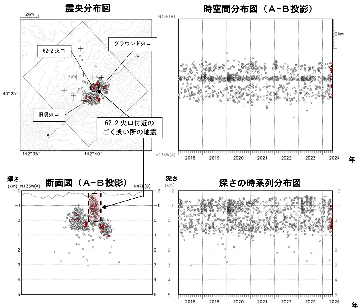
図4 十勝岳 火山性地震の震源分布（2018年1月～2024年5月）
