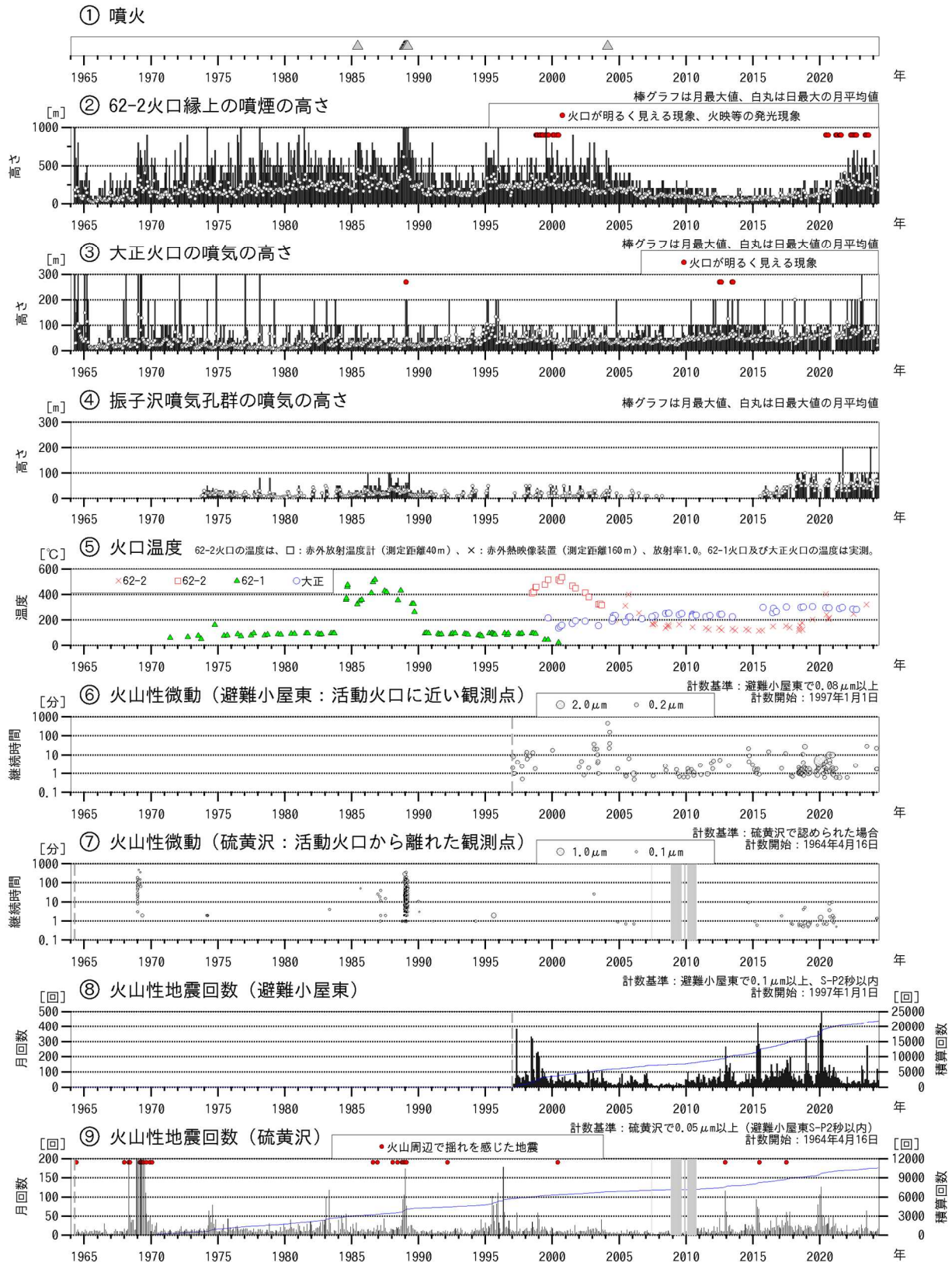
図1 十勝岳 火山活動経過図（1964年1月～2024年5月）
