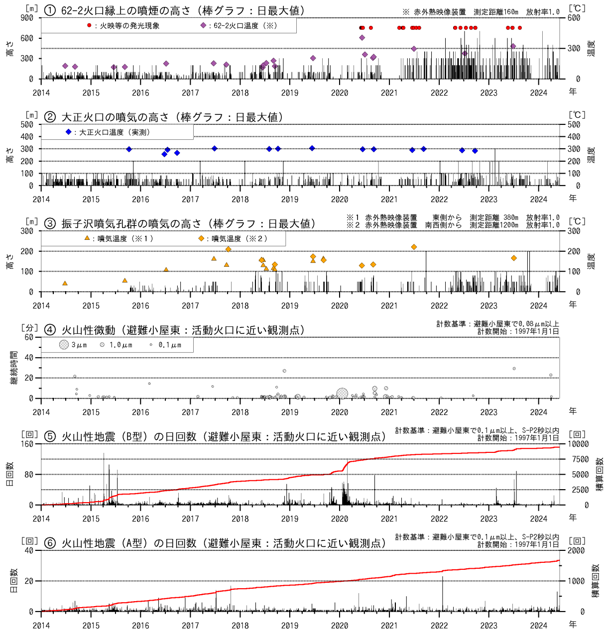
図2 十勝岳 火山活動経過図（2014年1月～2024年5月）
