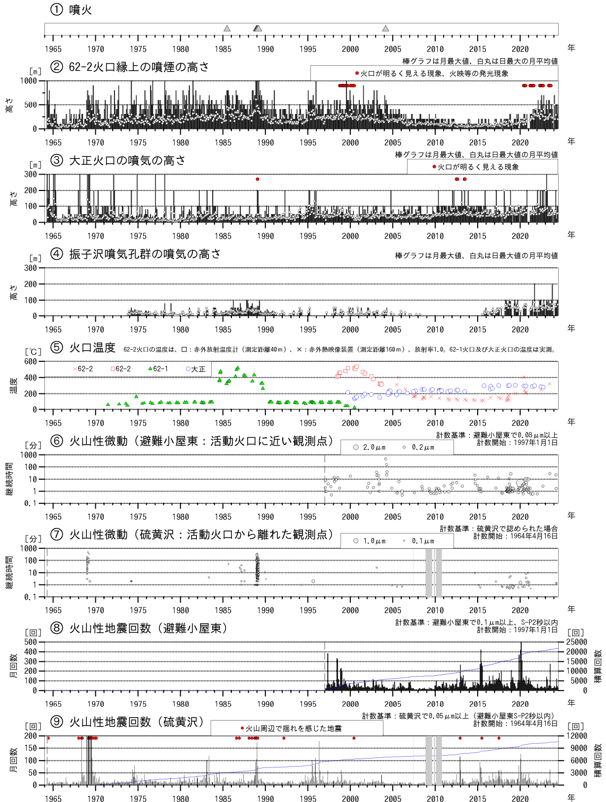
図1 十勝岳 火山活動経過図（1964年1月～2024年6月）
