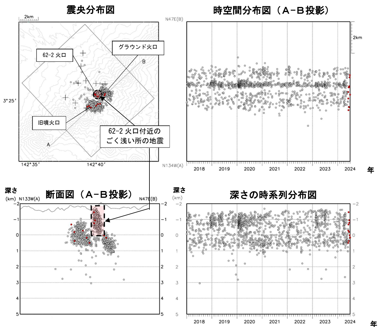
図4 十勝岳 火山性地震の震源分布（2018年1月～2024年6月） ●：2018年1月～2024年5月の震源 ●：2024年6月の震源 ＋：地震観測点
