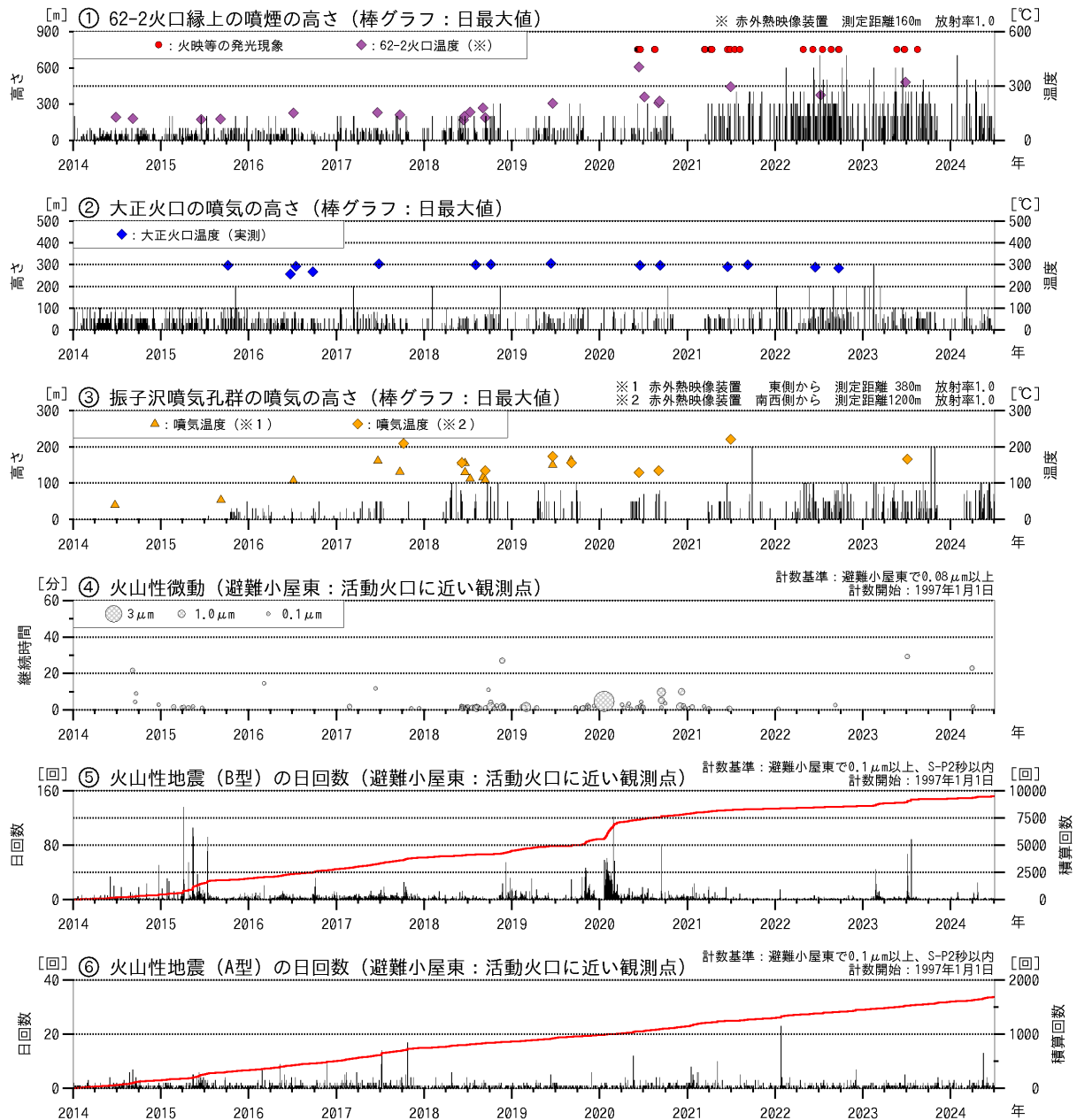
図2 十勝岳 火山活動経過図（2014年1月～2024年6月）
