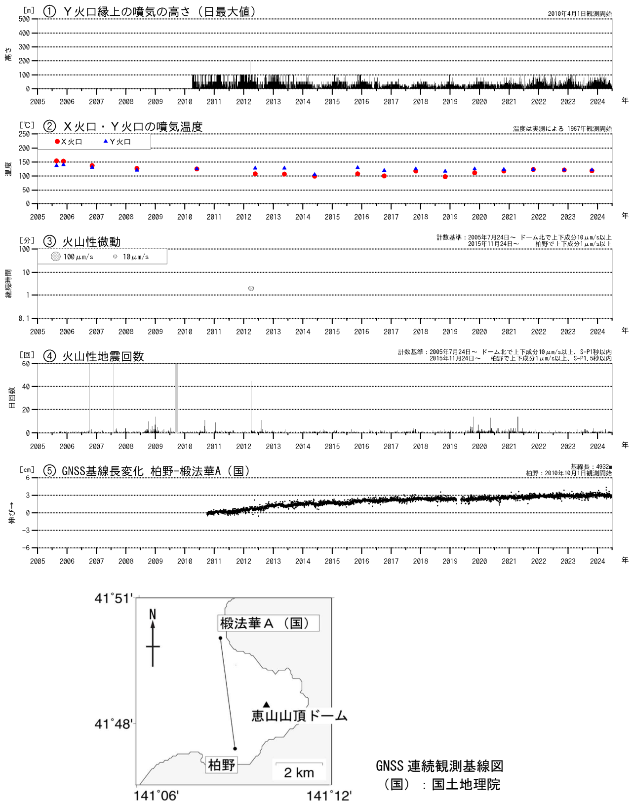
図2 恵山 火山活動経過図（2005年7月～2024年6月） ④の灰色部分は機器障害による欠測期間を示します。 ⑤のグラフは上図の基線に対応しています。 ⑤のグラフの空白部分は欠測を示します。
