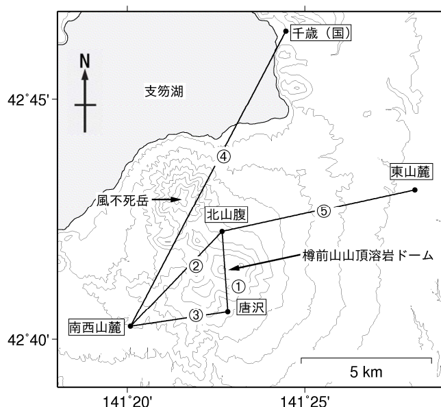
図4 樽前山 GNSS連続観測による基線長変化（2005年1月～2024年8月）及び観測点配置図 グラフ①～⑤は観測点配置図の基線①～⑤に対応しています。 グラフ中の空白部分は欠測を示しています。 ②～④の楕円内の変動（＊1）は2014年7月8日に発生した胆振地方中東部の地震によるものです。
