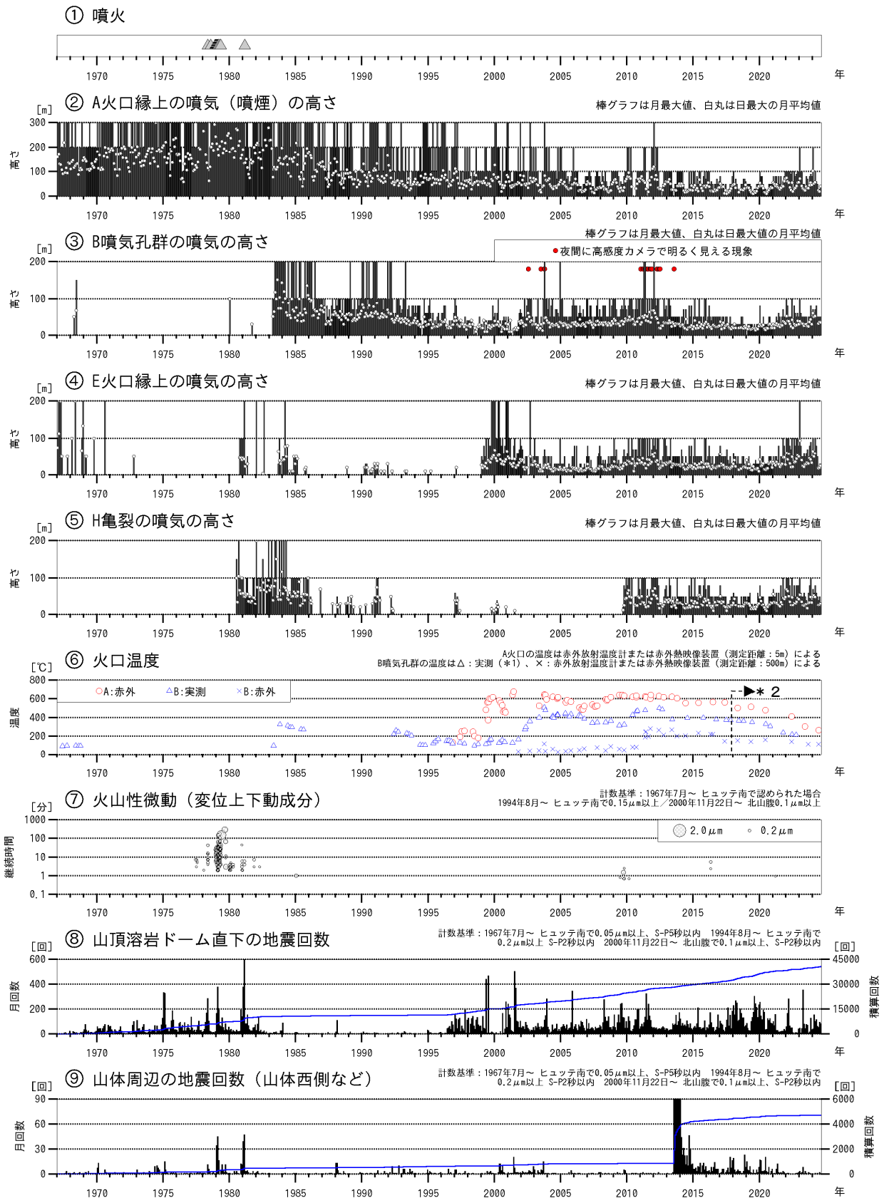
図2 樽前山 火山活動経過図（1967年1月～2024年8月）
