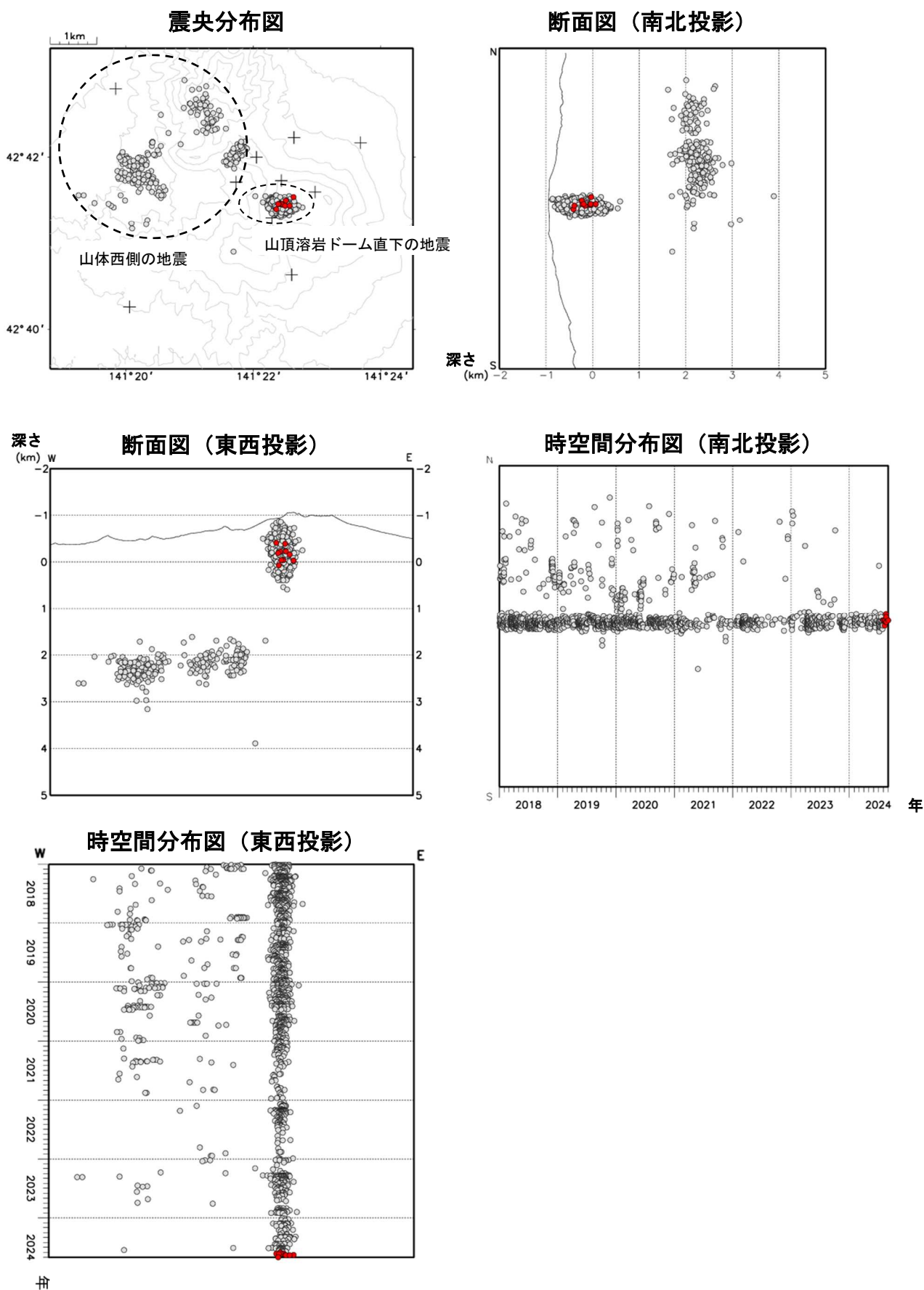
図3 樽前山 火山性地震の震源分布（2018年1月～2024年8月）
