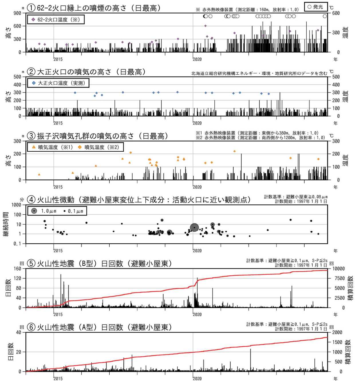
図2 十勝岳 火山活動経過図（2014年1月～2024年10月）
