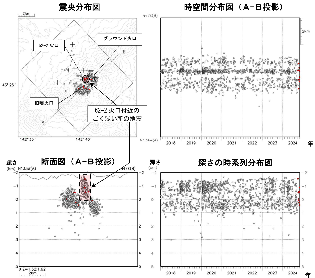
図4 十勝岳 火山性地震の震源分布（2018年1月～2024年10月）
