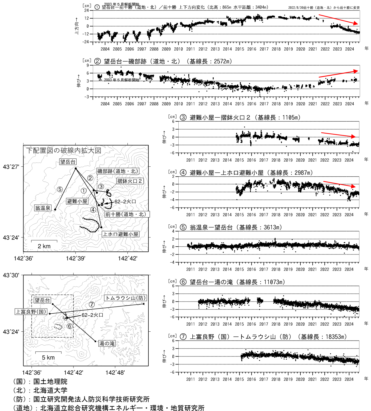
図5 十勝岳 GNSS連続観測による上下方向変化及び基線長変化（2003年5月～2024年10月）及び観測点配置図
