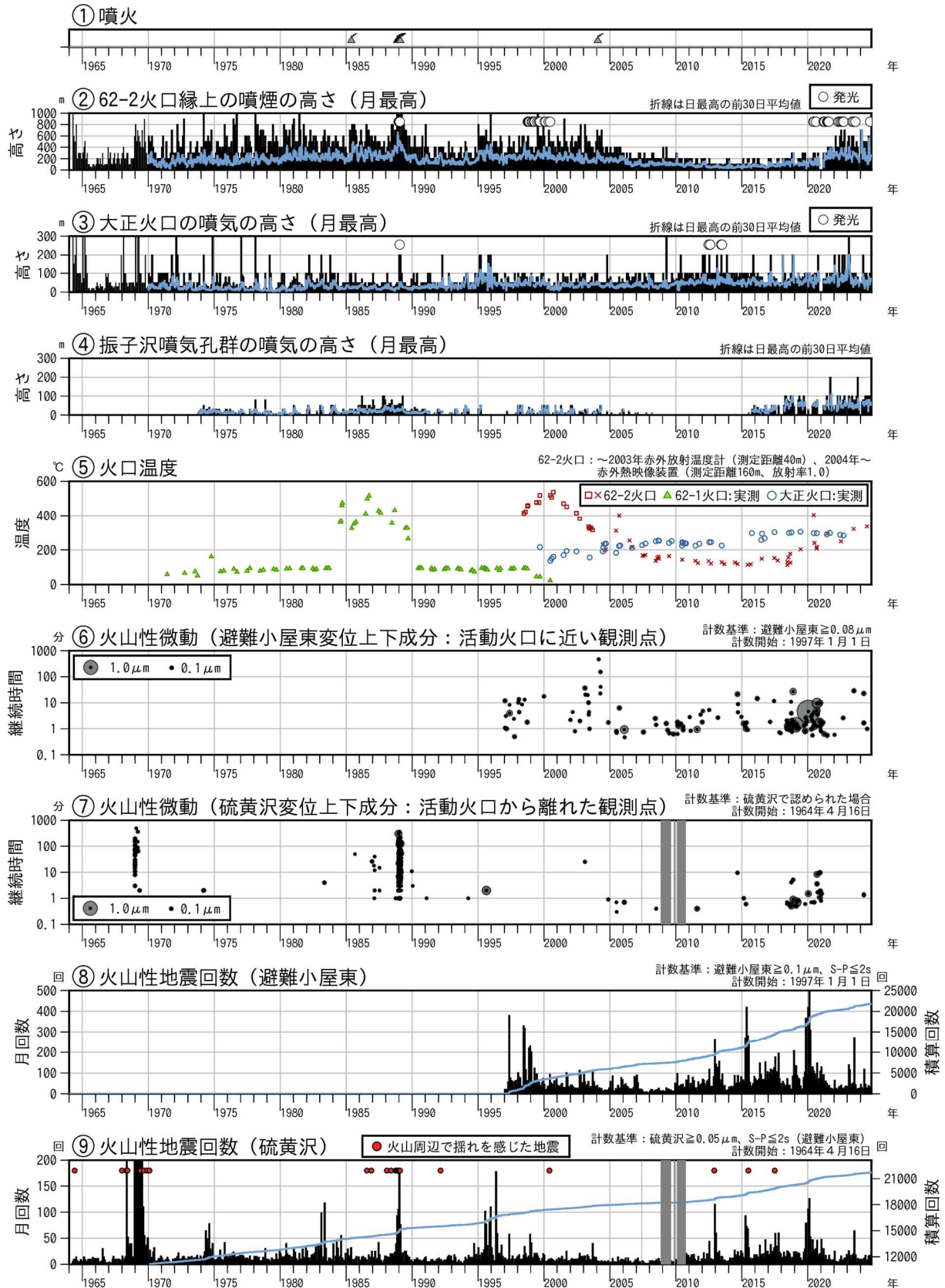
図1 十勝岳 火山活動経過図（1964年1月～2024年10月）
