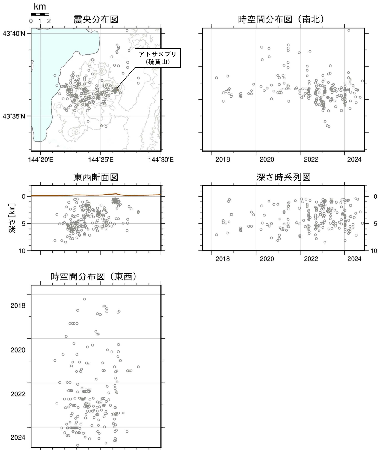
図3 アトサスプリ 火山性地震の震源分布（2017年8月～2024年11月）
