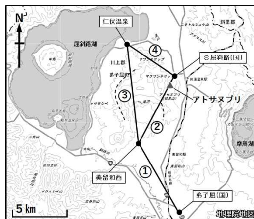
図4 アトサヌプリ GNSS連続観測による基線長変化（2010年10月～2024年11月）及び観測点配置図 冬季に凍上や積雪の影響によると考えられる変動がみられる基線があります。 ①の破線内の変動（* 1）は、弟子屈(国)付近の樹木の影響及び伐採によるものです。 グラフの空白部分は欠測を示します。 * 2 勝井義雄（1958）阿寒・屈斜路火山群、地球科学、39巻。
