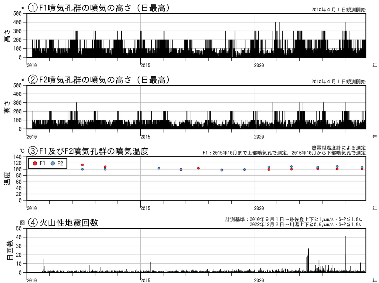
図1 アトサヌプリ 火山活動経過図（2010年4月～2024年11月）
