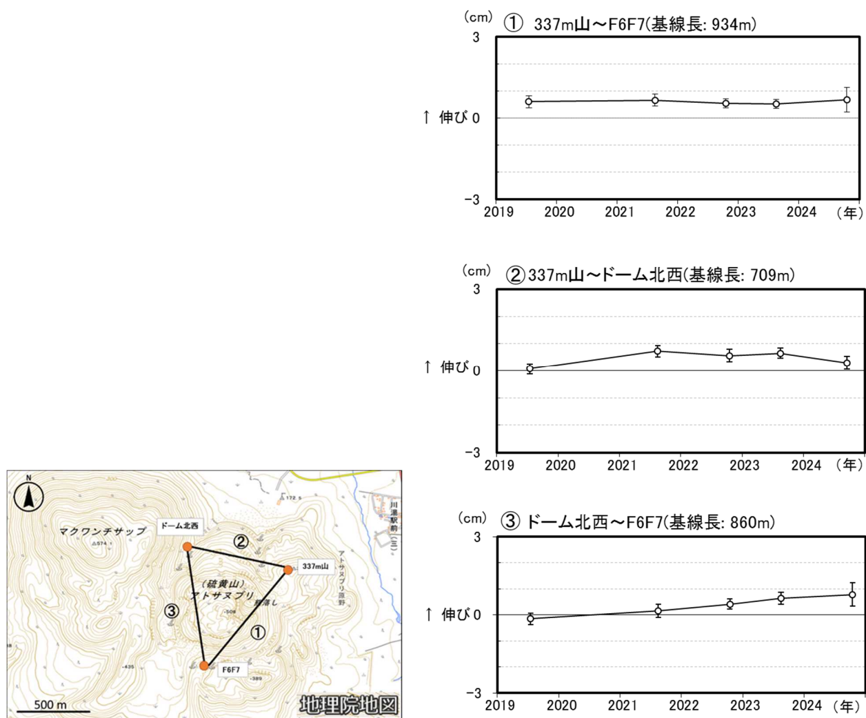
図5 アトサヌプリ GNSS繰り返し観測による基線長変化及び観測点配置図（2019年7月～2024年10月）と基線組み合わせ
